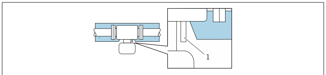
36 Isolamento térmico com pescoço estendido livre e célula de medição de pressão
