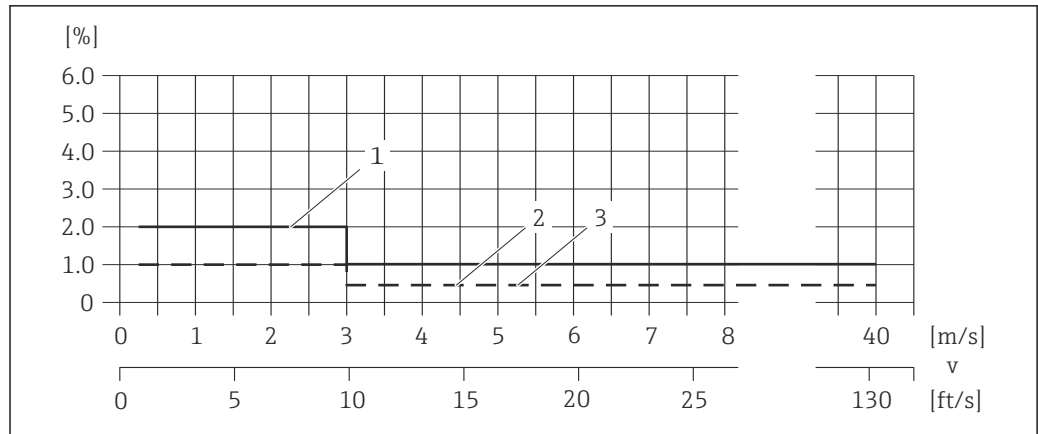
35 Erro máximo de medição (fluxo de volume) em % da leitura
