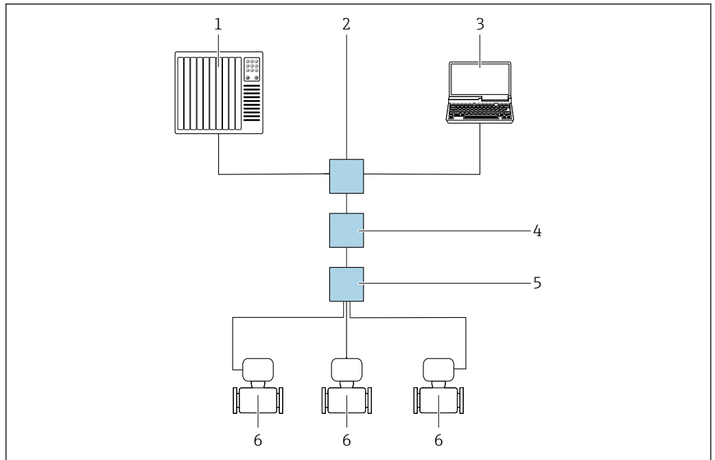
図 31 APL ネットワーク経由のリモート操作用オプション
