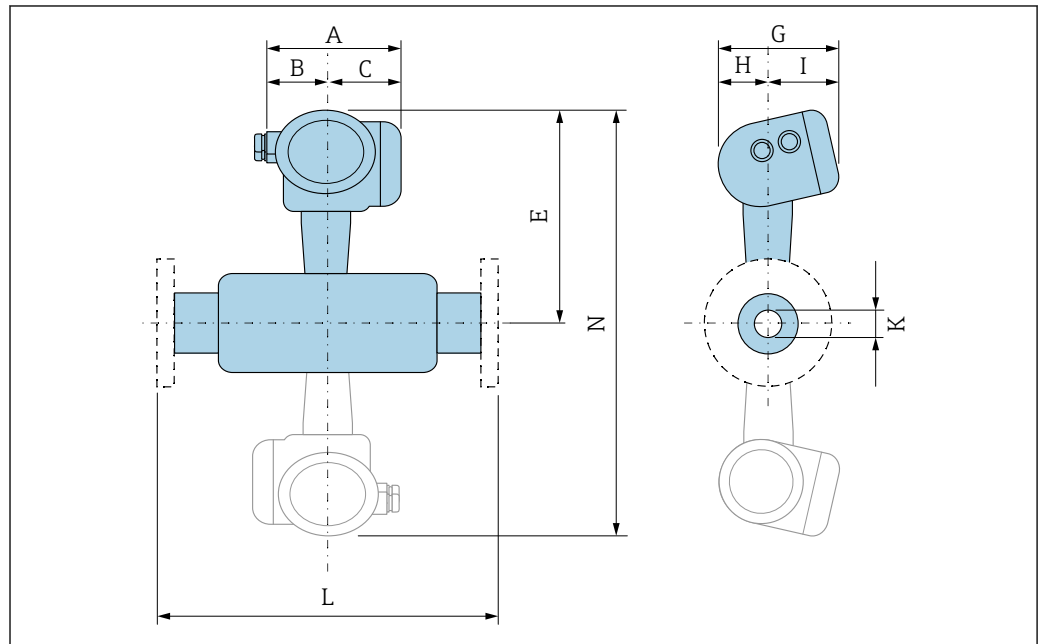
図 22 灰色表示：デュアルセンサタイプ
