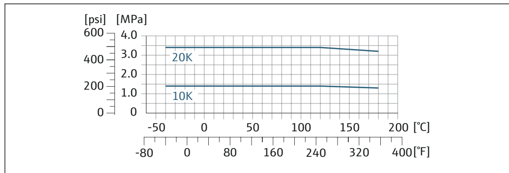
図 20 フランジ接続材質 : ステンレス、複数の認証、1.4404/SUS F316 または F316L 相当
