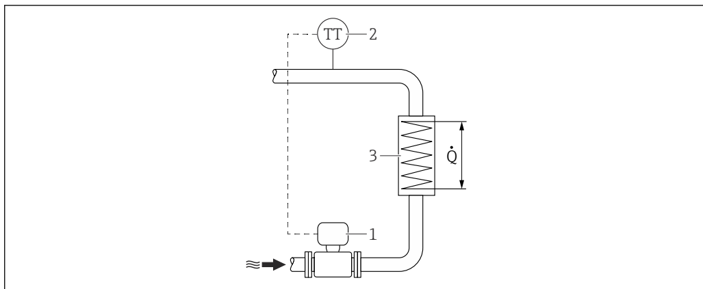
図 17 飽和蒸気/水の差エネルギー計測
