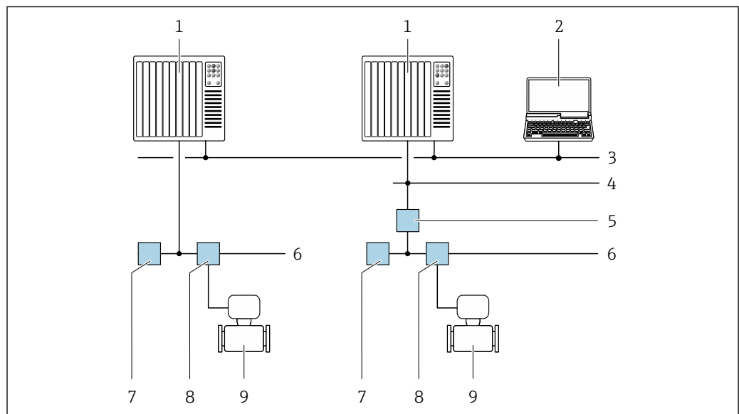
図 30 FOUNDATION フィールドバスネットワークを介したリモート操作のオプション
