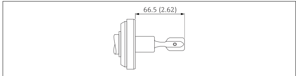
25 Соединительный штуцер DIN11864-1. Единица измерения мм (дюйм)
