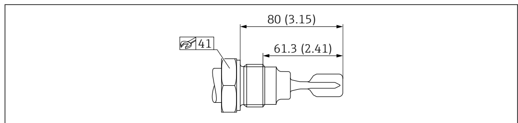
21 Резьба ISO 228 G 1. Единица измерения мм (дюйм)
