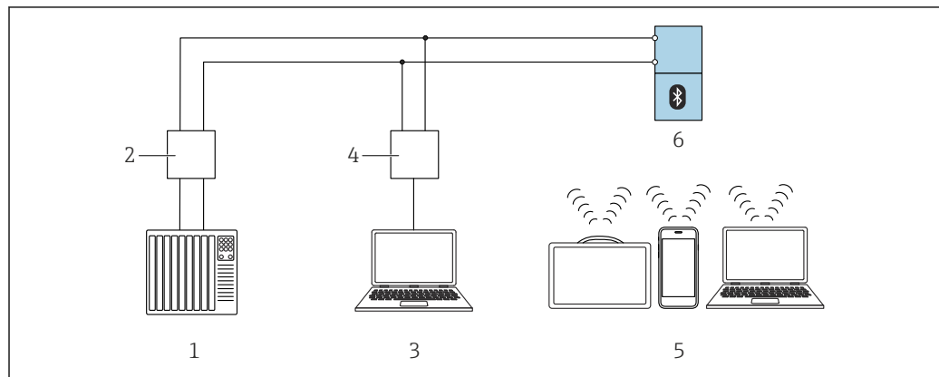
33 Варианты дистанционного управления по протоколу IO-Link
