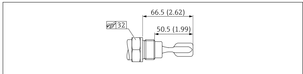
图 20 ISO228 G 3/4 螺纹。测量单位 mm (in)
