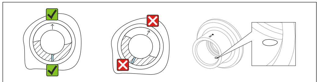
图 13 焊座，带泄漏检测孔
