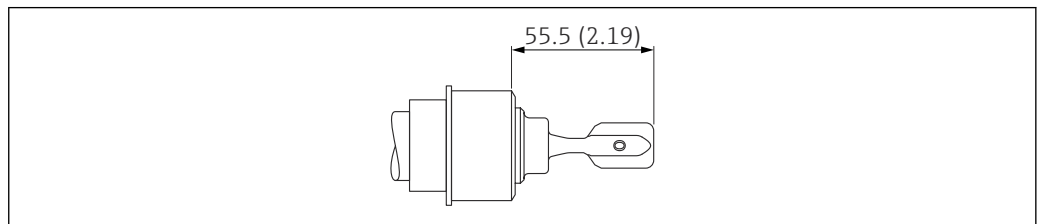
☒ 23 罐体接头 (齐平安装在焊座中)。测量单位 mm (in)
