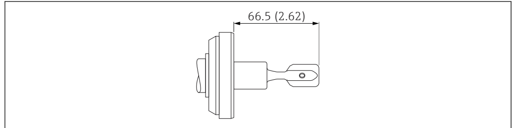
图 25 DIN11864-1 管接头。测量单位 mm (in)
