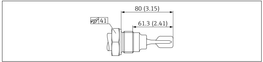
☒ 21 ISO228 G1 螺纹。测量单位 mm (in)
