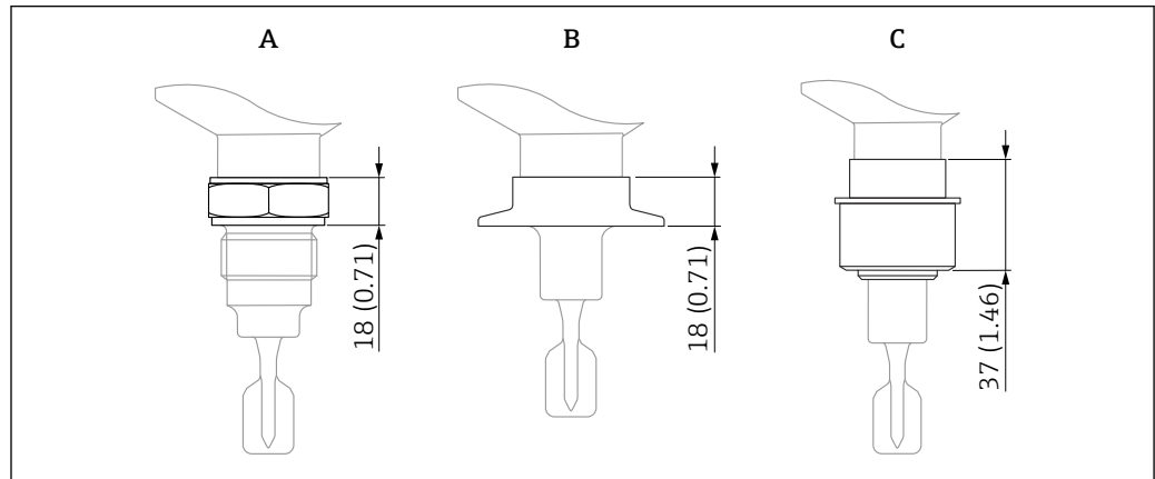
图 19 过程连接的最大高度规格。测量单位 mm (in)
