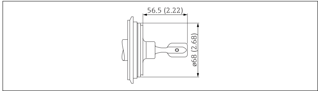
图 29 Varivent N 型接头，DN65-162 PN25 配合管道。测量单位 mm (in)
