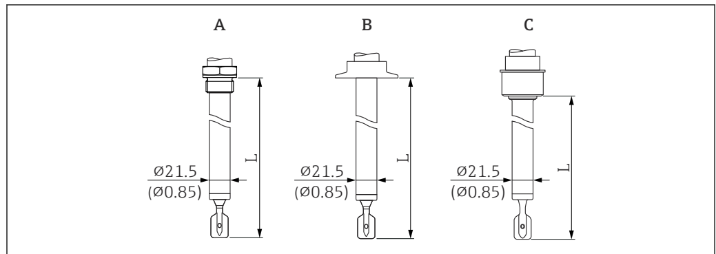
17 探头类型：延长管型、短管型（传感器长度 L）。测量单位 mm (in)
