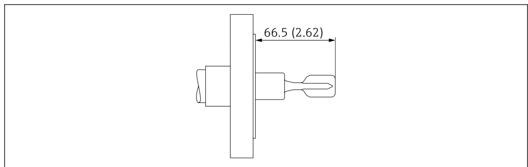
图 32 法兰连接型传感器示意图。测量单位 mm (in)
