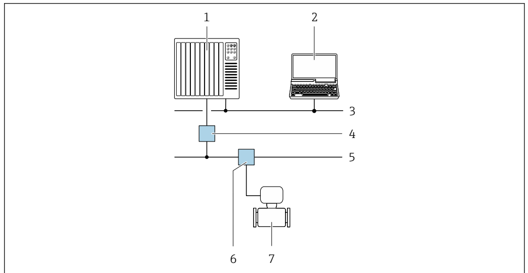
28 Opções para operação remota através da rede PROFIBUS PA
