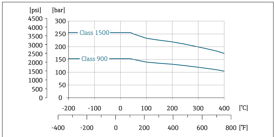
19 Material de conexão do flange: aço inoxidável, várias certificações, 1.4404 / F316 / F316L
