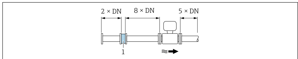
1 流量调节器
