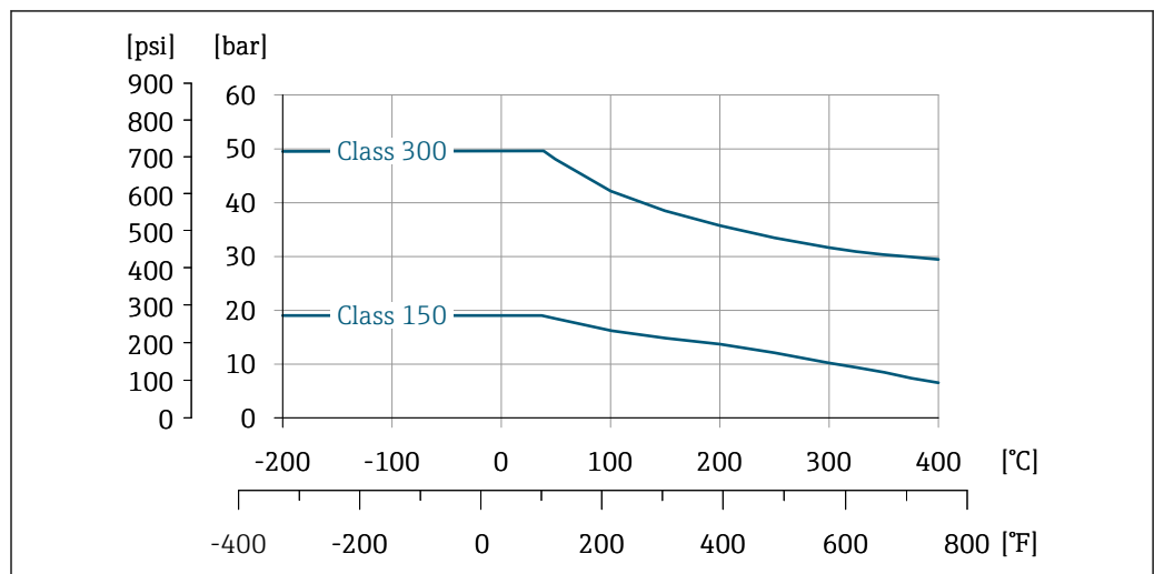
19 Material de la conexión bridada: acero inoxidable, múltiples certificaciones, 1.4404/F316/F316L
