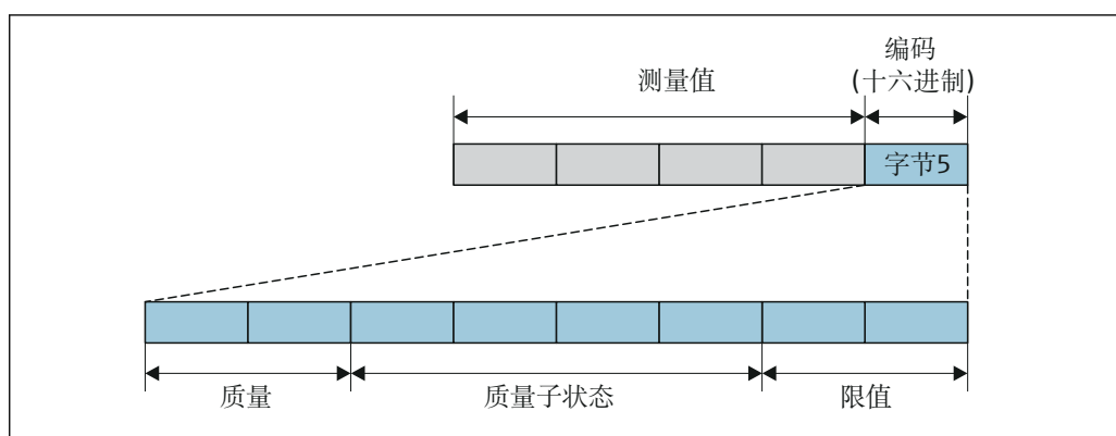
图 21 状态字节结构
