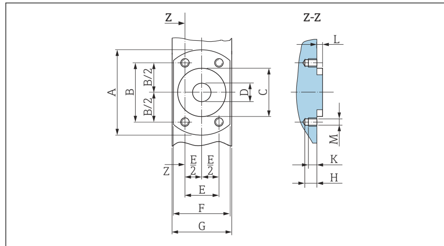
7 Вид спереди без присоединений к процессу
