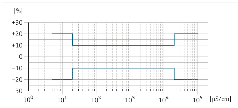
5 Погрешность измерения для кода заказа "Измерение электропроводности", опция CX
