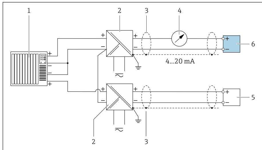
图 2 接线示例, HART 输入, 公共端接负极 (无源信号)
