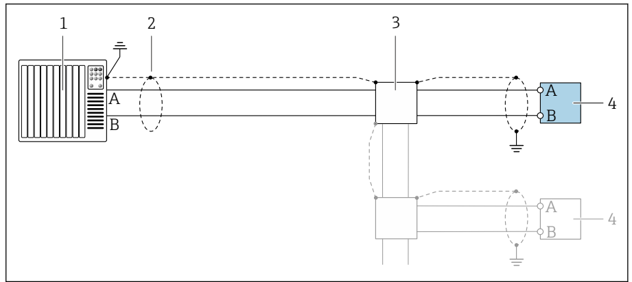
4 接线示例，Modbus RS485，非防爆区和防爆区（Zone 2；Cl. I, Div. 2）
