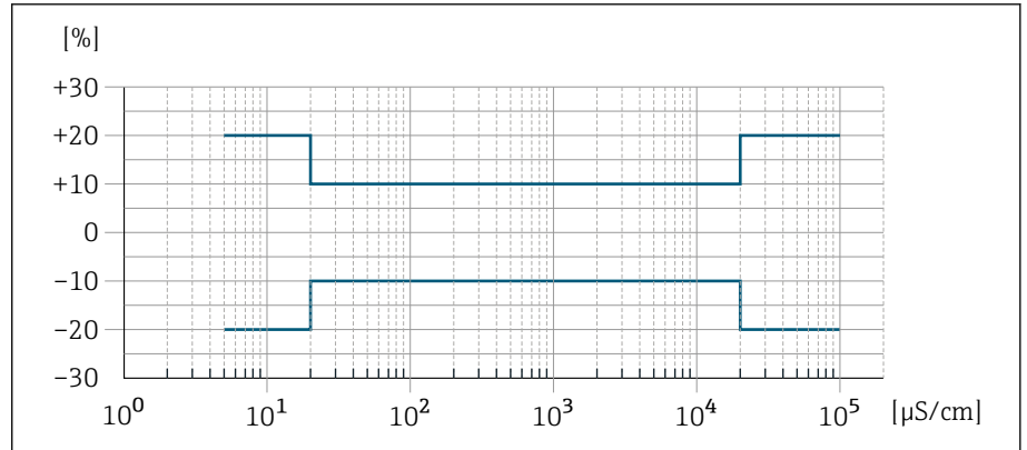
图 5 测量误差 (订购选项“电导率测量”, 选型代号 CX)
