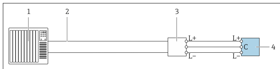
图 3 IO-Link 通信连接实例 (仅针对非防爆危险区)
