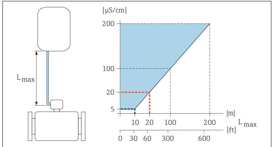
图 6 允许连接电缆长度
