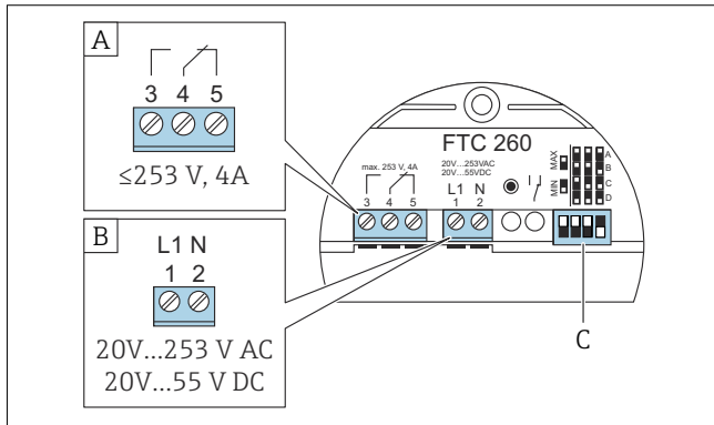
图 3 带交流或直流供电接口和继电器输出的设备
