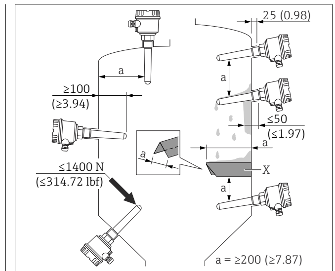
图 1 在料仓中安装设备需满足的最小间距要求，单位：mm (in)；x：防护罩
