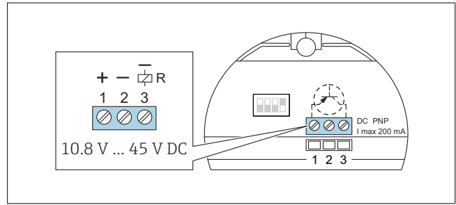
图 4 带直流供电接口的设备
