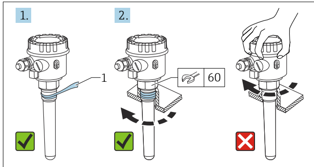
图 2 拧入设备
