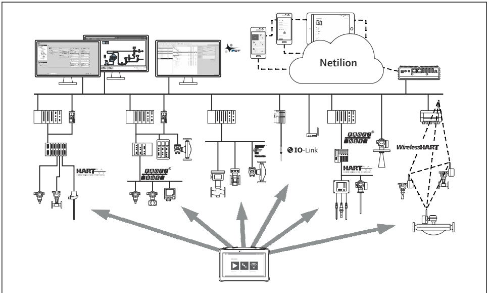
图 3 网络架构
