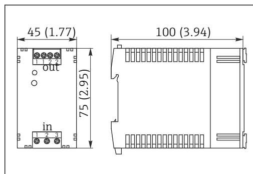
35 Alimentation 24 V
