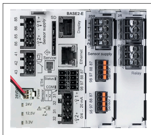
12 CM444R : exemple
