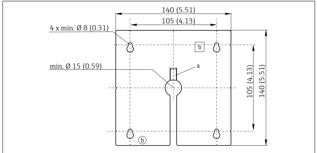
33 Plaque de montage de l'afficheur externe, dimensions en mm (in)
