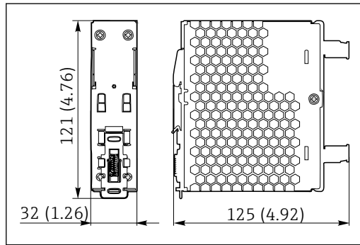
37 Alimentation 230 V
