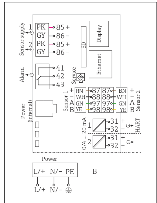
15 Schéma de raccordement complet, exemple du BASE2-E et de l'alimentation externe (B)
