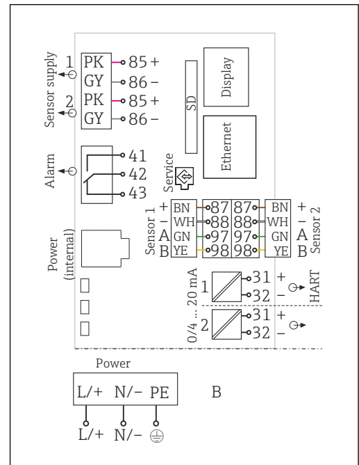
13 Schéma de raccordement complet, exemple du BASE2-E et de l'extension d'alimentation (B)
