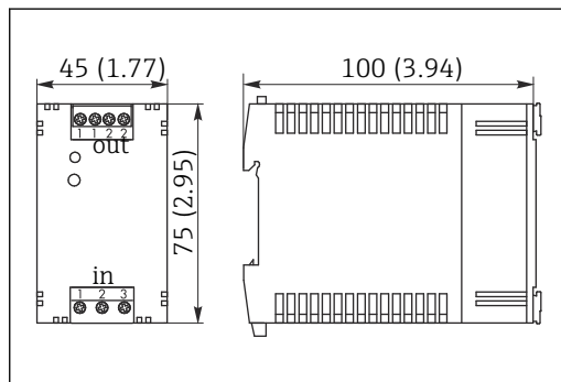
39 Alimentation 24 V
