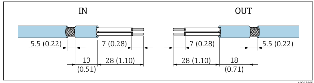
10 Empfohlene Abmessungen für die Abisolierung bei Kabelverschraubungen für geschirmtes Kabel für die Eingangsklemme IN und die Ausgangsklemme OUT
