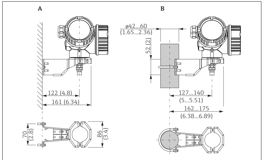
40 Монтажный кронштейн для корпуса электроники, единицы измерения: мм (дюймы)
