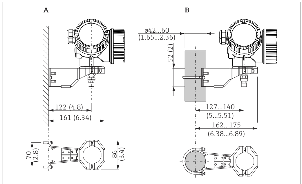
6 Монтаж корпуса блока электроники на монтажном кронштейне. Единица измерения мм (дюйм)
