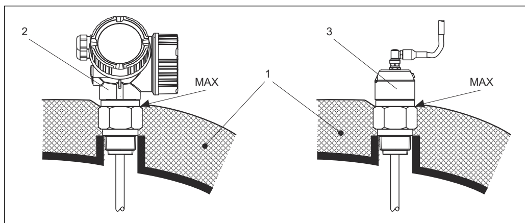
5 Технологическое соединение с резьбой
