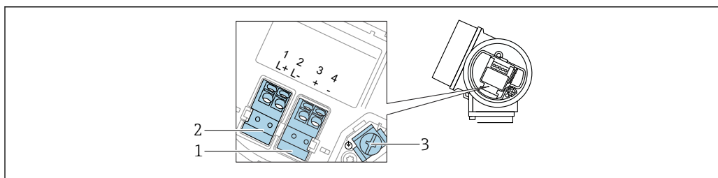
16 Назначение клемм, 4-проводное подключение: 4 до 20 мА HART (10,4 до 48 V DC )
