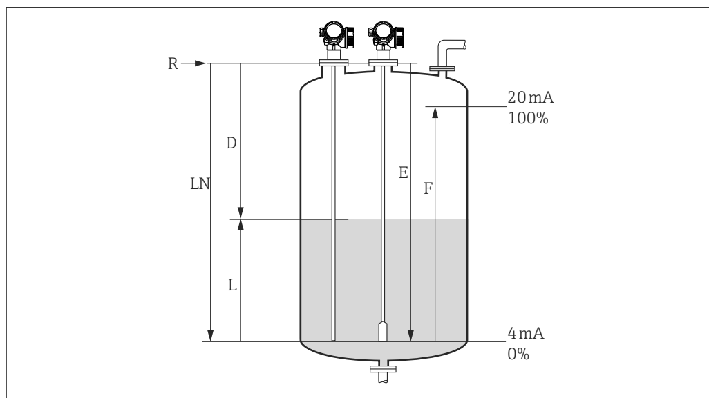
33 Параметры конфигурации для измерения уровня жидкости
