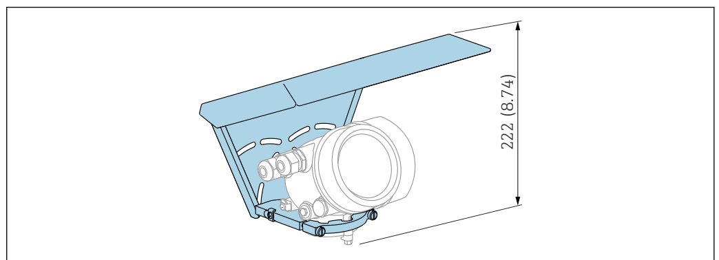
38 Высота. Единица измерения мм (дюйм)
