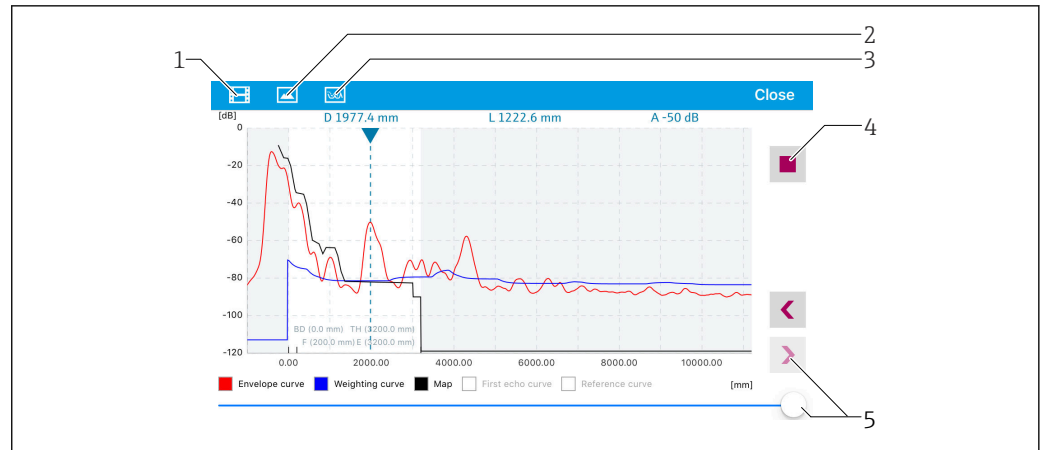
31 Отображение огибающей кривой (пример) в приложении SmartBlue; устройство iOS
