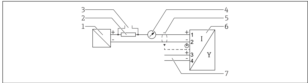
図 11 機能図：4~20 mA HART、スイッチ出力
