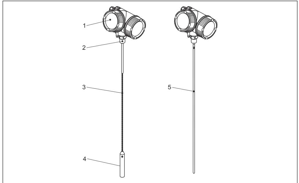
図 1 Levelflex の構造
