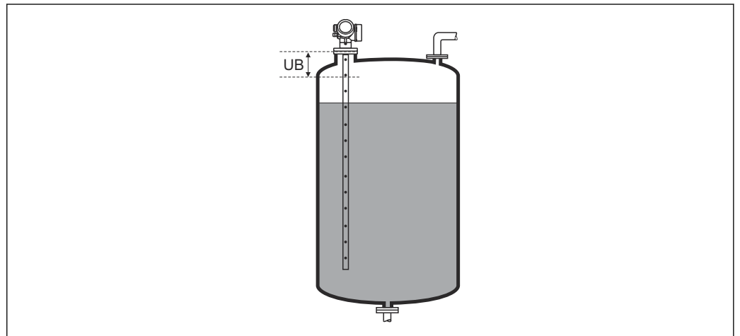
50 液体計測の不感知距離 (UB)
