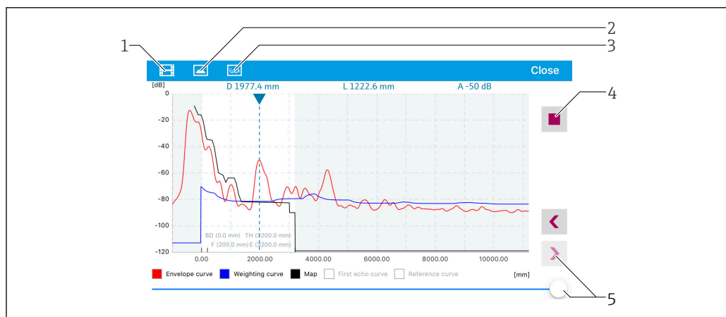
図 31 SmartBlue (iOS 版) での反射波形表示 (例)
