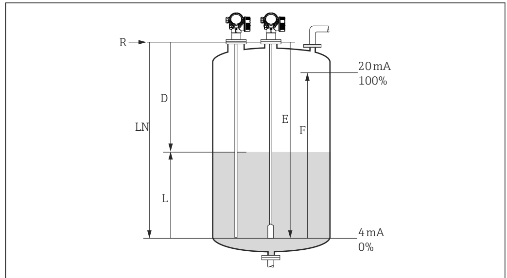
図 33 液体のレベル測定用パラメータの設定
