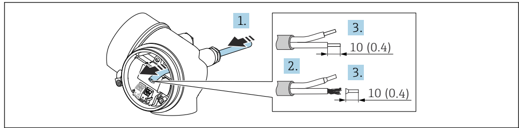
図 22 単位 : mm (in)
