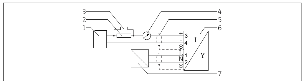
図 19 機能図、4 線式：4~20 mA HART (90~253 V AC )
