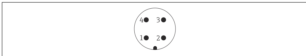
図 20 M12 プラグのピン割当て
