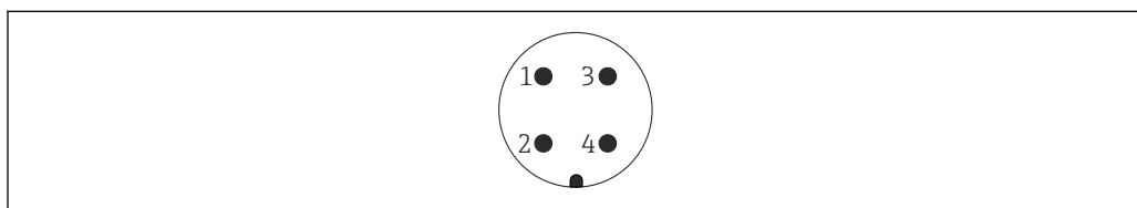
図 21 7/8" プラグのピン割当て
