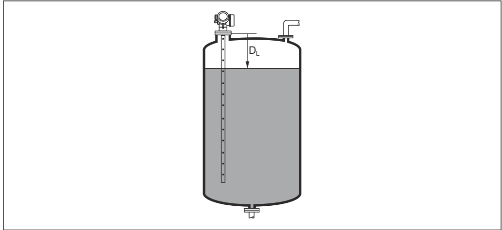
図 46 液体計測の距離
