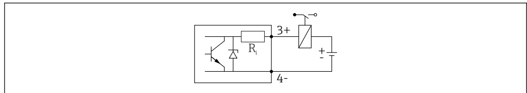
図 12 リレーの接続例
