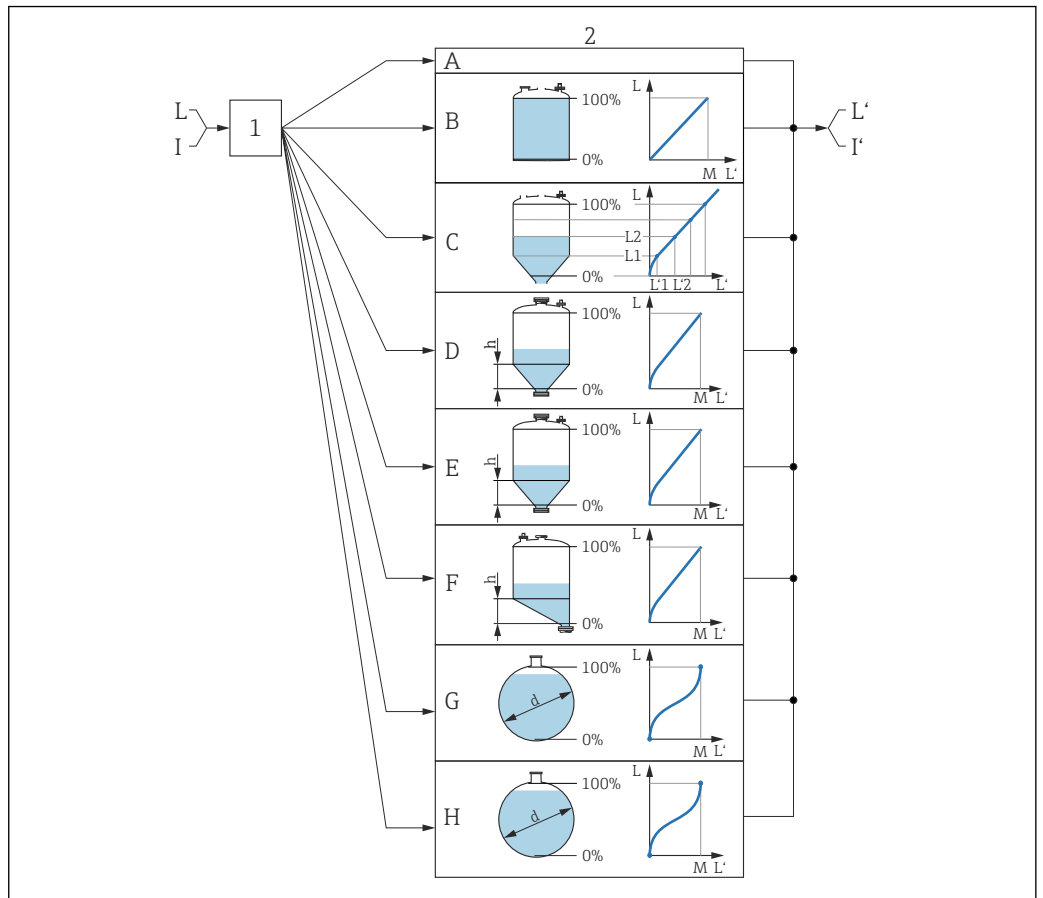
48 リニアライゼーション：レベルから、および（該当する場合は）界面から体積または質量に変換。変換は容器の形状に依存
