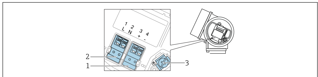
図 18 端子の割当て、4線式：4~20 mA HART (90~253 V AC )
