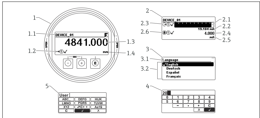
図 28 表示モジュールおよび操作モジュールの表示形式
