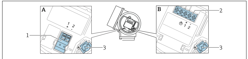
図 8 端子の割当て、2線式：4～20 mA HART
