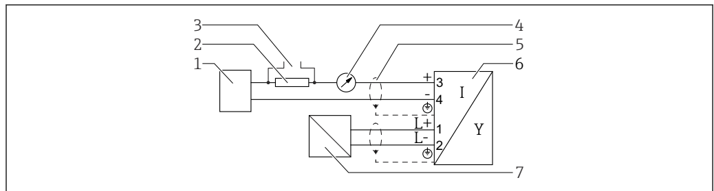
図 17 機能図、4線式：4~20 mA HART (10.4~48 V DC )
