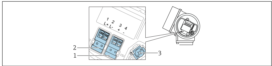
図 16 端子の割当て、4線式：4~20 mA HART (10.4~48 V DC )
