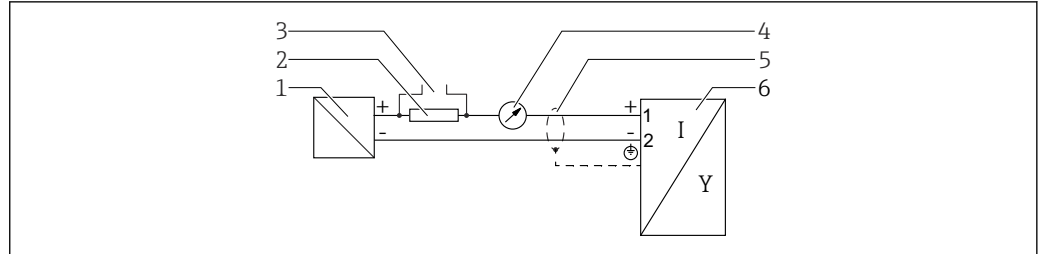
図 9 機能図：4～20 mA HART
