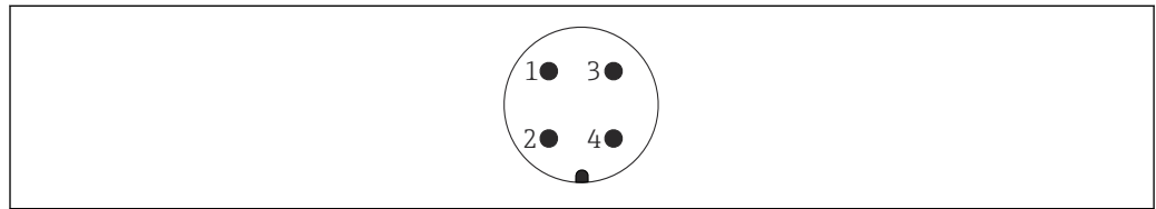
图 21 7/8"插头的针脚分配
