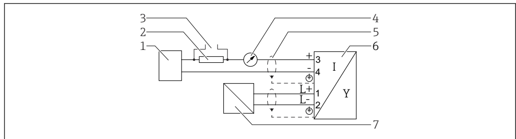
图 17 功能框图, 四线制: 4 ... 20 mA HART (10.4 ... 48 V DC )
