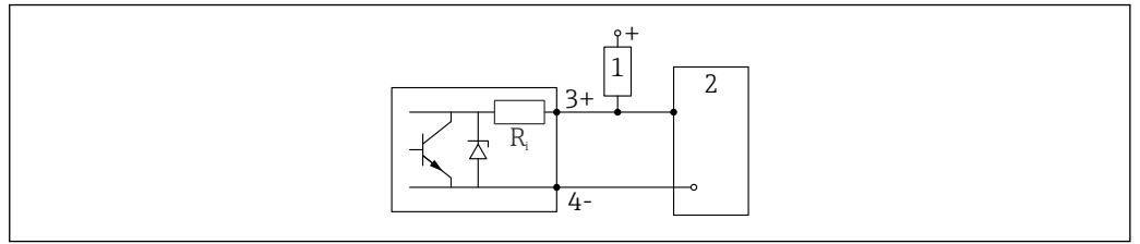
图 13 数字量输入的连接示例
