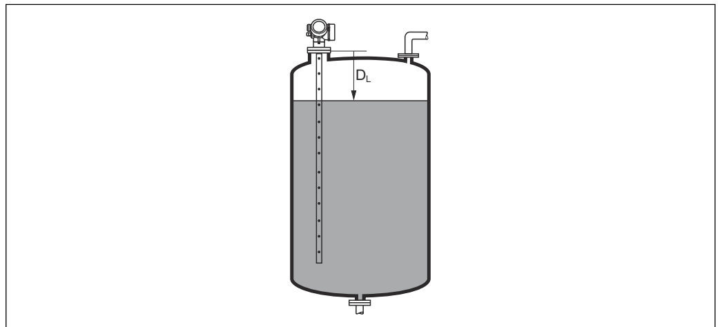
46 液位测量时的距离
