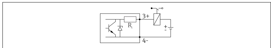
图 12 继电器的连接示例
