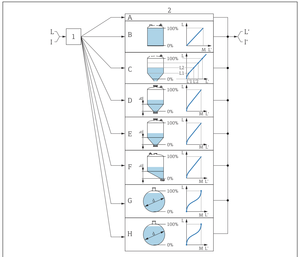
48 线性化：将物位和（相关）界面高度转换成体积或重量；转换取决于罐体形状
