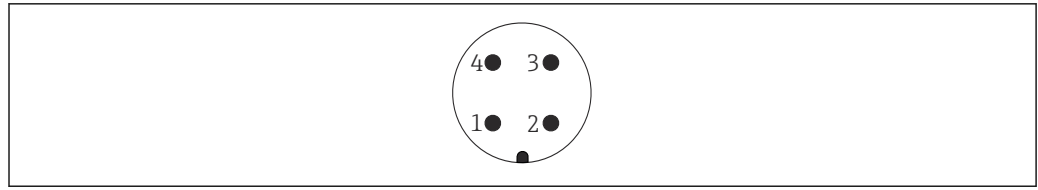
图 20 M12 插头的针脚分配
