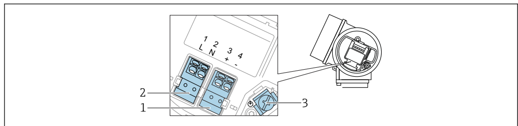
图 18 接线端子分配, 四线制: 4 ... 20 mA HART (90 ... 253 V AC )
