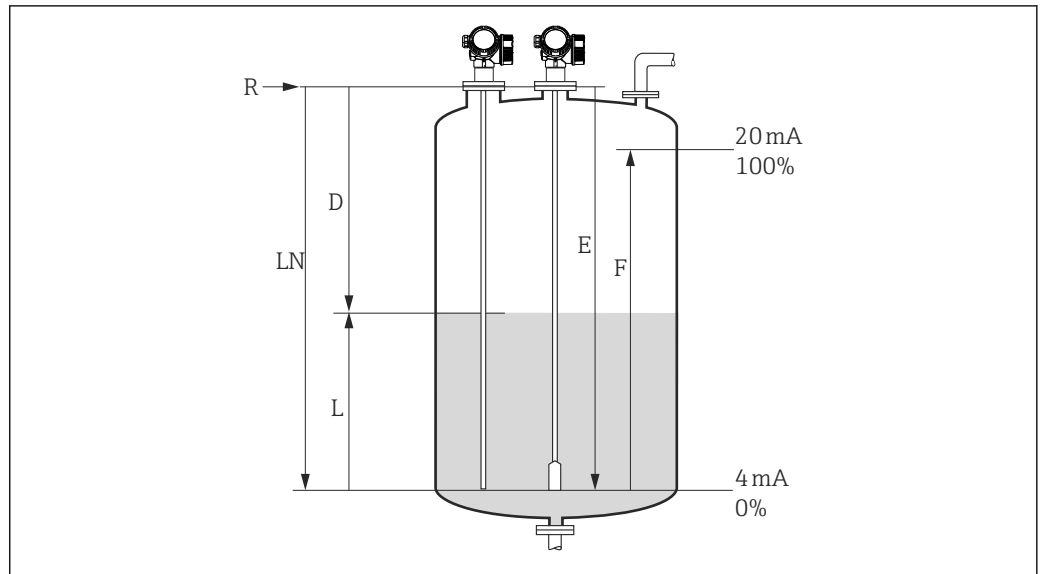
图 33 液位测量的设置参数
