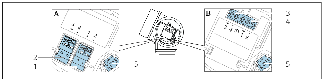
图 14 接线端子分配, 两线制: 4 ... 20 mA HART, 4 ... 20 mA
