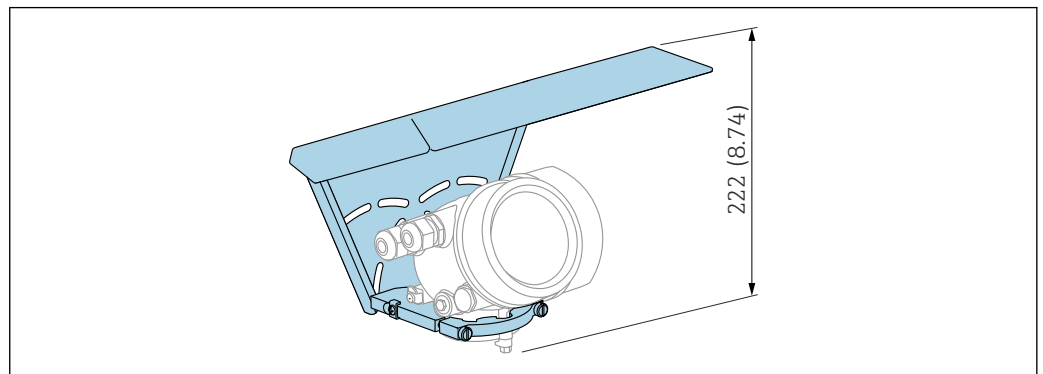
38 高度。测量单位 mm (in)
