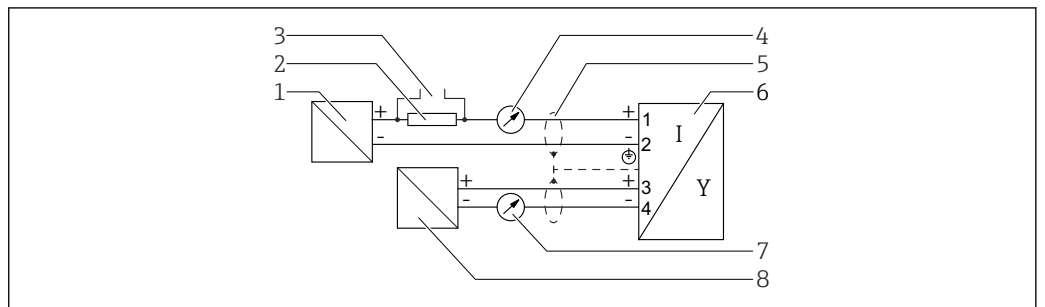
图 15 功能框图: 4 ... 20 mA HART + 4 ... 20 mA 模拟量
