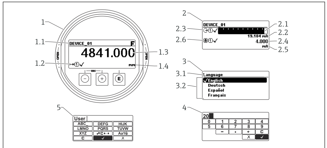
图 28 显示与操作单元的显示格式
