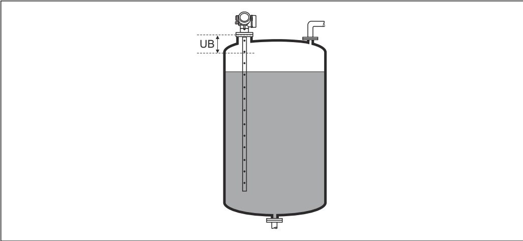
50 液位测量的盲区距离 (UB)
