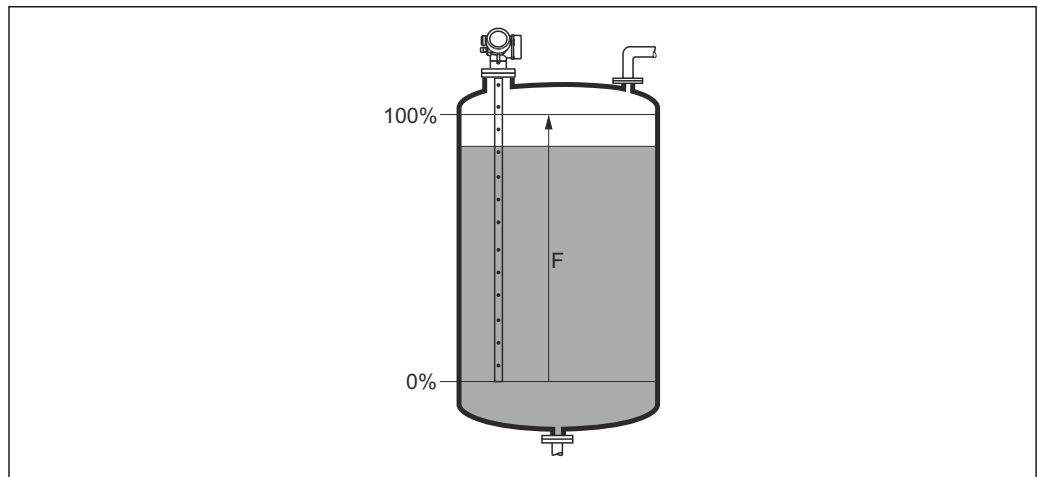
图 44 液位测量时的满标 (F)
