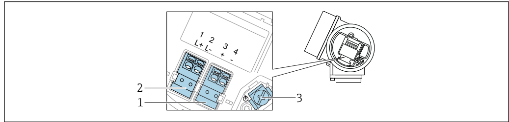
图 16 接线端子分配, 四线制: 4 ... 20 mA HART (10.4 ... 48 V DC )
