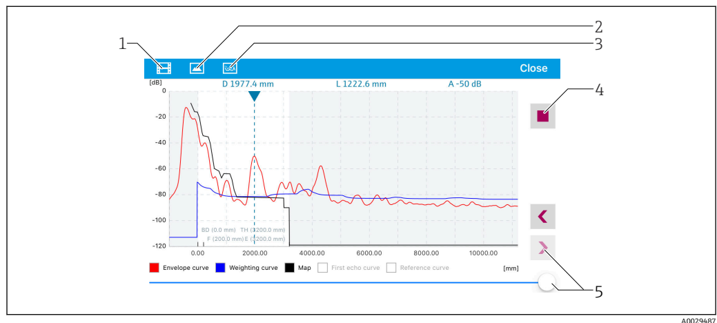
图 31 实例：iOS 设备使用 SmartBlue 显示包络线
