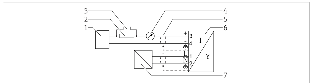
图 19 功能框图，四线制：4 ... 20 mA HART (90 ... 253 V AC )
