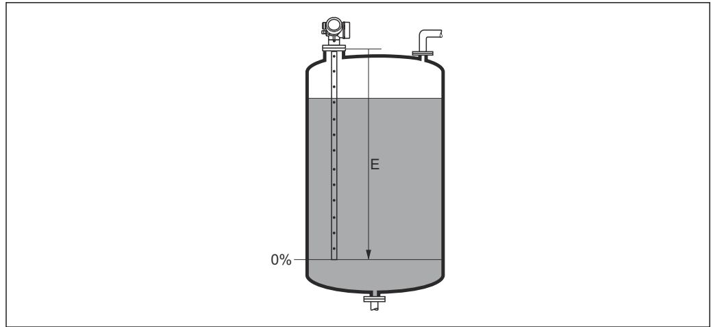
图 43 液位测量时的空标 (E)
