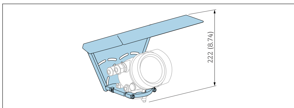
38 Hauteur. Unité de mesure mm (in)
