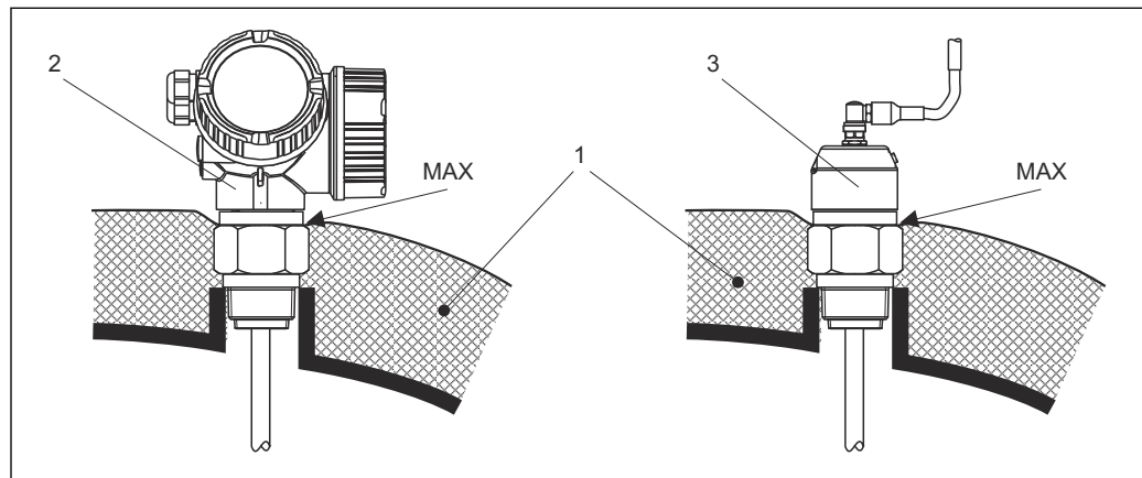
5 Raccord process avec filetage
