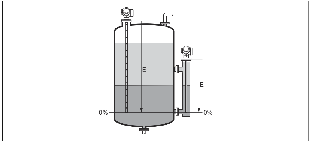
51 界面测量时空标 (E)
