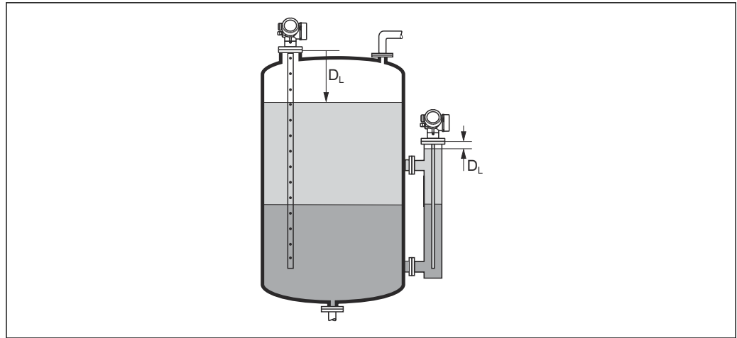
图 57 界面测量时的距离
