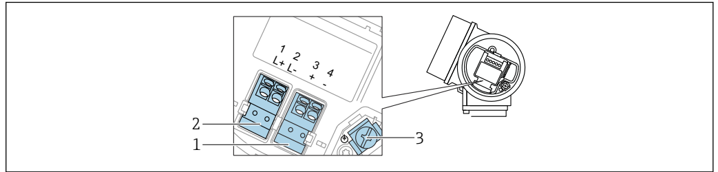
20 接线端子分配, 四线制: 4 ... 20 mA HART (10.4 ... 48 V DC )
