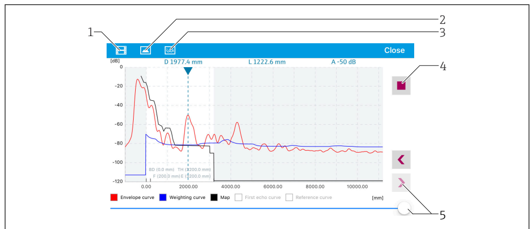
图 36 实例：iOS 设备使用 SmartBlue 显示包络线
