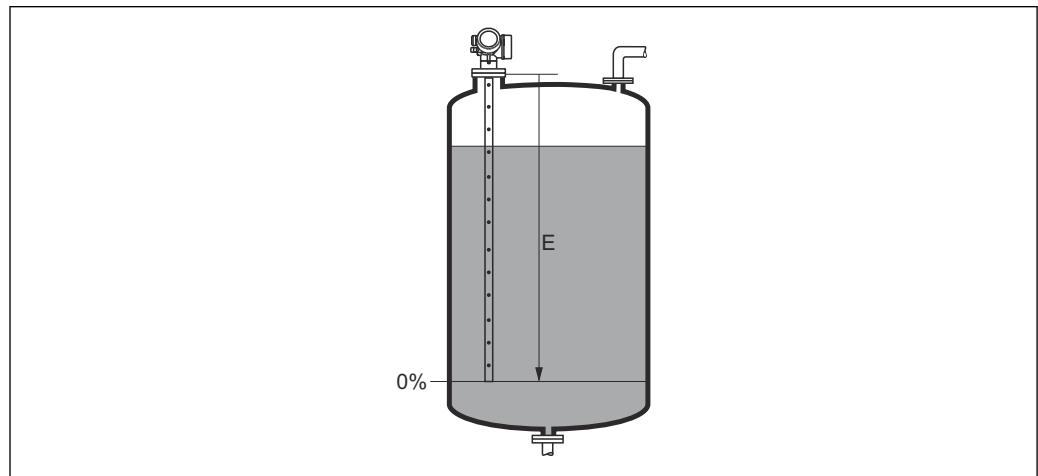
50 液位测量时的空标 (E)
