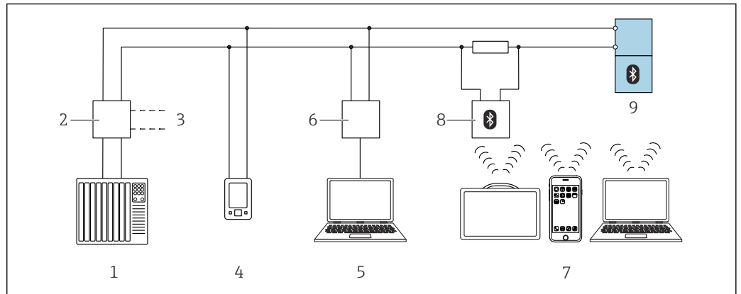
图 30 通过 HART 通信实现远程操作
