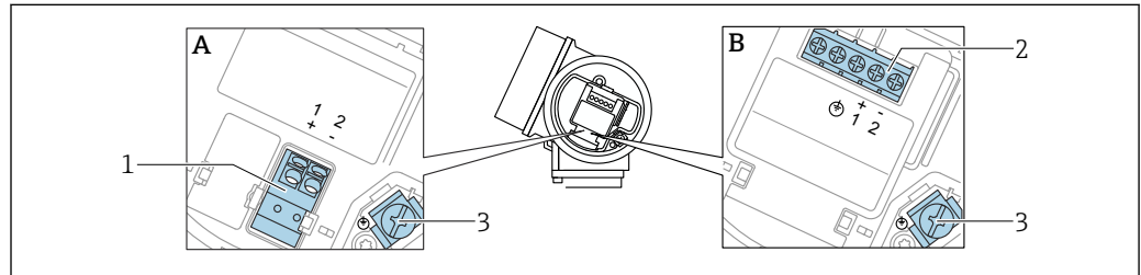
图 12 接线端子分配, 两线制: 4 ... 20 mA HART
