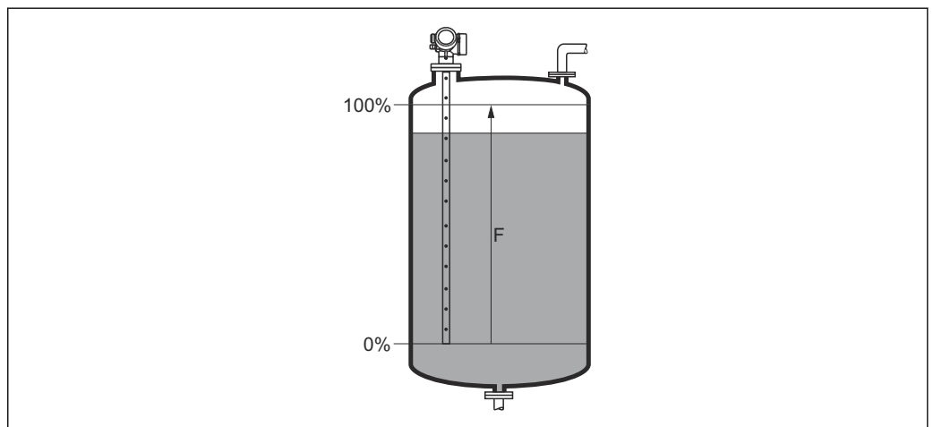
52 液位测量时的满标 (F)
