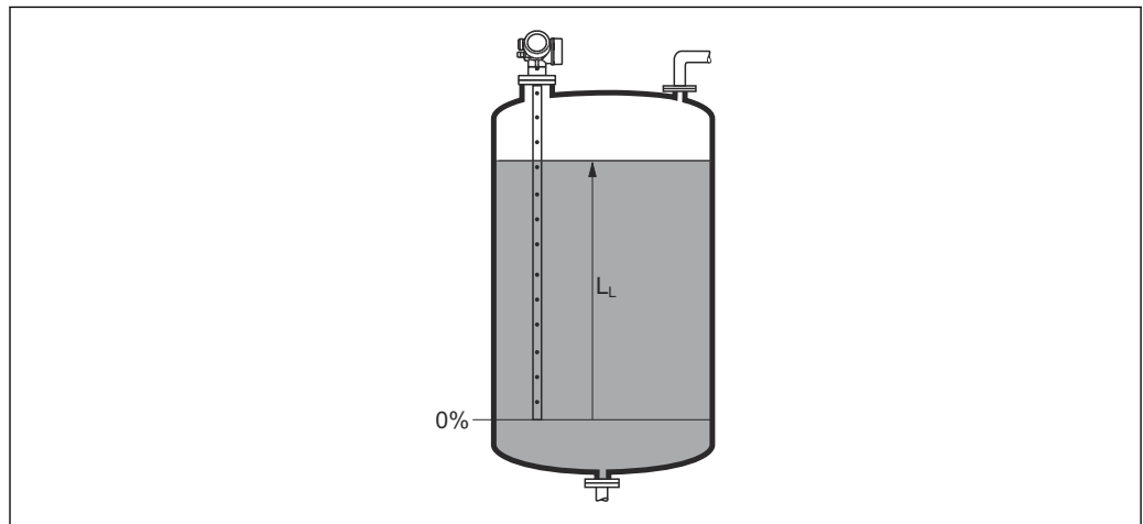
图 54 液位测量时的液位
