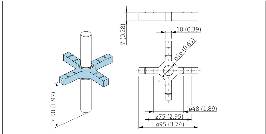
图 49 尺寸参数; \phi 48 \dots 95 \text{ mm} (1.89 ... 3.74 in) 对中环, PEEK
