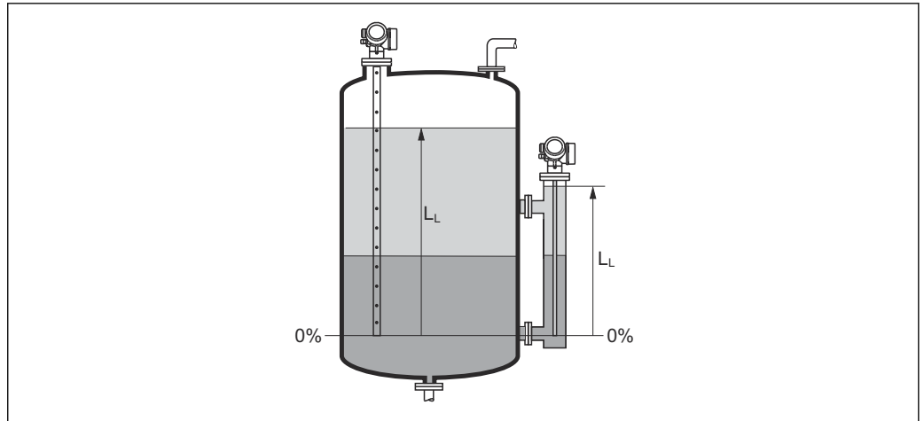
☑ 55 界面测量时的液位
