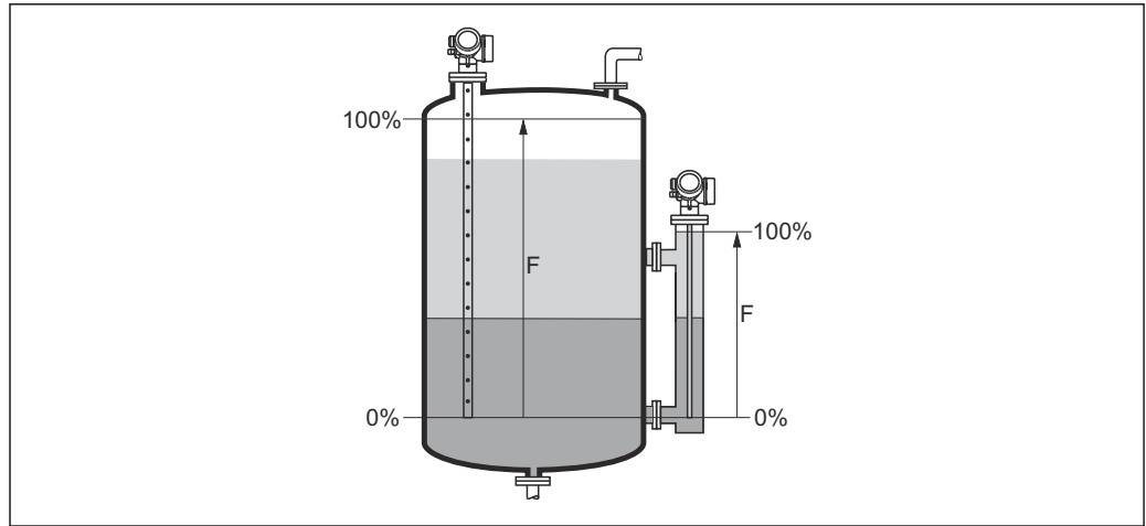
图 53 界面测量时的满标 (F)
