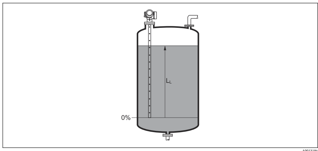
図 43 液体計測時のレベル
