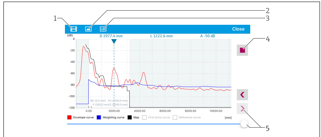
図 29 SmartBlue (iOS 版) での反射波形表示 (例)
