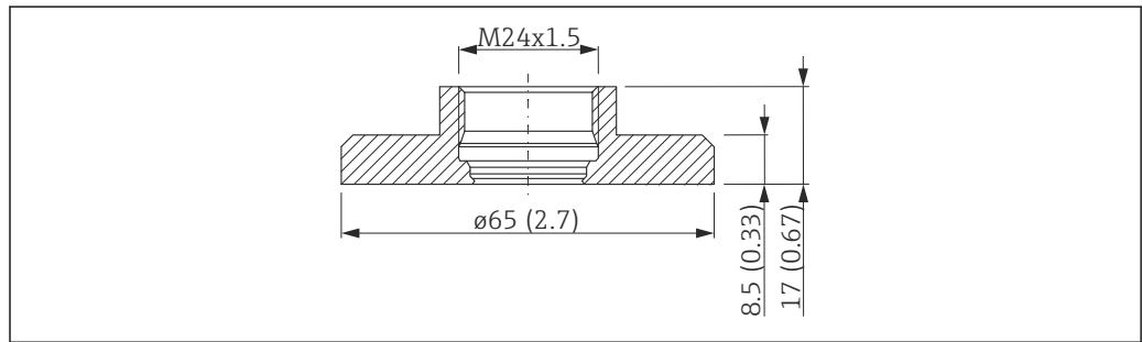
図 40 寸法、溶接アダプタ
