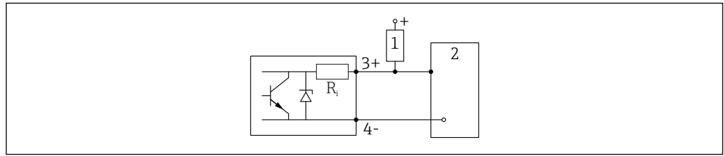
図 11 デジタル入力の接続例
