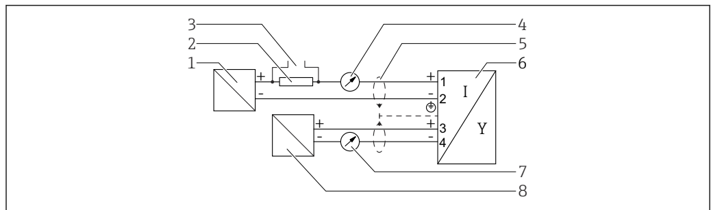
図 13 機能図：4~20 mA HART + 4~20 mA アナログ
