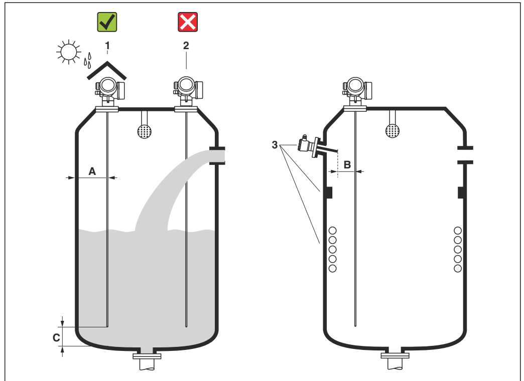
図 3 取付け位置
