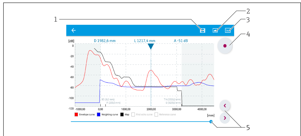
図 28 SmartBlue (Android 版) での反射波形表示 (例)
