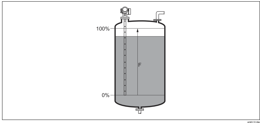
図 42 液体レベル測定用の満量校正 (F)
