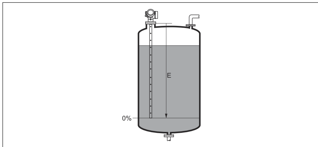
☰ 41 液体レベル測定用の空校正 (E)
