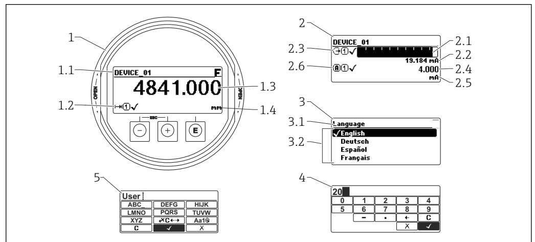
図 26 表示モジュールおよび操作モジュールの表示形式
