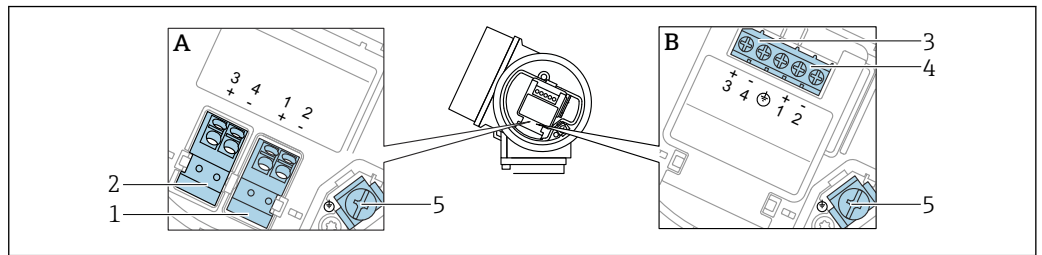
図 8 端子の割当て、2線式：4～20 mA HART、スイッチ出力
