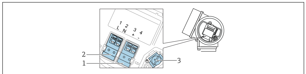
☑ 16 端子の割当て、4線式：4~20 mA HART (90~253 V AC )
