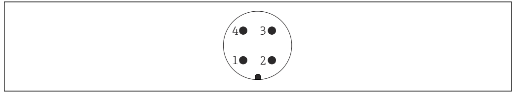
図 18 M12 プラグのピン割当て
