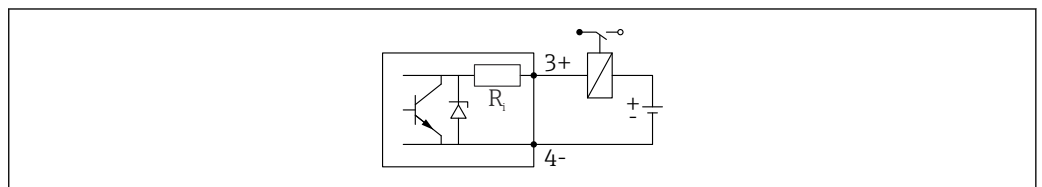
図 10 リレーの接続例
