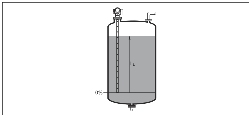
43 Nível em caso de medições de líquidos
