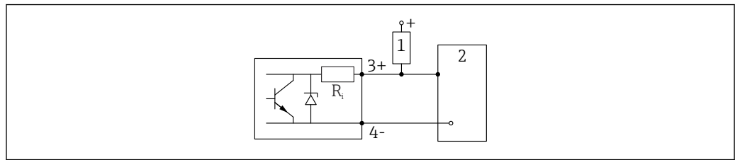
11 Exemplo de conexão para a entrada digital
