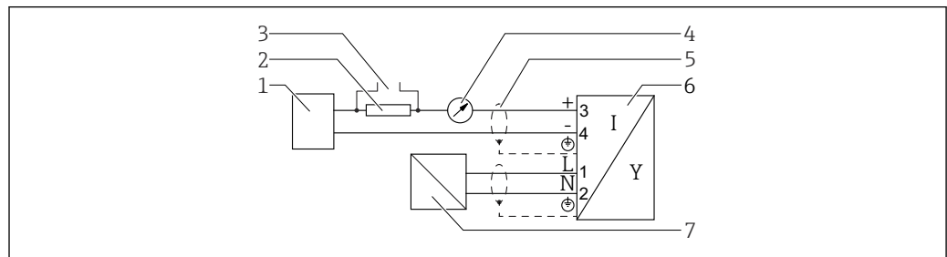
Fig. 17 Diagrama de função de 4 fios: HART 4 para 20 mA (90 para 253 V AC )
