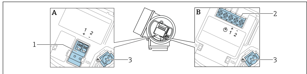
▣ 6 Esquema de ligação elétrica, 2 fios: 4 para 20 mA HART
