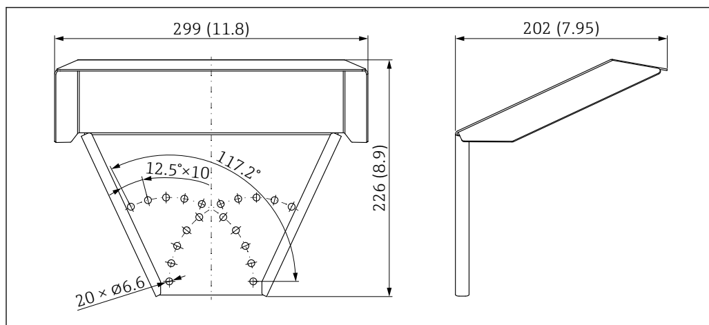
37 Dimensões. Unidade de medida mm (in)
