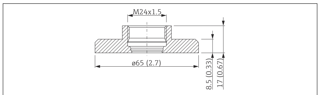
40 Dimensões, adaptador soldado
