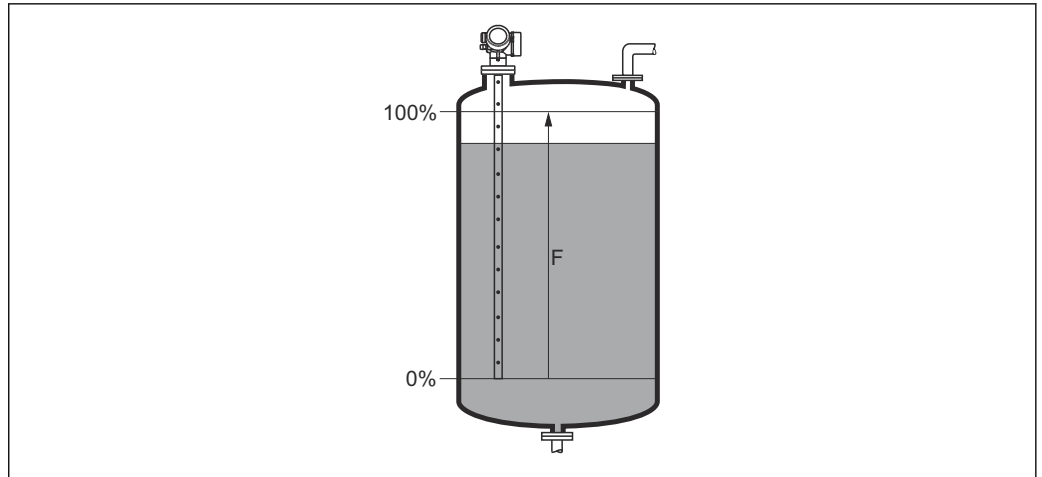
42 Калибровка полной емкости (F) для измерения уровня жидких сред
