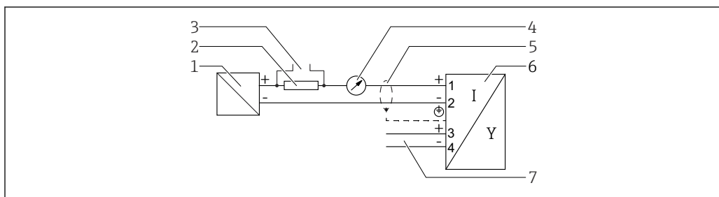
9 Функциональная схема 4 до 20 мА HART, релейный выход
