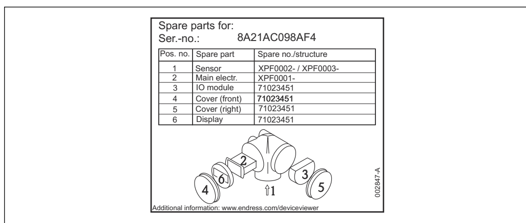
34 Пример заводской таблички с перечнем запасных частей, размещаемой на крышке присоединительного отсека
