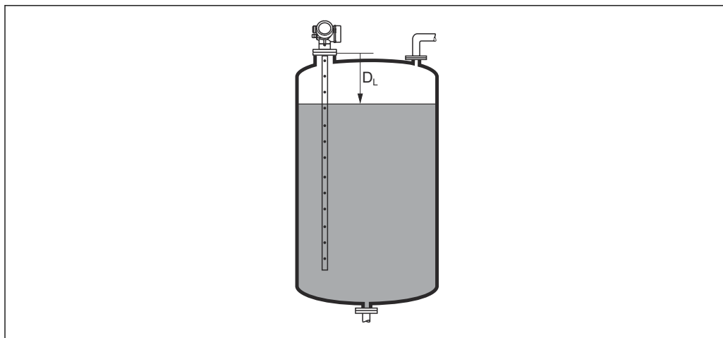
44 Расстояние для измерения в жидких средах
