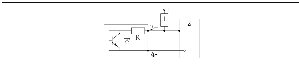
11 Пример подключения через цифровой вход
