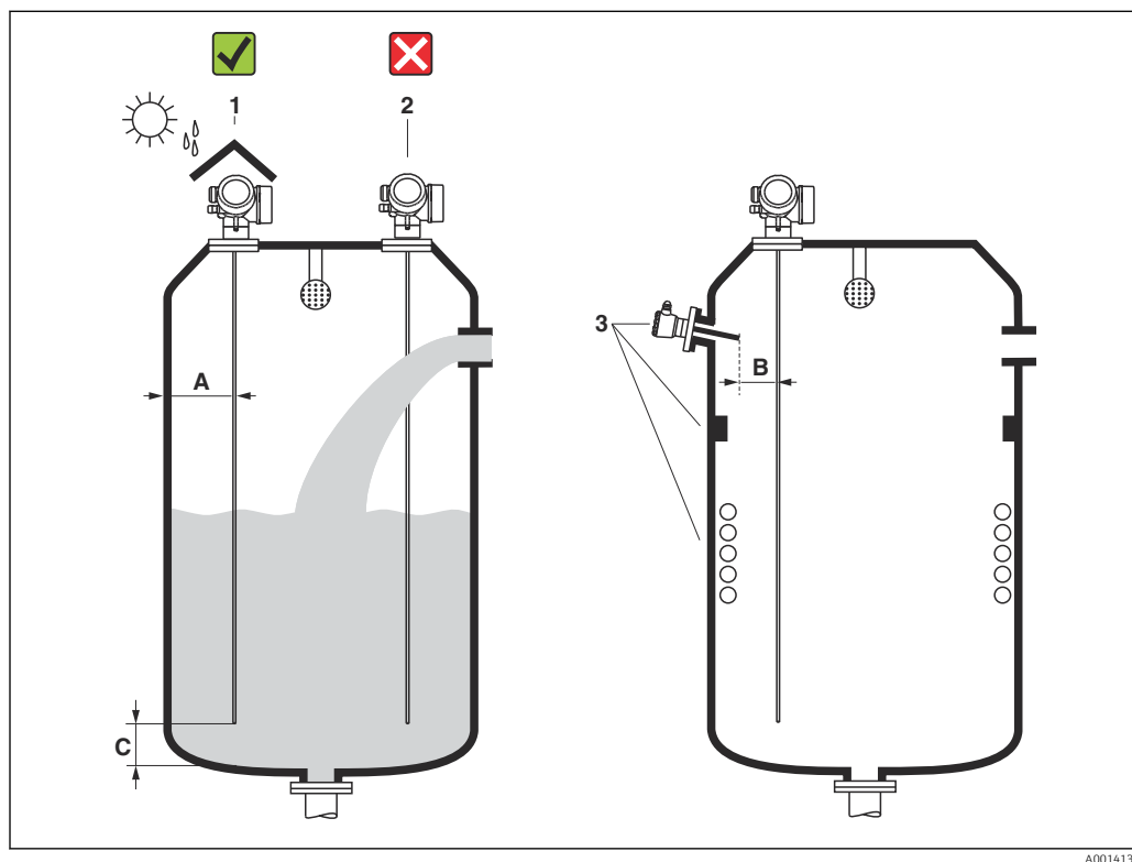
3 Положения установки
