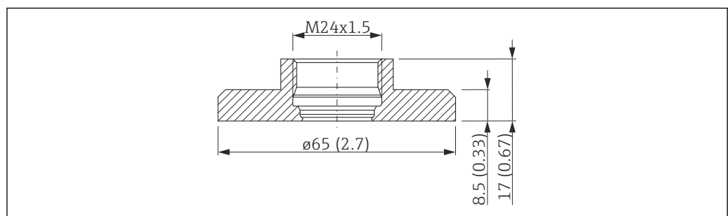
40 Размеры; приварной переходник
