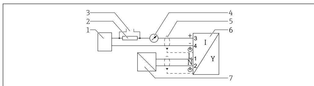
17 Функциональная схема 4-проводного подключения: 4 до 20 мА HART (90 до 253 В АС )
