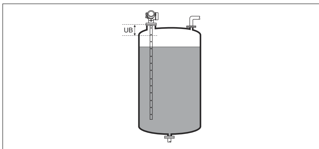
45 Блокирующая дистанция (UB) для измерения в жидких средах
