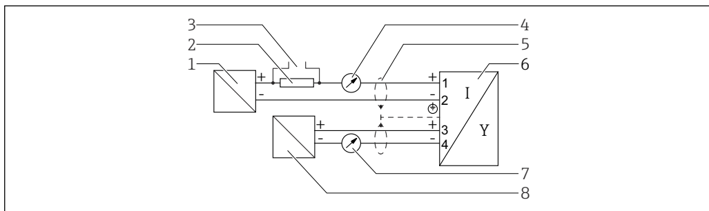
13 Функциональная схема 4 до 20 мА HART + 4 до 20 мА аналоговый
