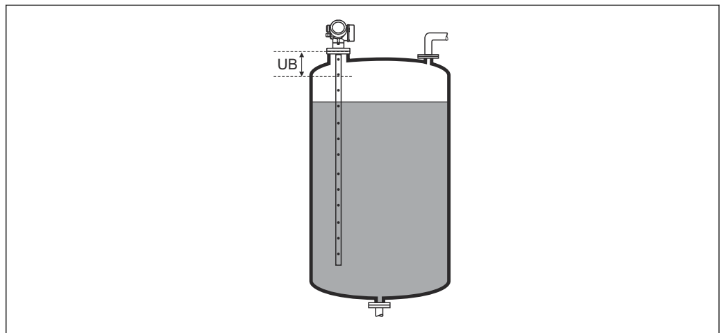
48 Блокирующая дистанция (UB) для измерения в жидких средах
