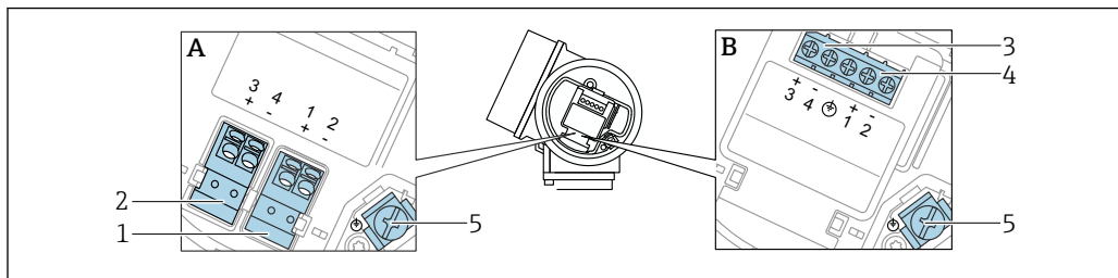
8 Назначение клемм, 2-проводное подключение: 4 до 20 мА HART, релейный выход
