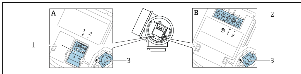
6 Назначение клемм, 2-проводное подключение: 4 до 20 мА HART
