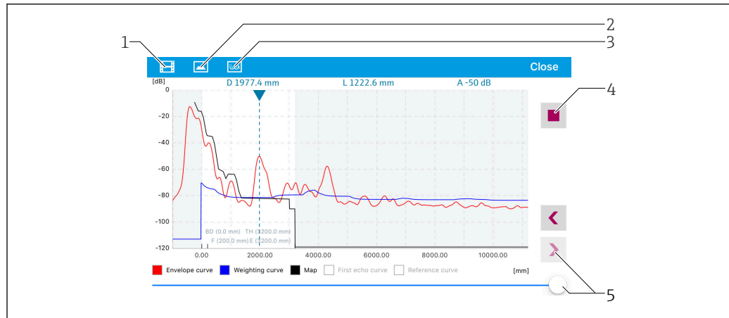
29 Visualización de la curva envolvente (muestra) en SmartBlue para iOS
