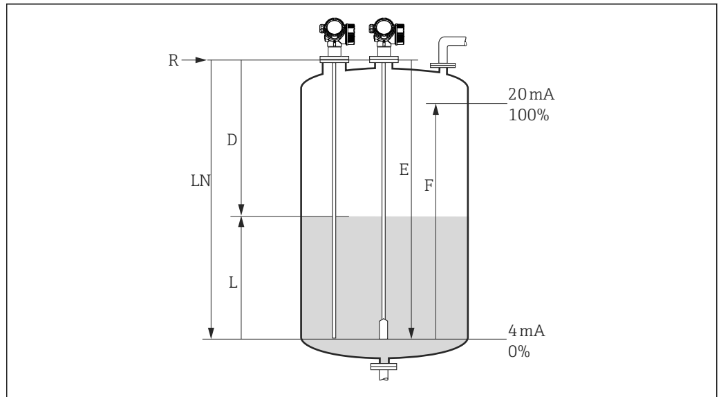
31 Parámetros de configuración para la medición de nivel en líquidos
