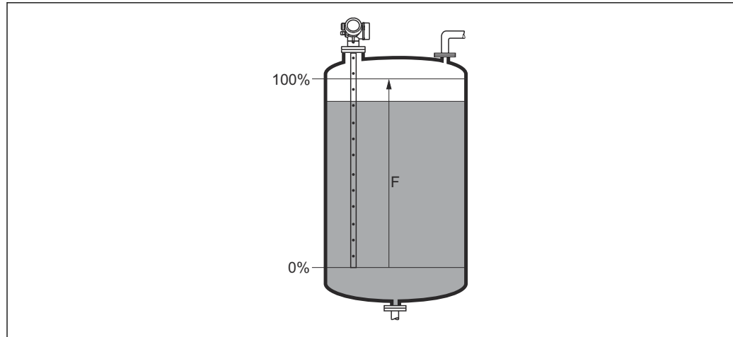
42 Calibración lleno (F) para mediciones de nivel en líquidos
