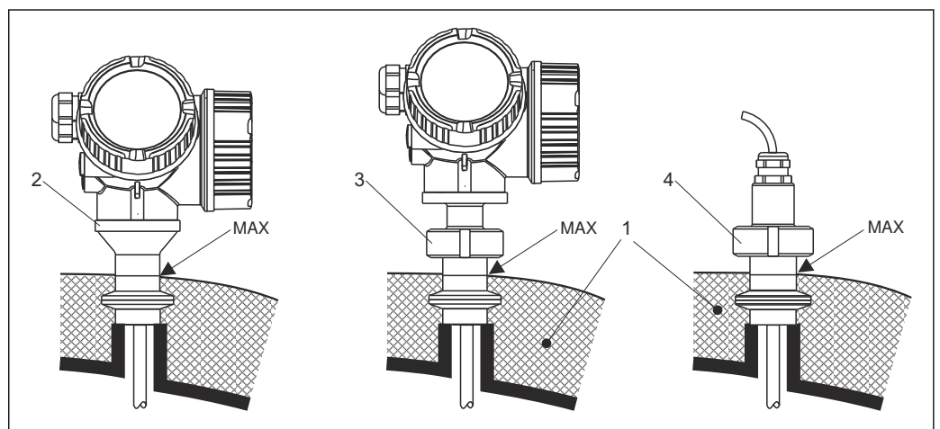
4 Conexiones a proceso higiénico
