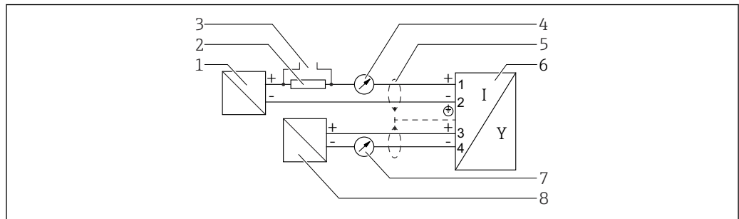
13 Diagrama de funciones de 4 ... 20 mA HART + 4 ... 20 mA analógica
