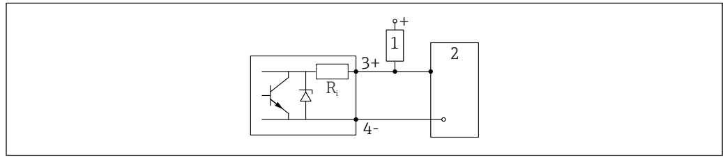
11 Ejemplo de conexión para la entrada digital
