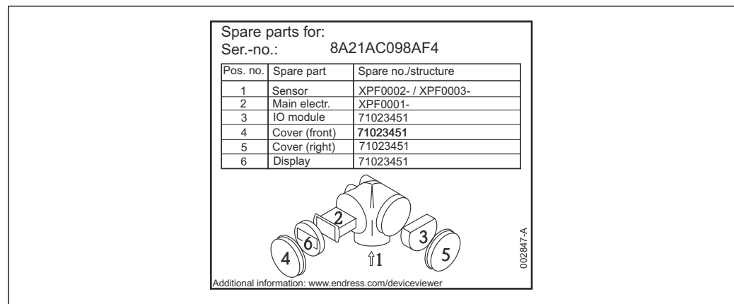
34 Ejemplo de una placa de identificación de piezas de repuesto en la cubierta del compartimento de conexiones
