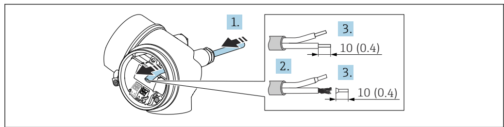
23 Unidad física: mm (in)
