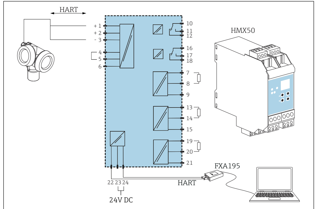
20 Diagrama de conexión del convertidor de lazo HART HMX50 (ejemplo: instrumento pasivo a 2 hilos y salidas de corriente conectados como fuentes de alimentación)
