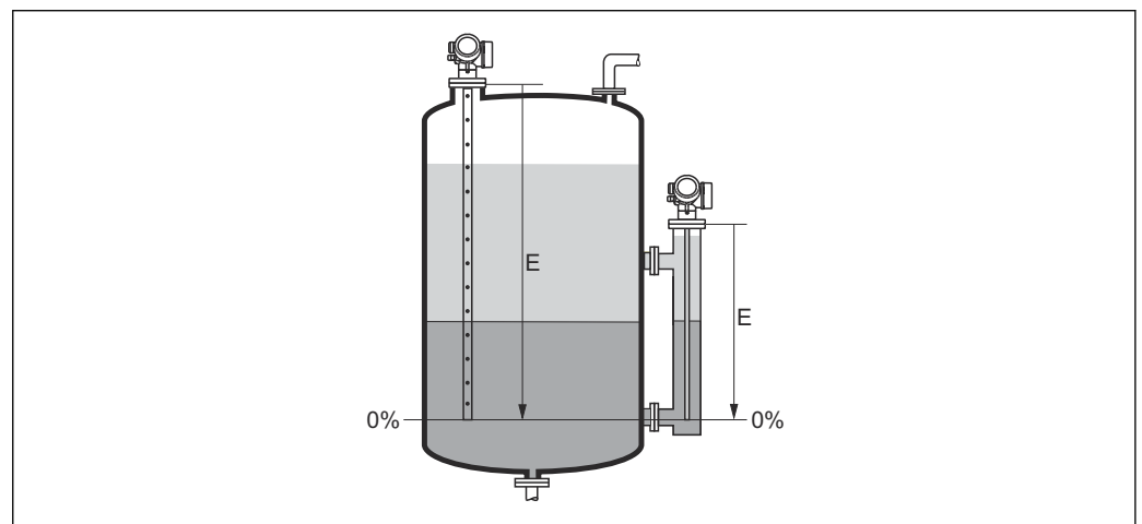
41 Calibración vacío (E) para mediciones de la interfase
