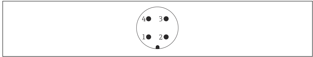
21 Asignación de pins del conector M12
