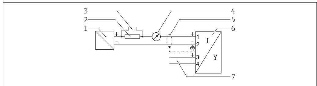
11 Diagrama de bloques, a 2 hilos: 4 ... 20 mA HART, salida de conmutación
