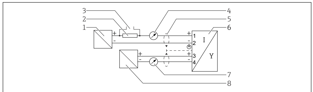
13 Diagrama de bloques, a 2 hilos: 4 ... 20 mA HART, 4 ... 20 mA
