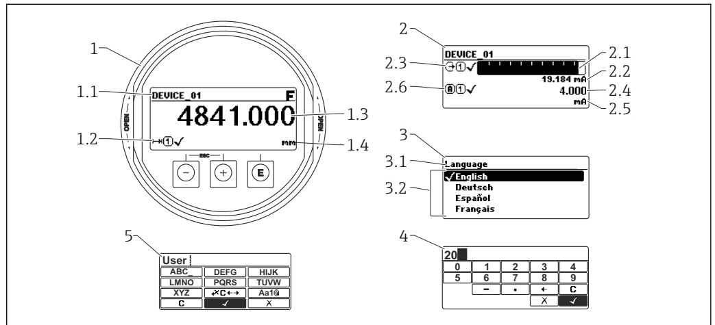
Fig. 29 Formato de indicación en el módulo indicador y de configuración
