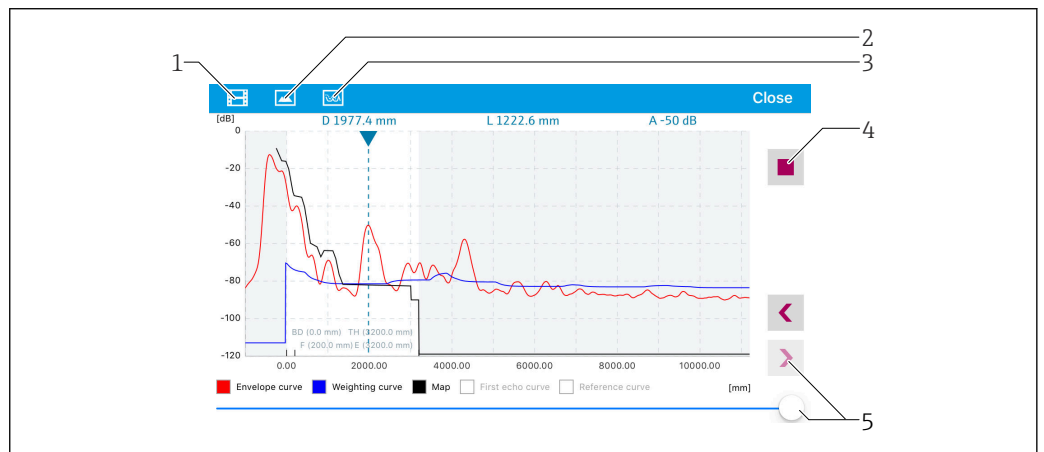
32 Visualización de la curva envolvente (muestra) en SmartBlue para iOS
