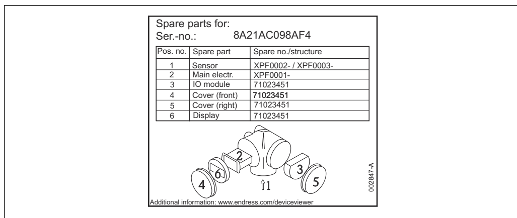
Fig. 37 Ejemplo de una placa de identificación de piezas de repuesto en la tapa del compartimento de conexiones
