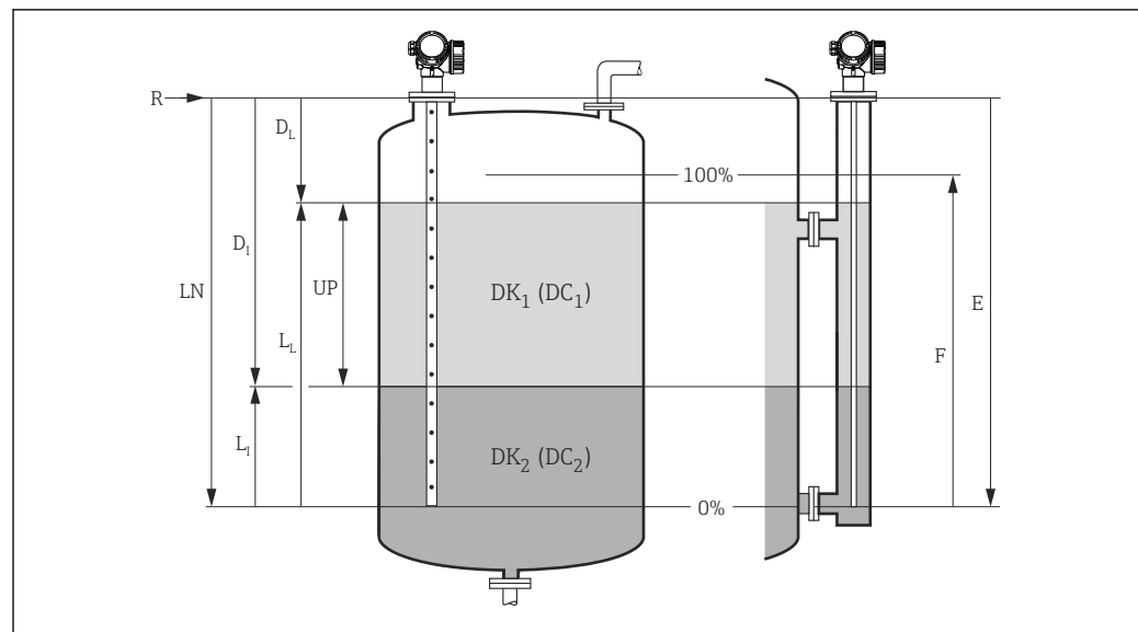
34 Parámetros de configuración para la medición de la interfase
