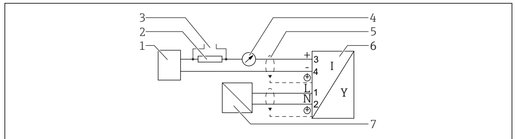
17 Diagrama de bloques, a 4 hilos: 4 ... 20 mA HART (90 ... 253 V AC )
