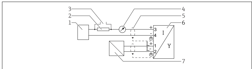
15 Diagrama de bloques, a 4 hilos: 4 ... 20 mA HART (10,4 ... 48 V DC )
