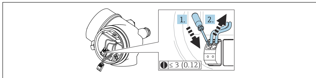
Fig. 24 Unidad física: mm (in)
