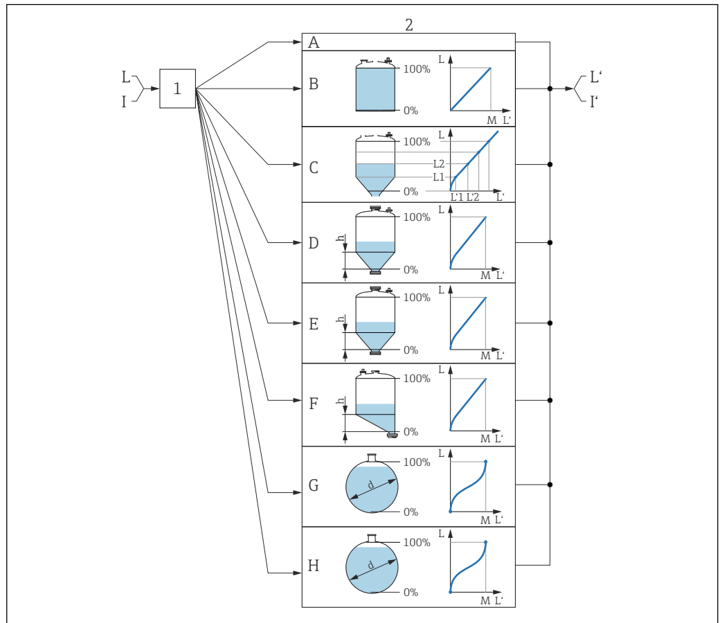
45 Linealización: conversión del nivel y, en caso aplicable, de la interfaz a un volumen o peso; la conversión depende de la forma del depósito
