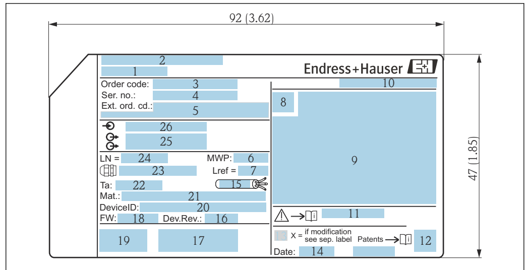
3 Placa de identificación del Levelflex; unidad física: mm (in)
