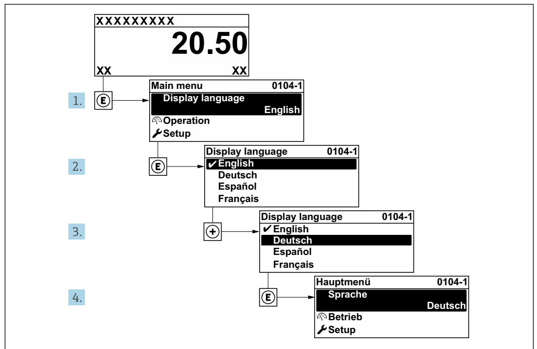
33 El indicador local como ejemplo
