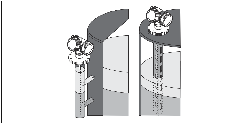
図 4 Levelflex FMP55 の取付位置
