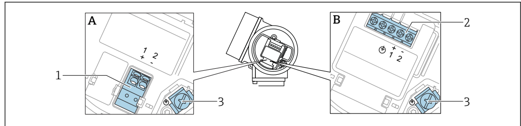
図 8 端子の割当て、2線式：4～20 mA HART
