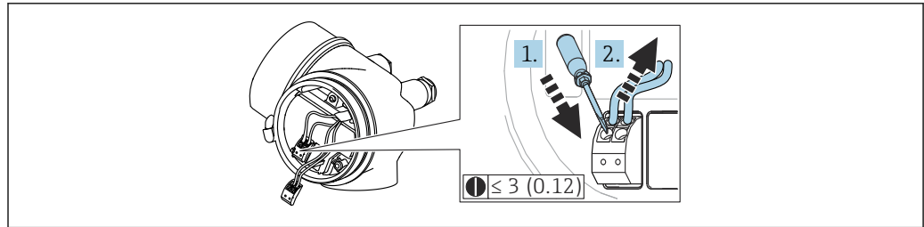
図 24 単位 : mm (in)
