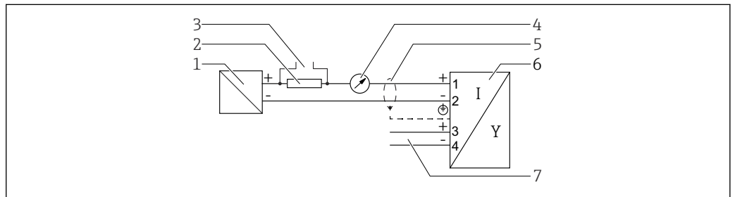
図 11 ブロック図、2線式：4~20 mA HART、スイッチ出力
