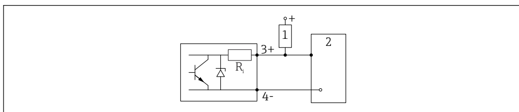
図 19 デジタル入力の接続
