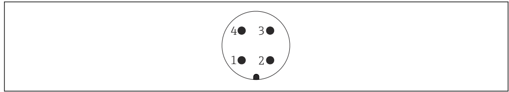
図 21 M12 プラグのピン割当て
