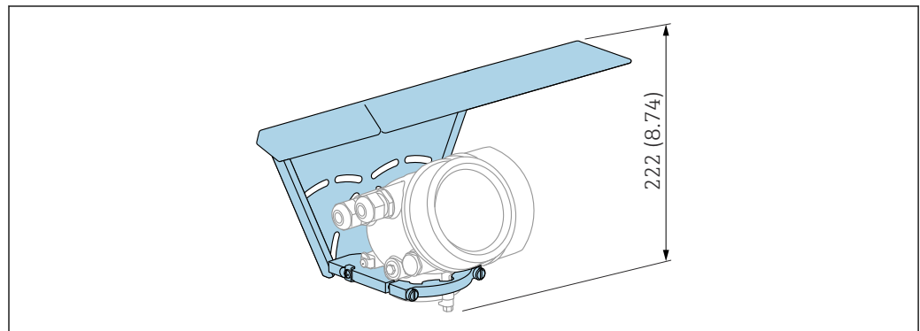
図 38 高さ。測定単位 mm (in)
