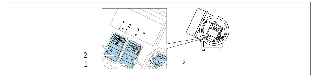
図 14 端子の割当て、4線式：4~20 mA HART（10.4~48 V DC ）
