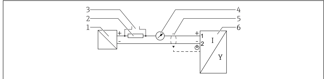
図 9 ブロック図、2線式：4～20 mA HART
