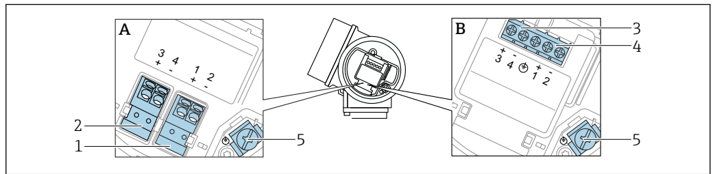
図 10 端子の割当て、2線式：4~20 mA HART、スイッチ出力
