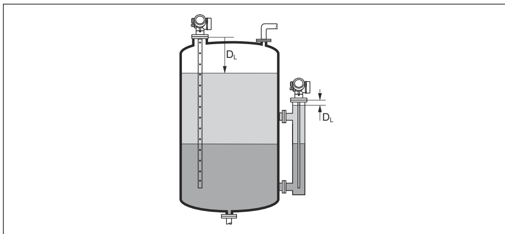
図 44 界面測定の距離
