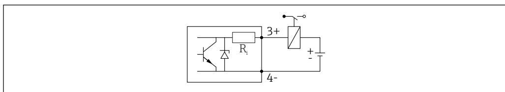
図 18 リレーの接続
