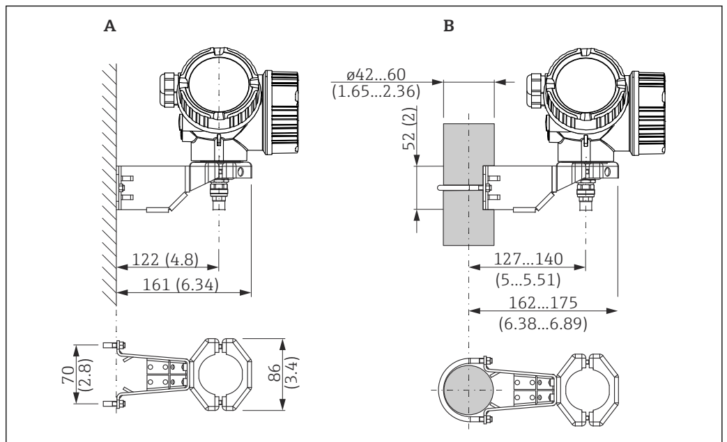
図 6 取付ブラケットを使用した電子部ハウジングの取付け。測定単位 mm (in)
