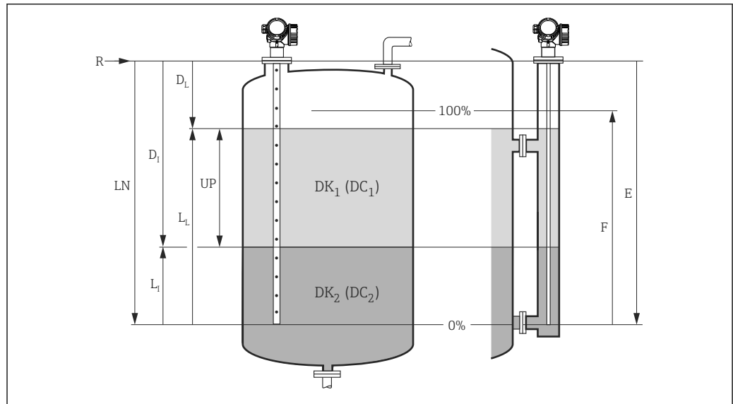
図 34 界面測定用パラメータの設定
