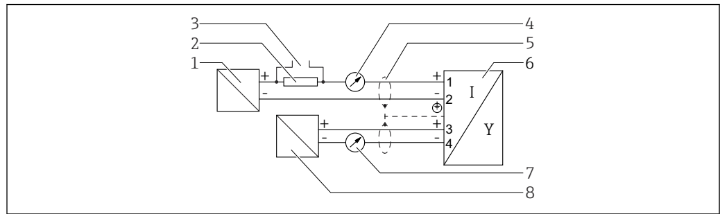
図 13 ブロック図、2線式：4~20 mA HART、4~20 mA
