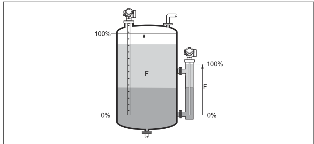
図 42 界面測定用の満量校正 (F)
