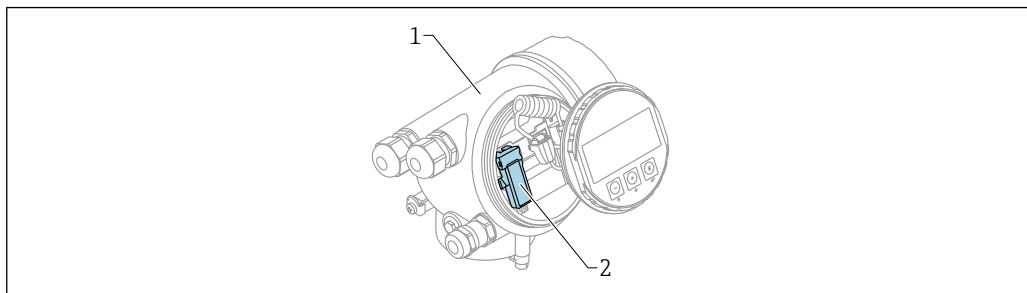
図 26 Bluetooth モジュール搭載の機器
