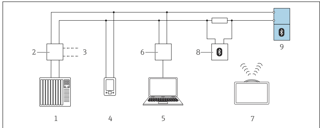
図 28 HART 経由のリモート操作オプション
