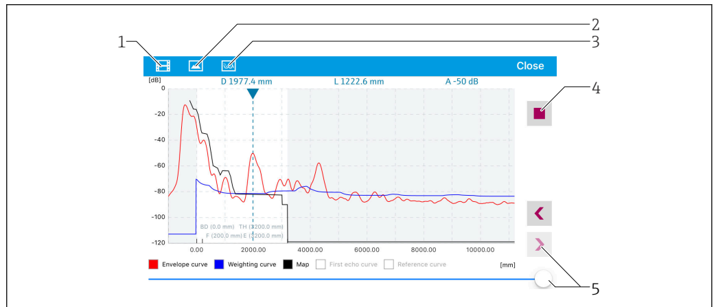
図 32 SmartBlue (iOS 版) での反射波形表示 (例)
