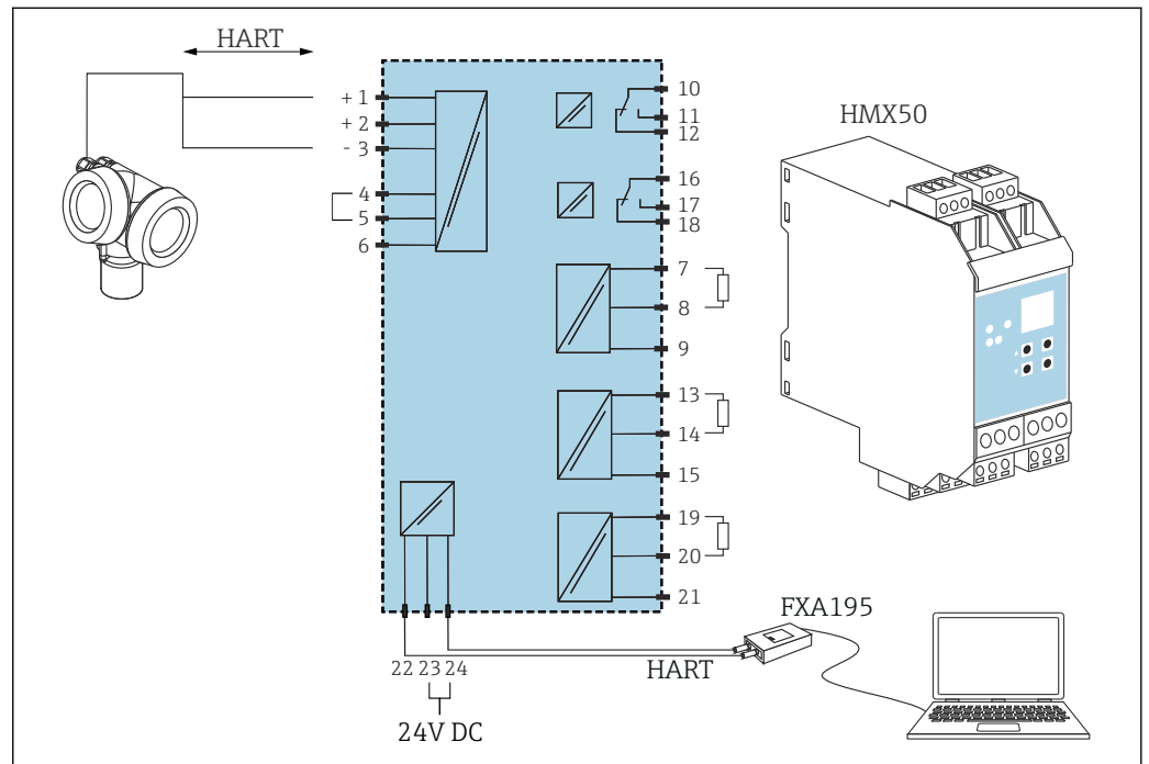
図 20 HART ループコンバータ HMX50 の接続図 (例：パッシブ 2 線機器と電流出力 (電源として接続))
