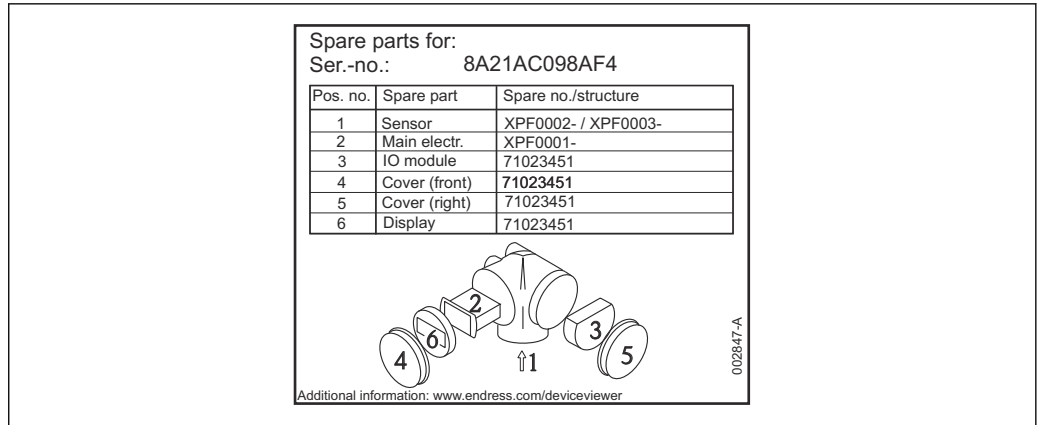
图 37 接线腔外壳内的备件铭牌示意图
