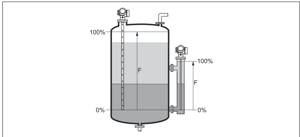
42 界面测量时的满标 (F)
