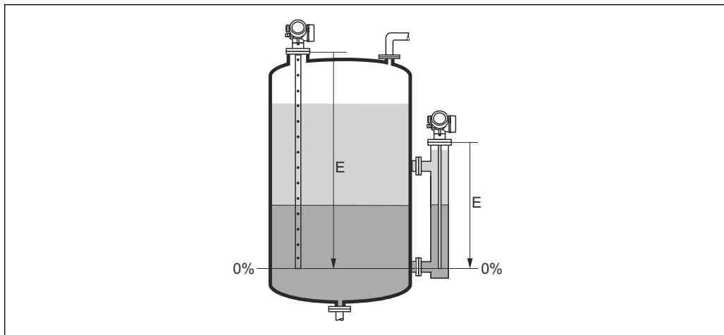
41 界面测量时的空标 (E)
