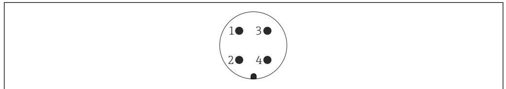
图 22 7/8"插头的针脚分配
