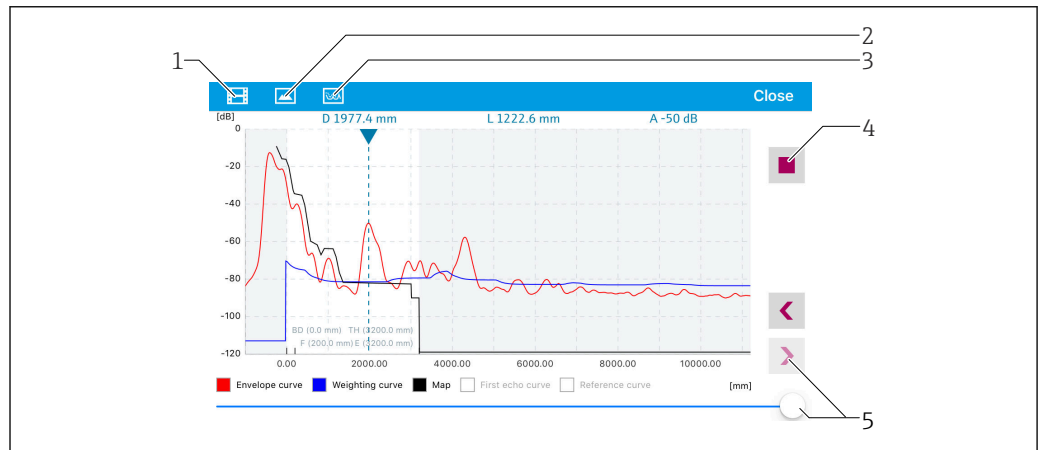
图 32 实例：iOS 设备使用 SmartBlue 显示包络线
