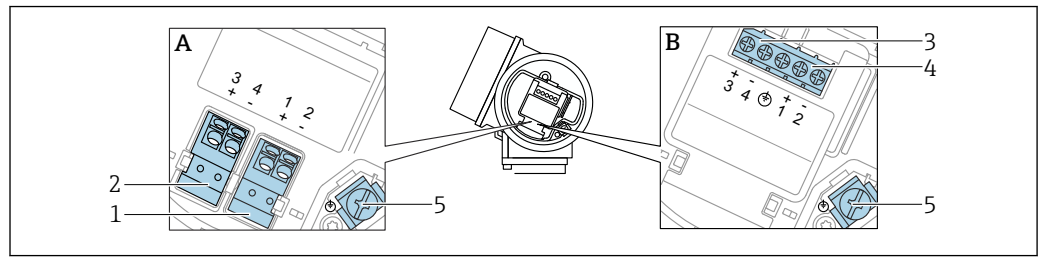
图 10 接线端子分配，两线制：4 ... 20 mA HART，开关量输出
