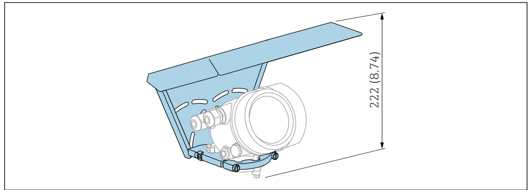
图 38 高度。测量单位 mm (in)
