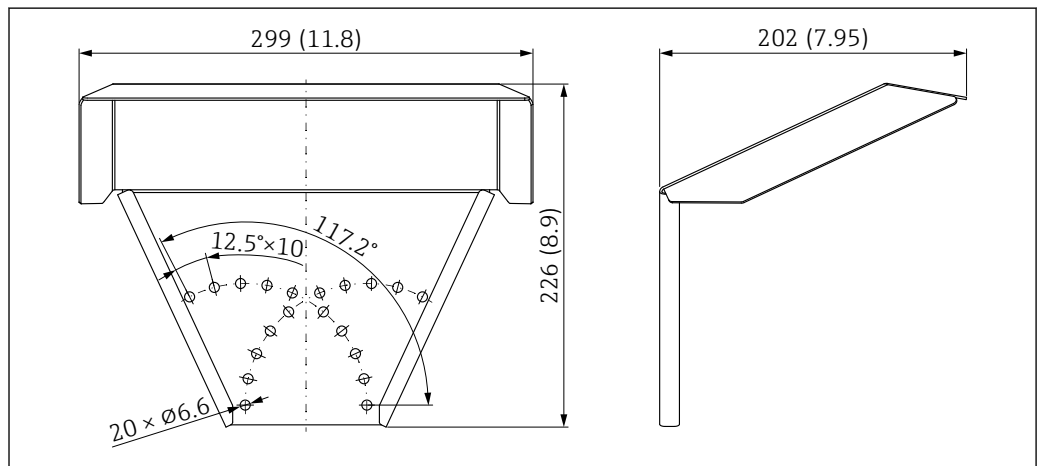
图 39 外形尺寸。测量单位 mm (in)
