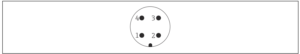
图 21 M12 插头的针脚分配
