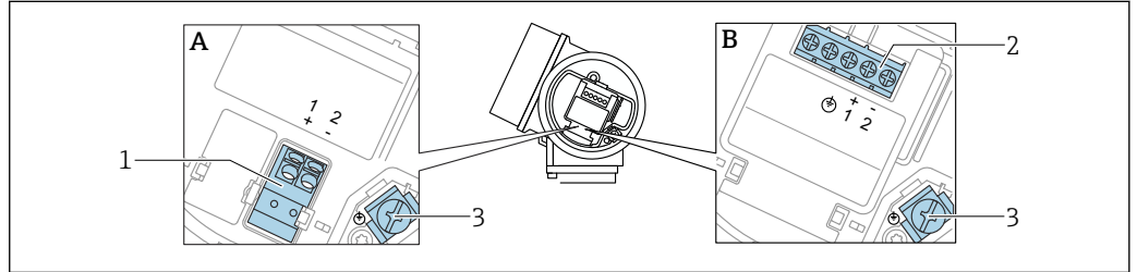
图 8 接线端子分配，两线制：4 ... 20 mA HART
