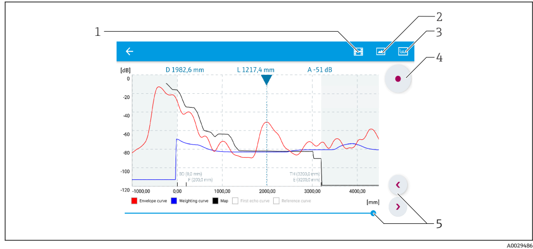
图 31 实例：Android 设备使用 SmartBlue 显示包络线
