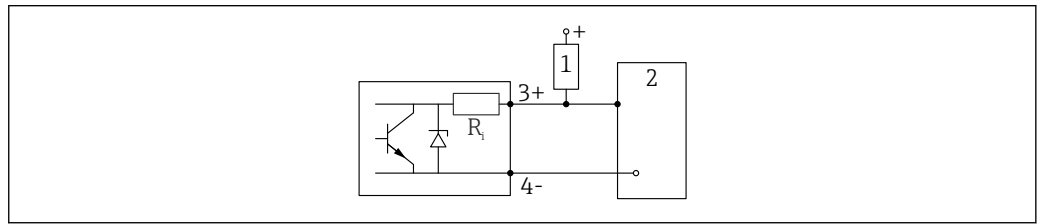
19 连接数字量输入
