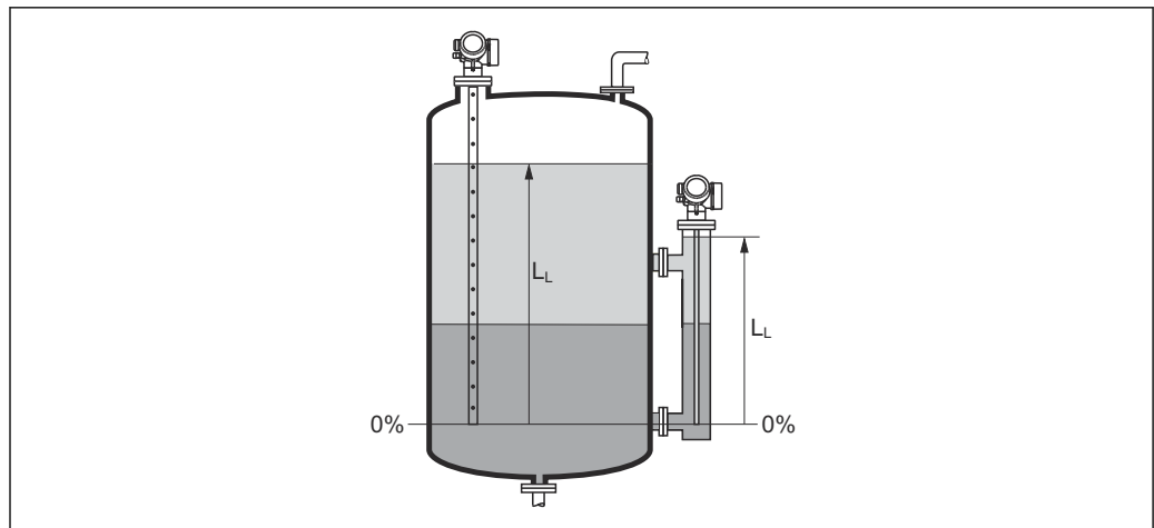
43 界面测量时的液位
