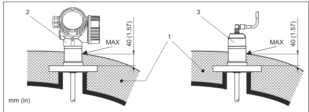
5 法兰过程连接
