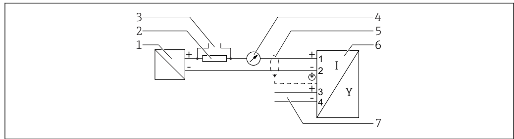
图 11 接线图：两线制：4 ... 20 mA HART，开关量输出
