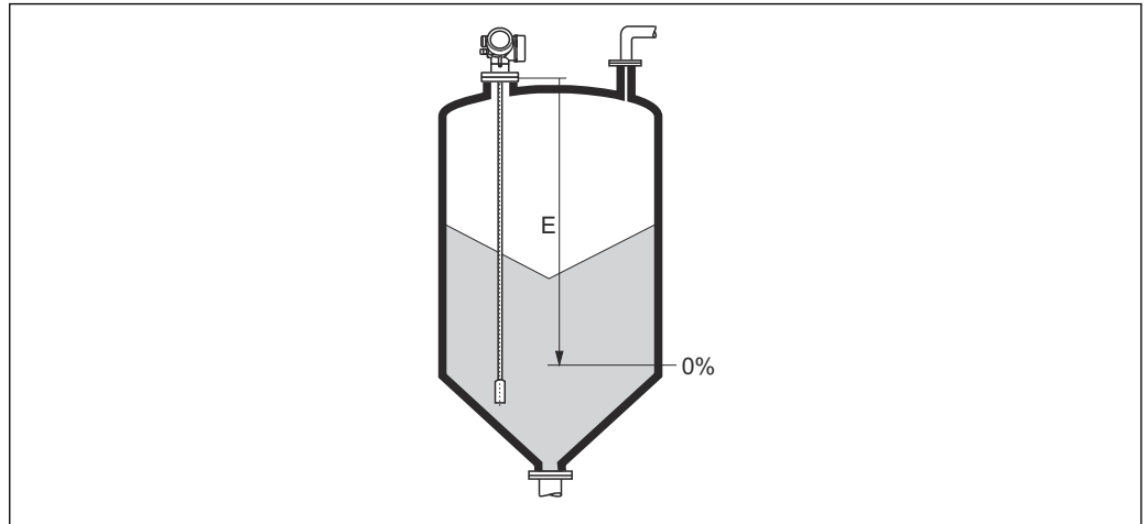
48 料位测量时的空标 (E)
