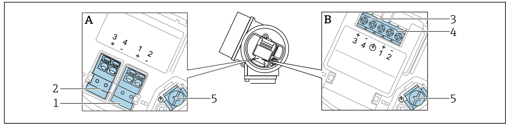
图 15 接线端子分配, 两线制: 4 ... 20 mA HART, 开关量输出
