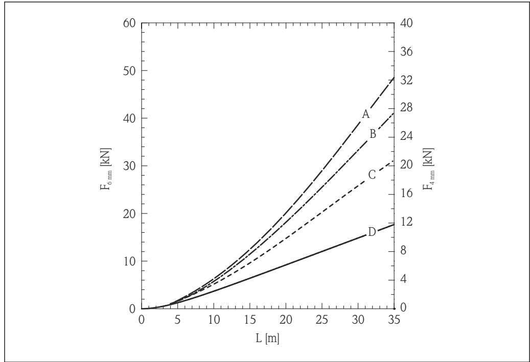
图 4 张力负载与物位 (L) 关系曲线图; 6 mm (0.24 in) 和 4 mm (0.16 in) 缆式探头, 石英砂料仓; 光滑金属仓壁
