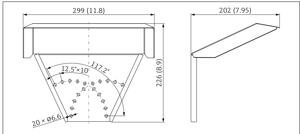
图 44 尺寸参数。测量单位 mm (in)
