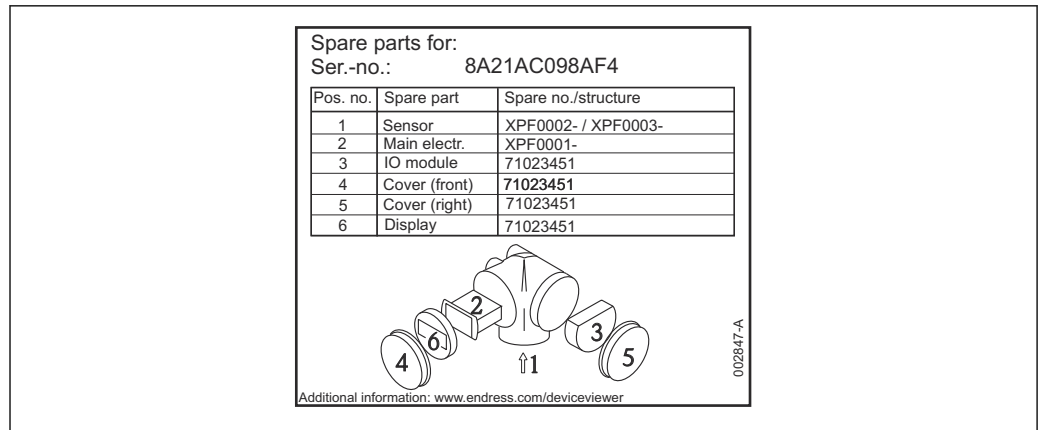
图 41 接线腔外壳内的备件铭牌示意图
