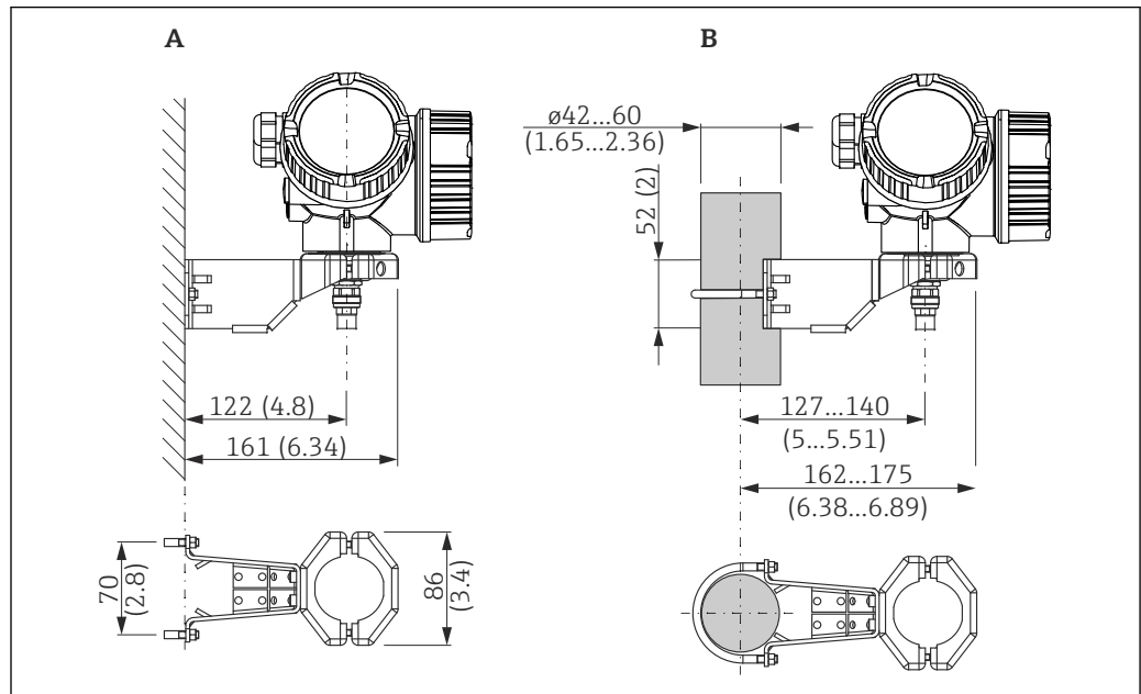
图 45 电子腔外壳安装架; 单位: mm (in)
