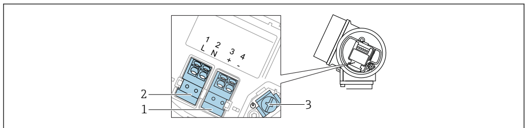
图 23 接线端子分配, 四线制: 4 ... 20 mA HART (90 ... 253 V AC )
