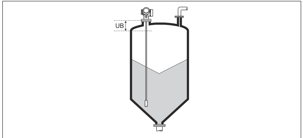
52 料位测量的盲区距离 (UB)
