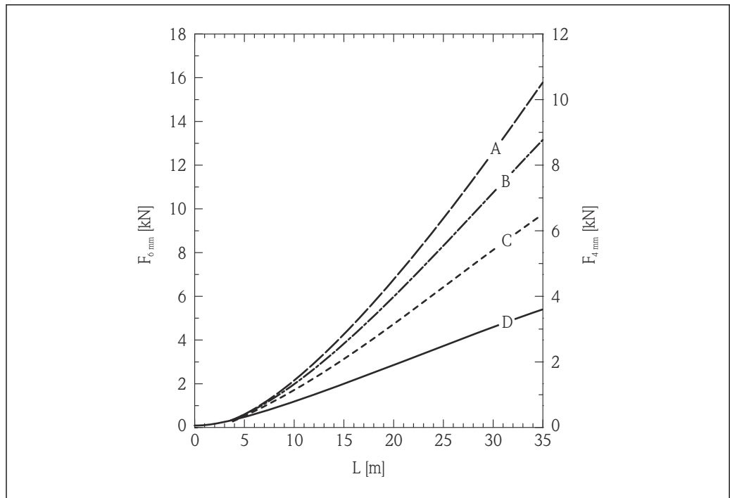
图 5 张力负载与物位 (L) 关系曲线图; 6 mm (0.24 in) 和 4 mm (0.16 in) 缆式探头, 聚乙烯颗粒料仓; 光滑金属仓壁
