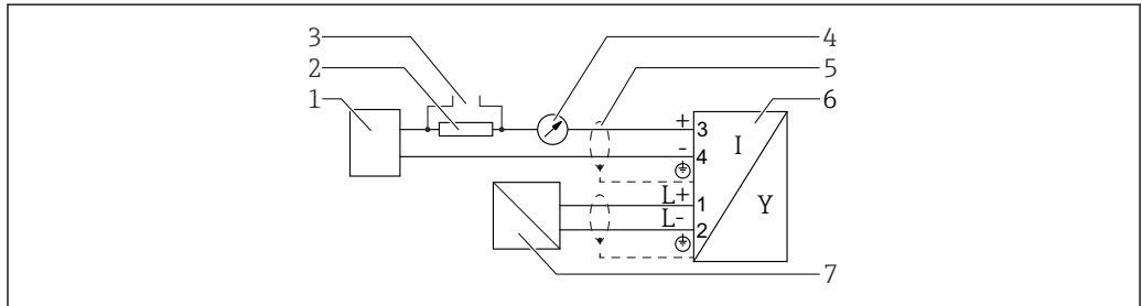
图 22 功能框图, 四线制: 4 ... 20 mA HART (10.4 ... 48 V DC )
