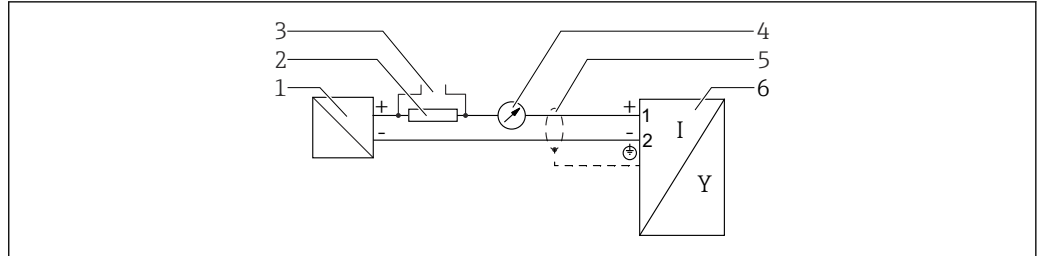
图 14 功能框图：4 ... 20 mA HART
