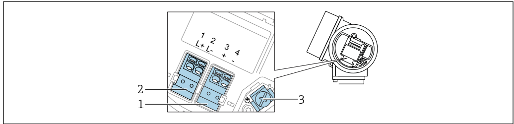
图 21 接线端子分配, 四线制: 4 ... 20 mA HART (10.4 ... 48 V DC )
