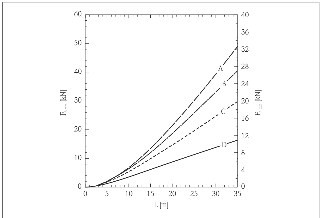
图 7 张力负载与物位 (L) 关系曲线图; 6 mm (0.24 in)和 4 mm (0.16 in)缆式探头, 水泥料仓; 光滑金属仓壁
