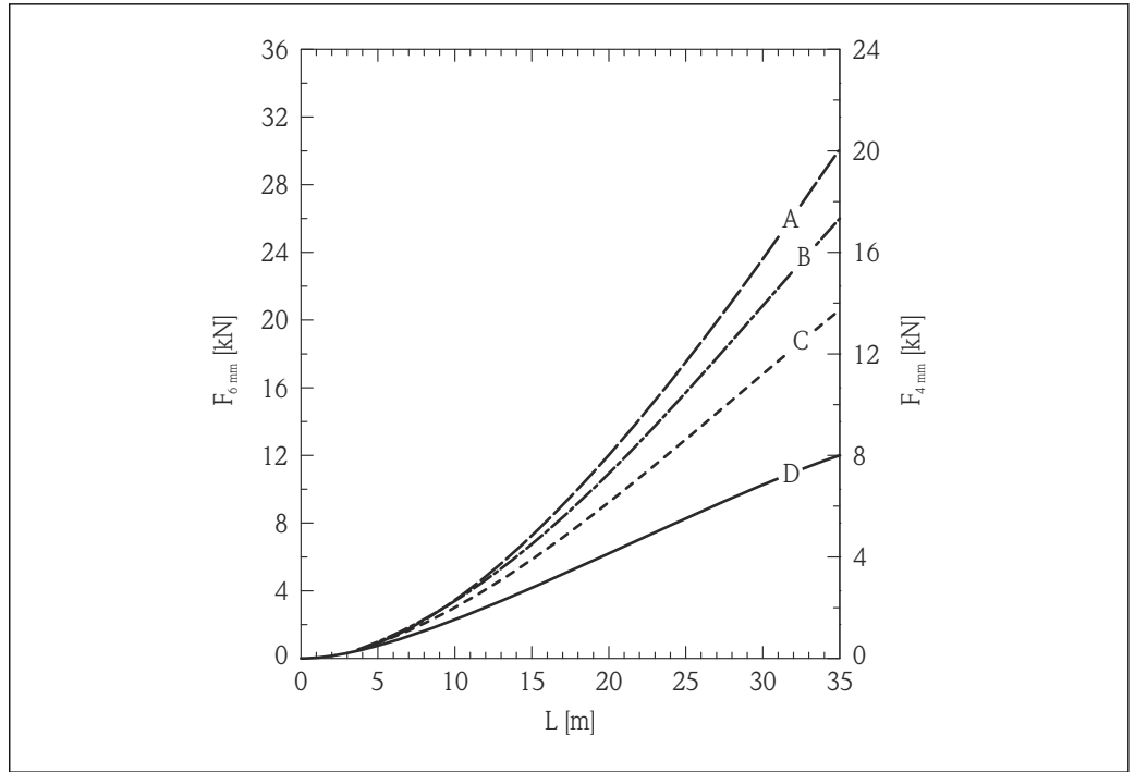
图 6 张力负载与物位 (L) 关系曲线图; 6 mm (0.24 in)和 4 mm (0.16 in)缆式探头, 小麦料仓; 光滑金属仓壁
