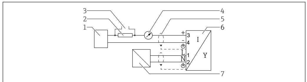
图 24 功能框图，四线制：4 ... 20 mA HART (90 ... 253 V AC )
