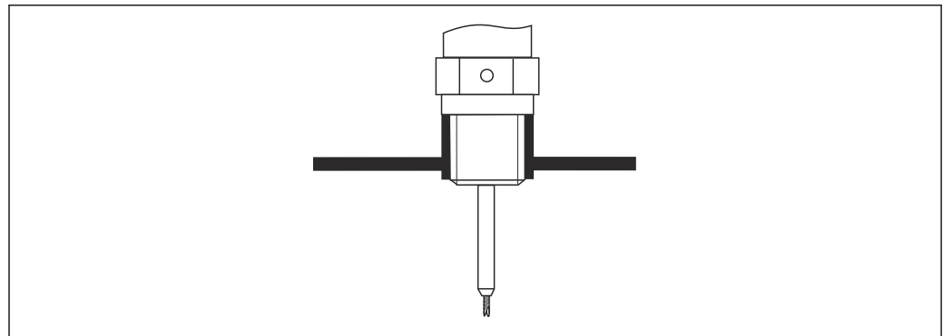
8 安装带螺纹连接的仪表；与罐顶齐平安装
