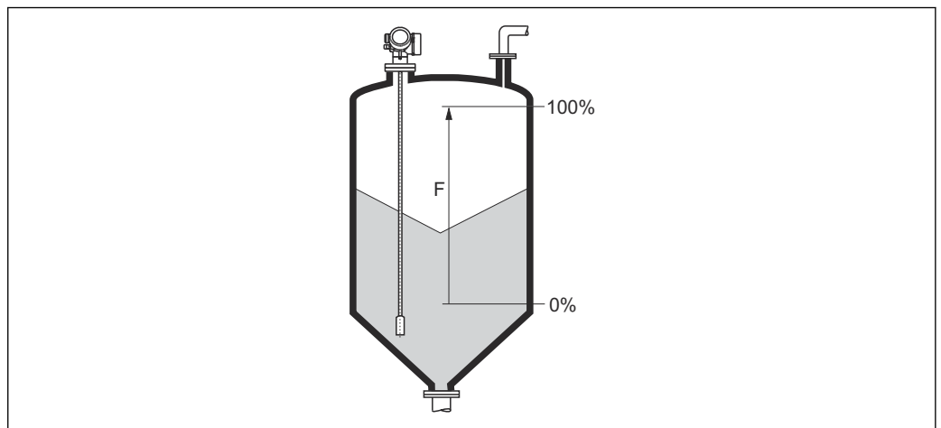
49 料位测量时的满标 (F)
