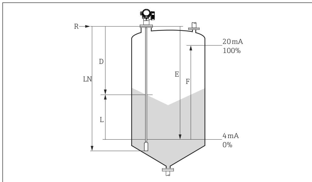
图 38 固体散料料位测量的设置参数
