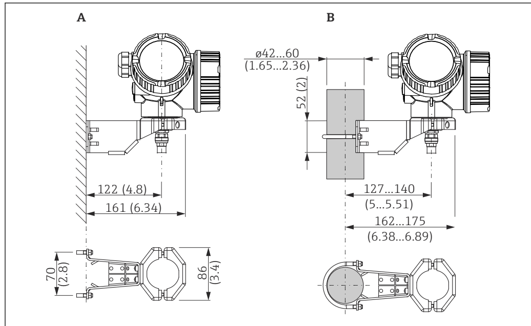
▣ 29 Suporte de montagem para invólucro dos componentes eletrônicos; unidade: mm (pol.)
