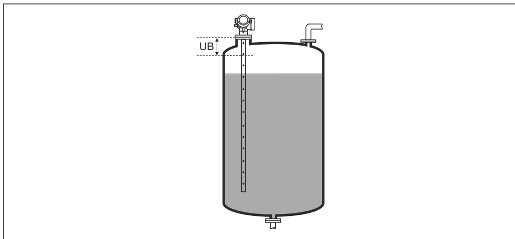
36 Distância de bloqueio (UB) para medições em líquidos
