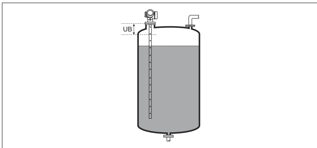
39 Distância de bloqueio (UB) para medições em líquidos
