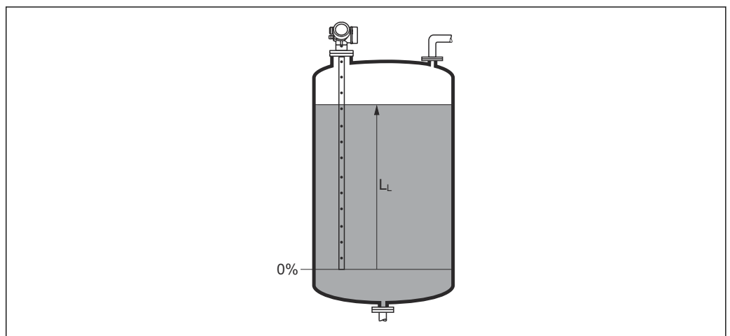
34 Nível em caso de medições de líquidos
