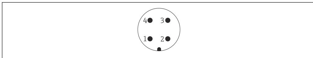
11 Affectation des broches du connecteur M12
