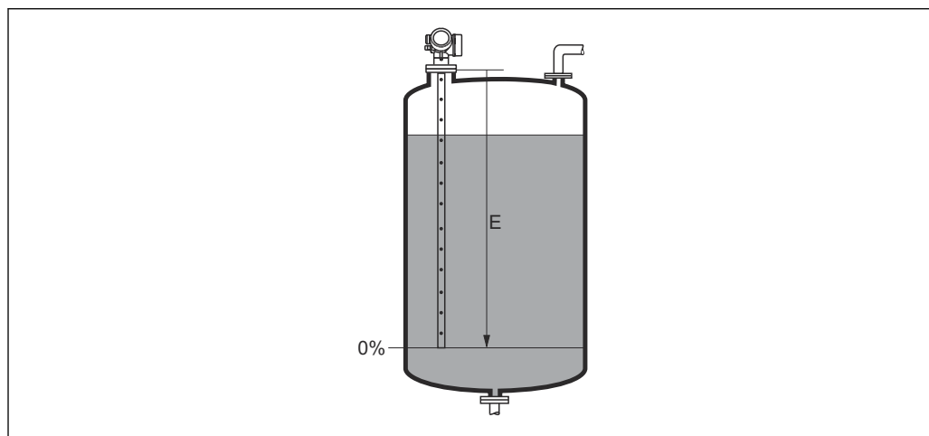
🔗 32 Distance du point zéro (E) pour la mesure sur liquides
