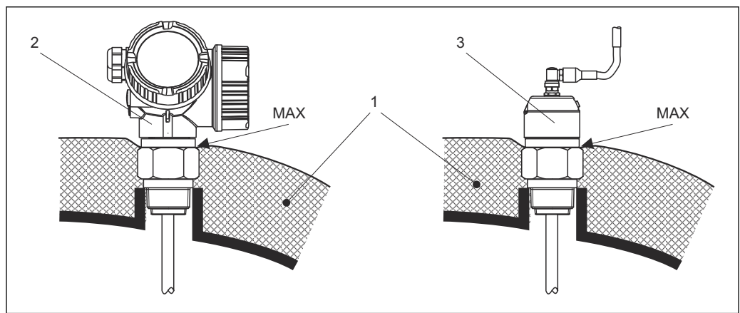
5 Технологическое соединение с резьбой
