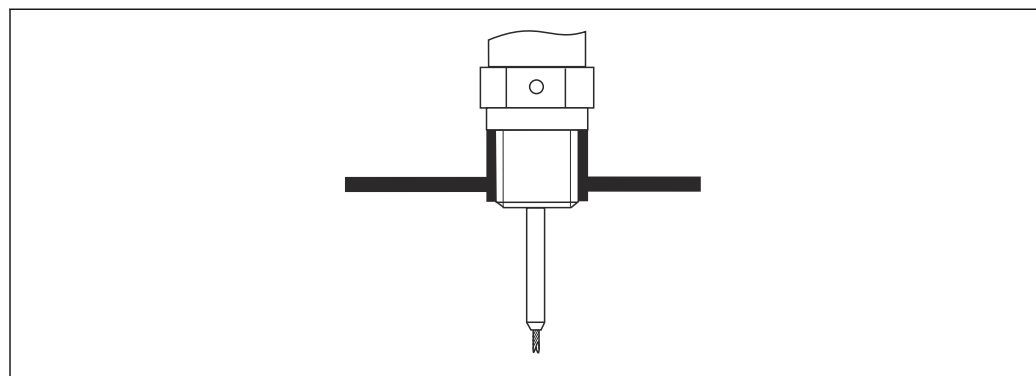
4 Монтаж с резьбовым соединением; вровень с крышей резервуара
