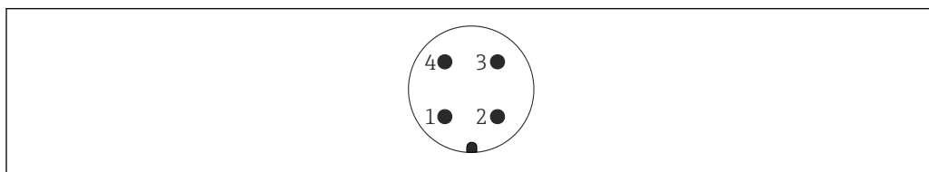
11 Назначение контактов разъема M12
