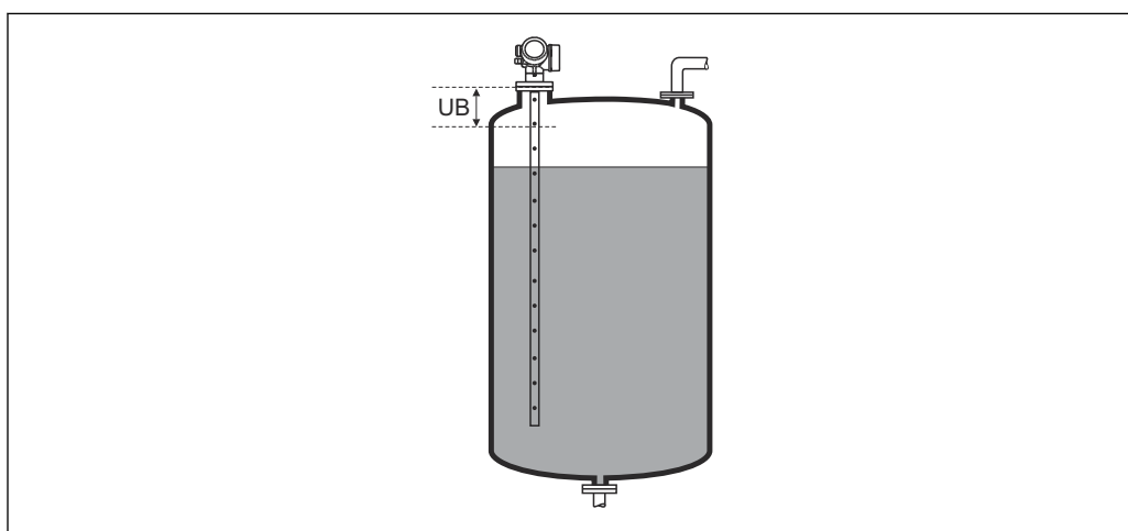
39 Блокирующая дистанция (UB) для измерения в жидких средах
