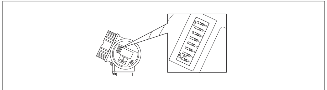
18 Переключатель адресов в клеммном отсеке
