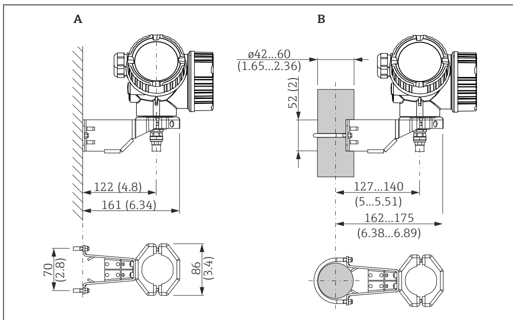
6 Монтаж корпуса блока электроники на монтажном кронштейне. Единица измерения мм (дюйм)
