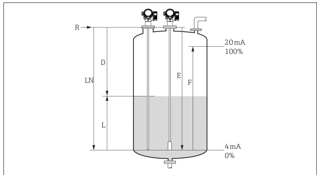
図 22 液体のレベル測定用パラメータの設定
