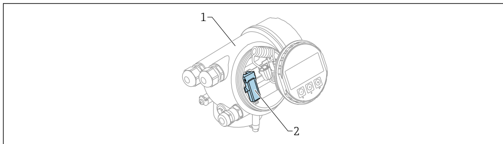
図 15 Bluetooth モジュール搭載の機器
