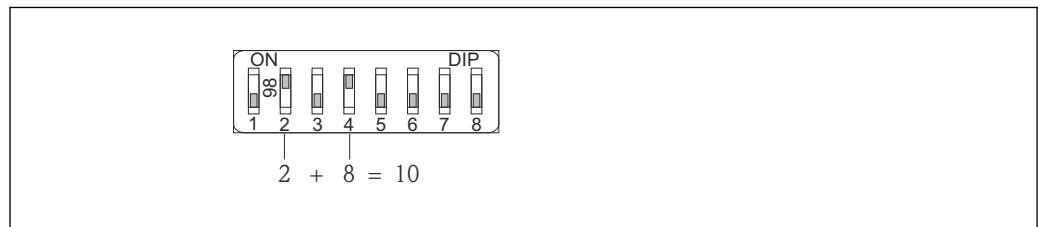
図 19 ハードウェアアドレス指定の例：スイッチ 8 を「オフ」位置にし、スイッチ 1～7 にアドレスを定義します。
