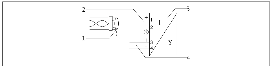
図 10 ブロック図：PROFIBUS PA / FOUNDATION フィールドバス
