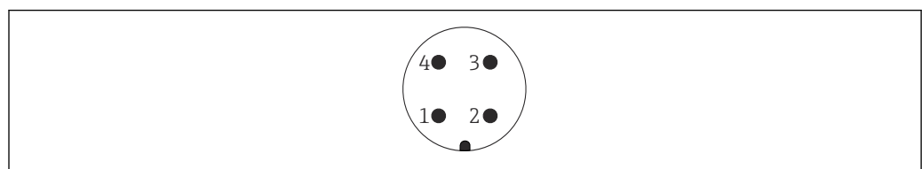
図 11 M12 プラグのピン割当て
