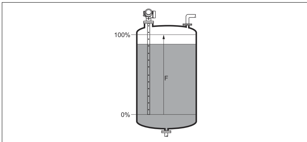
☐ 33 液体レベル測定用の満量校正 (F)
