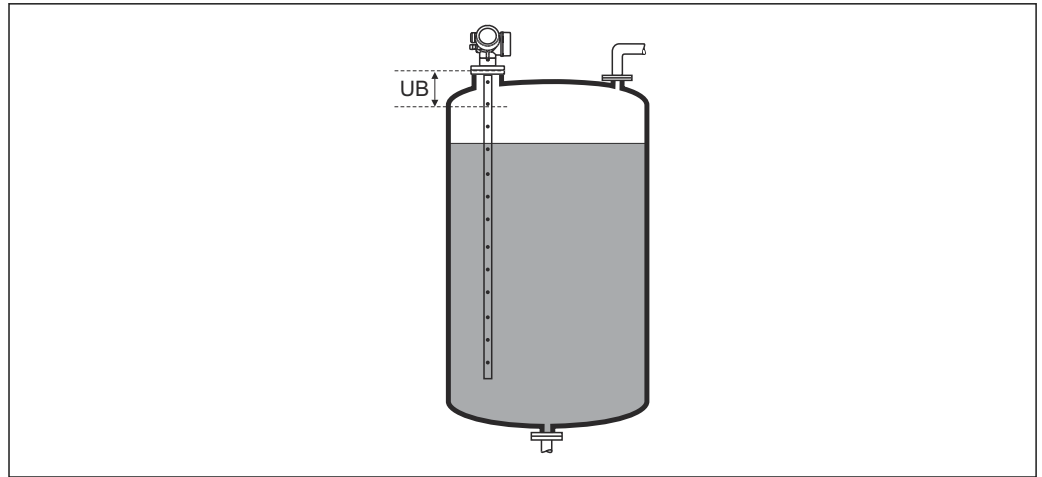
39 液位测量的盲区距离 (UB)
