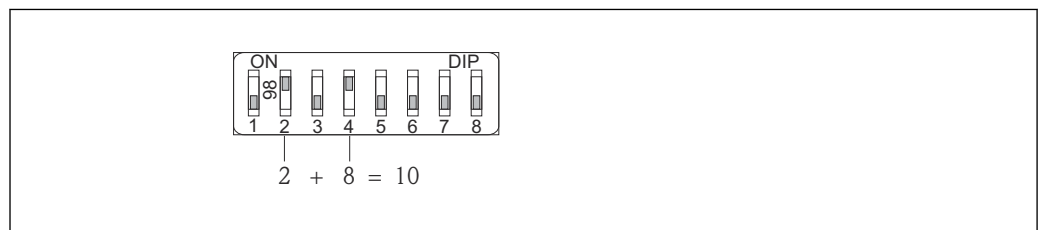
图 19 硬件地址设定示意图；开关 8 拨至“OFF”位置；使用开关 1...7 设置地址。
