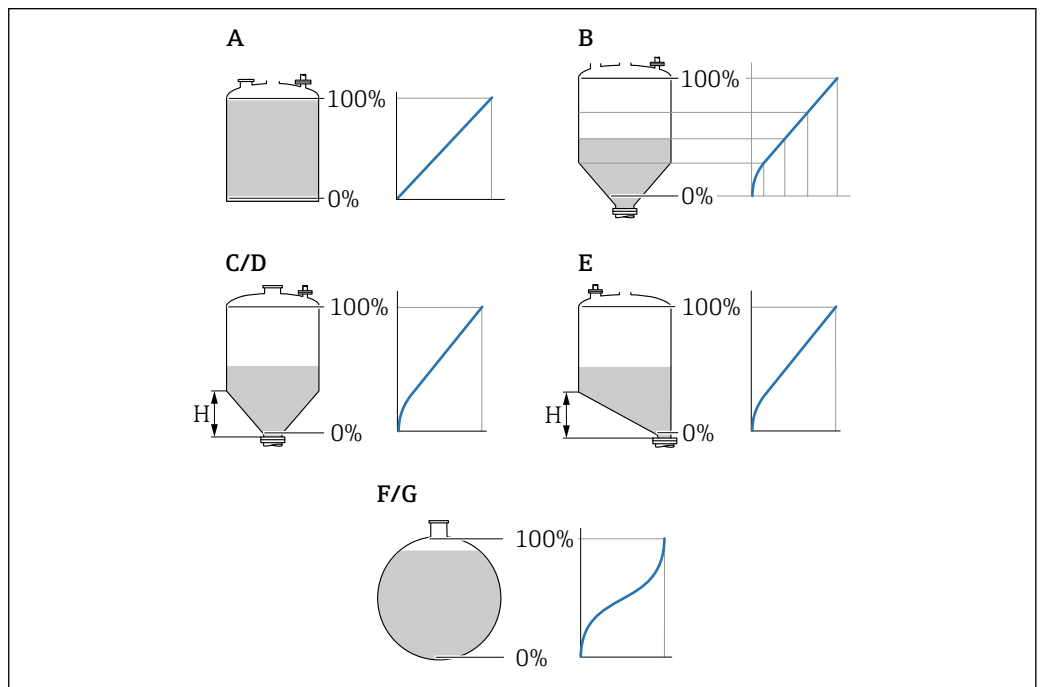
38 线性化类型
