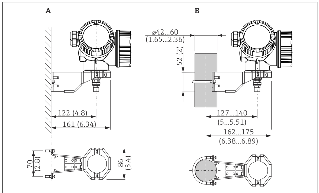
图 29 电子腔外壳安装架; 单位: mm (in)
