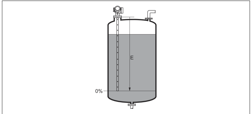
☑ 32 液位测量时的空标 (E)
