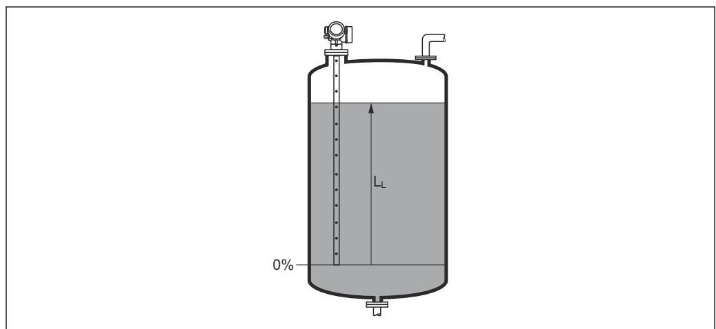
图 34 液位测量时的液位
