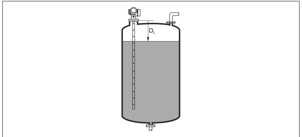
图 35 液位测量时的距离
