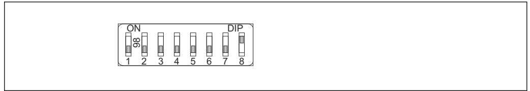
图 20 软件地址设定示意图；开关 8 拨至“ON”位置；进入操作菜单设置地址（Setup → Device address）。
