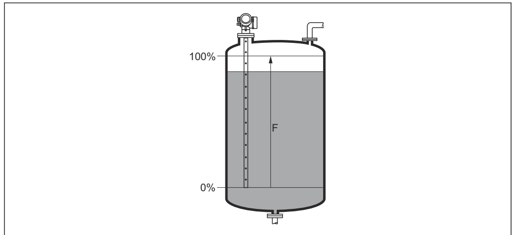
图 33 液位测量时的满标 (F)
