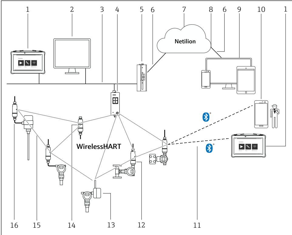
1 Architecture système de la version SWA50 WirelessHART
