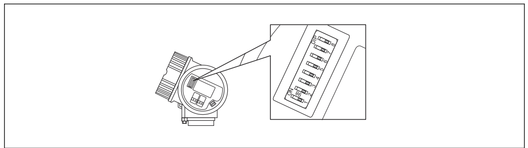
图 22 接线腔中的地址设定开关
