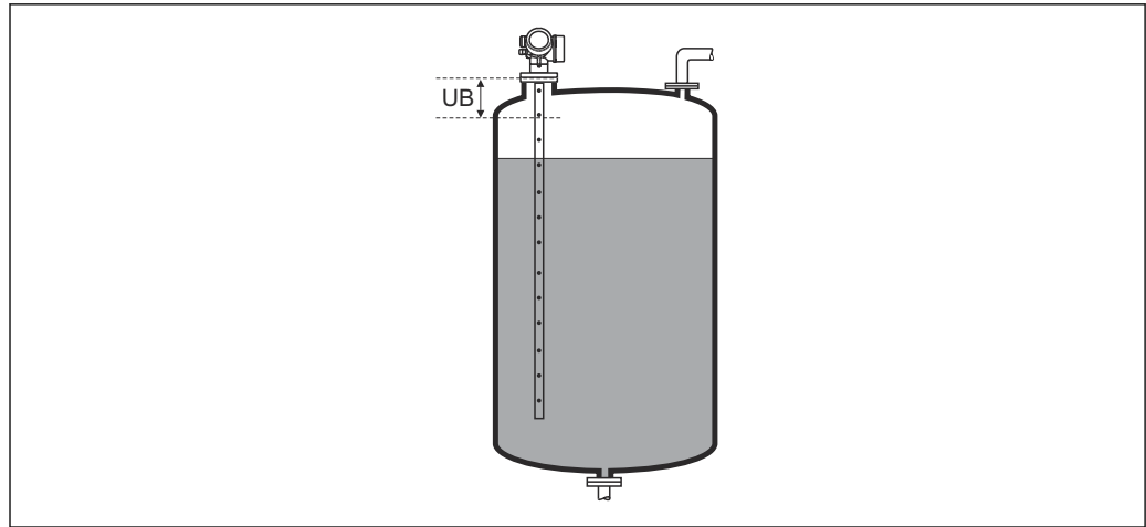
图 46 液位测量的盲区距离 (UB)
