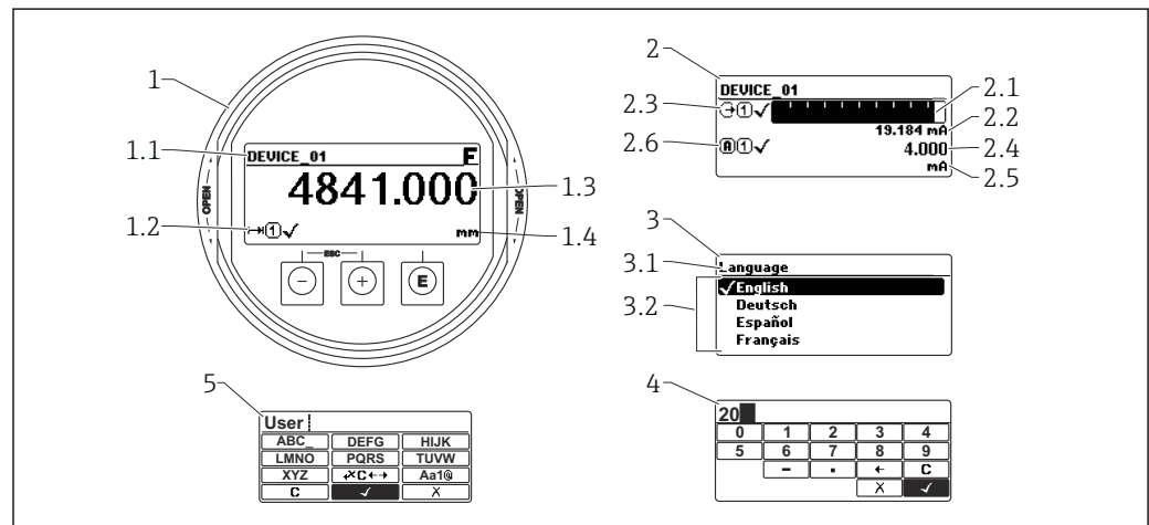
图 21 显示与操作单元的显示格式
