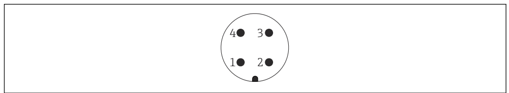
图 15 M12 插头的针脚分配
