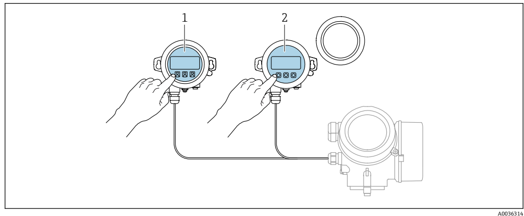
图 18 FHX50 的操作选项
