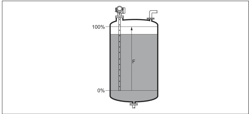
图 40 液位测量时的满标 (F)
