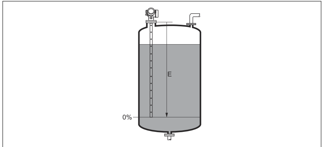
38 液位测量时空标 (E)
