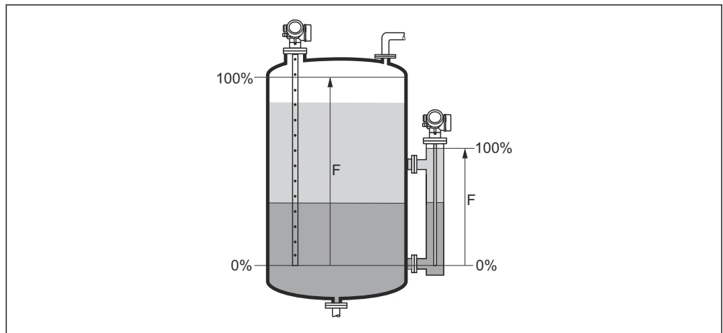
图 41 界面测量时的满标 (F)
