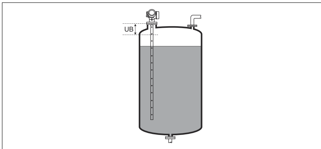
图 49 液位测量的盲区距离 (UB)
