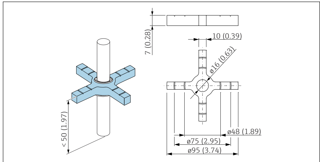
图 37 尺寸参数; \phi 48 \dots 95 \text{ mm} (1.89 ... 3.74 in) 对中环, PEEK
