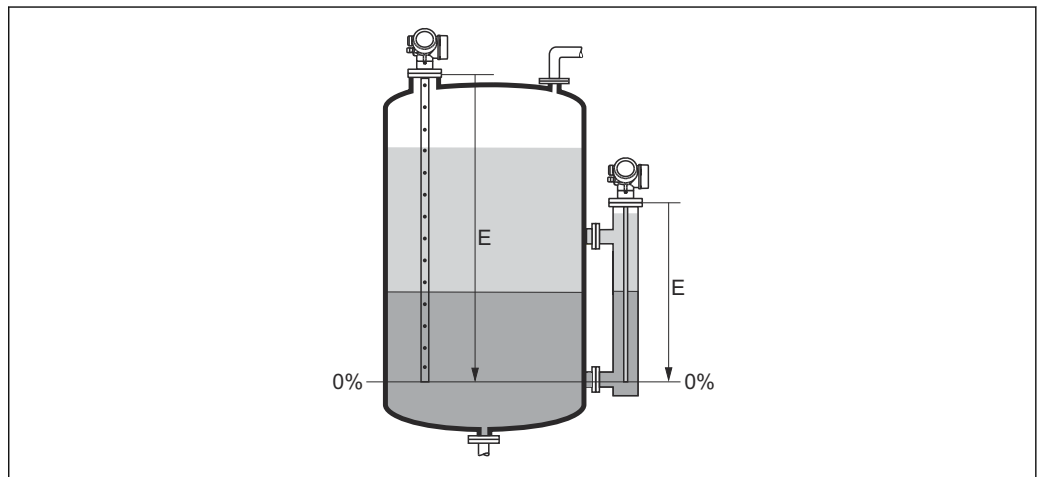
39 界面测量时空标 (E)
