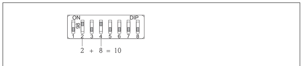
图 23 硬件地址设定示意图；开关 8 拨至“OFF”位置；使用开关 1...7 设置地址。
