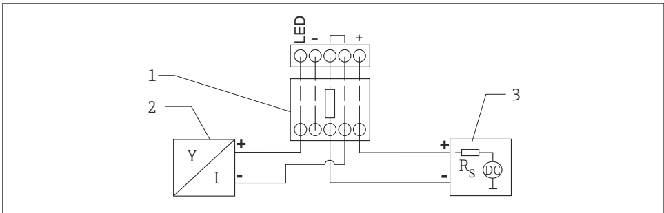
10 Diagrama de funciones del equipo HART, RIA15 con luz, módulo de resistencia para comunicaciones HART
