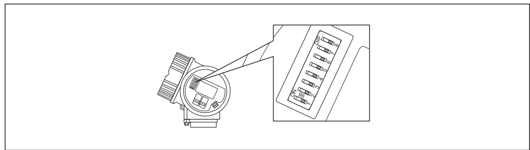
図 22 端子部のアドレススイッチ
