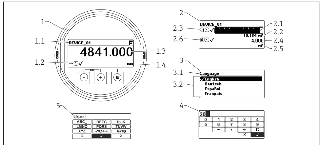
図 21 表示モジュールおよび操作モジュールの表示形式
