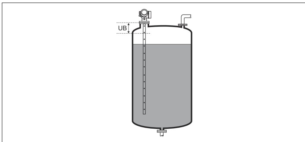
49 液体計測の不感知距離 (UB)
