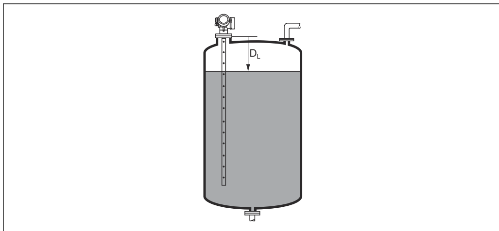
図 44 液体計測の距離
