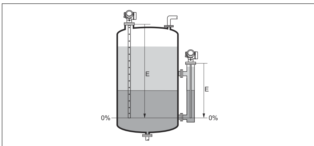
39 界面測定用の空校正 (E)
