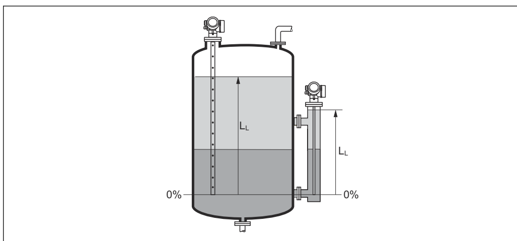
図 43 界面測定時のレベル
