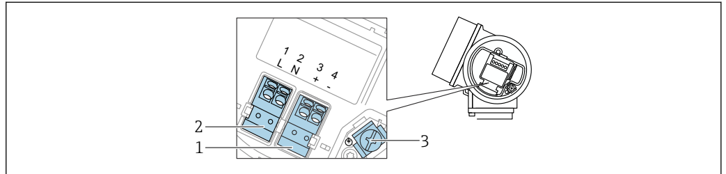
図 12 端子の割当て、4線式：4～20 mA HART (90～253 V AC )
