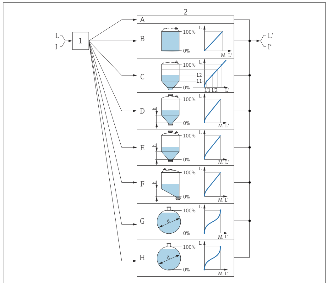
☐ 47 リニアライゼーション：レベルから、および（該当する場合は）界面から体積または質量に変換。変換は容器の形状に依存
