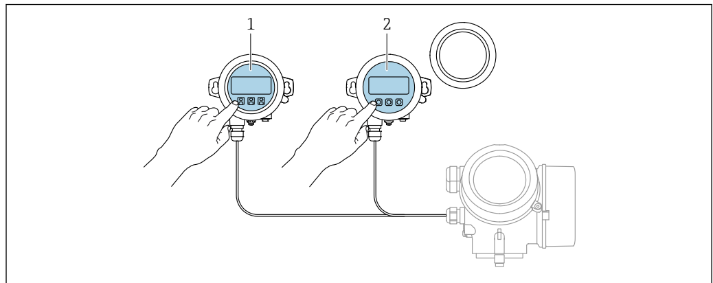
■ 18 FHX50 操作オプション
