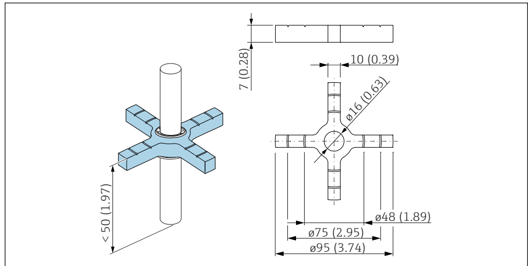
図 37 寸法 ; センタリングスター PEEK、 \varnothing 48 \sim 95 mm (1.89~3.74 in)
