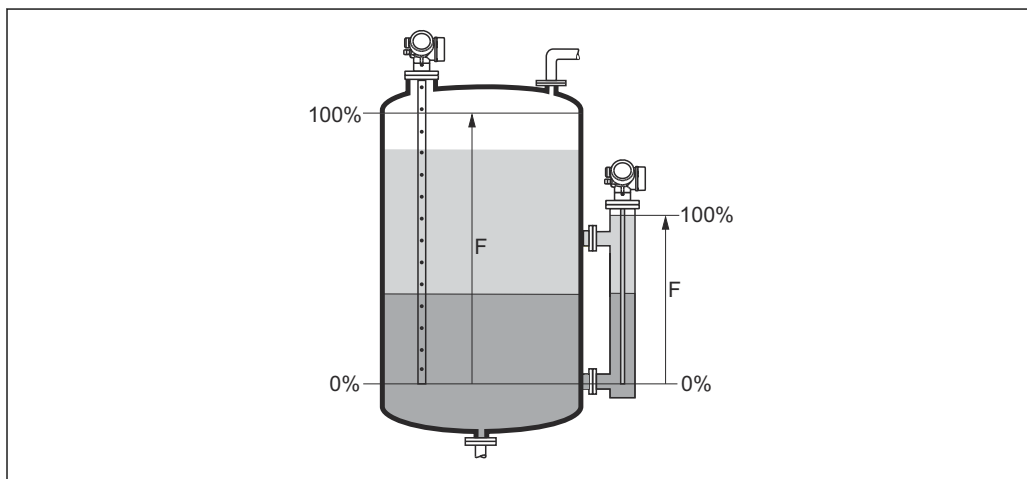
図 41 界面測定用の満量校正 (F)
