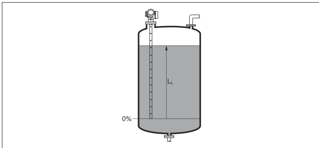
図 42 液体計測時のレベル
