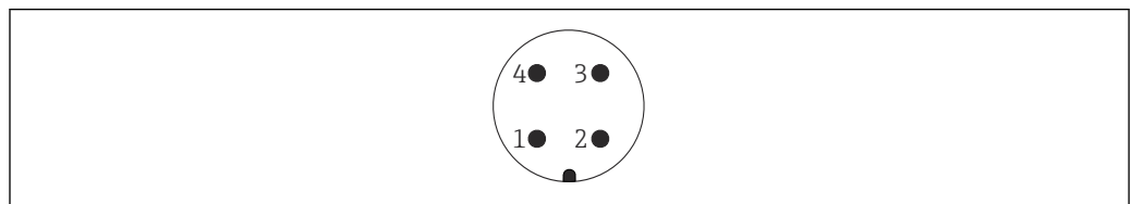
図 15 M12 プラグのピン割当て
