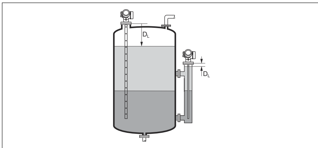
図 45 界面測定 of 距離
