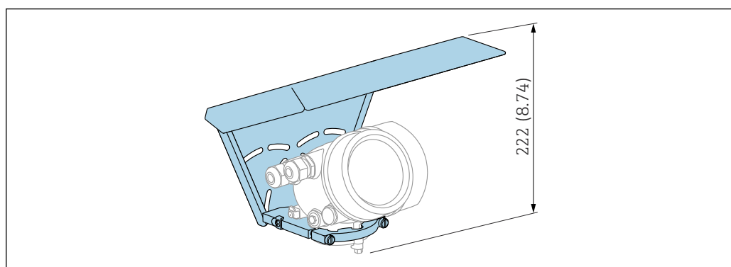
32 高さ。測定単位 mm (in)
