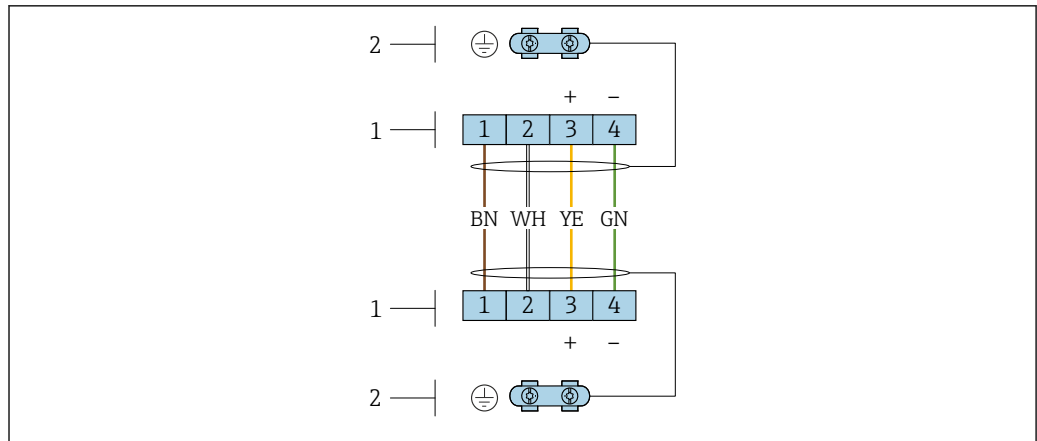
2 Bornes de raccordement pour le compartiment de raccordement dans le support mural du transmetteur et le boîtier de raccordement du capteur
