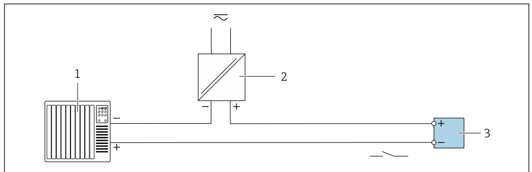
7 Exemple de raccordement pour la sortie tout ou rien (passive)
