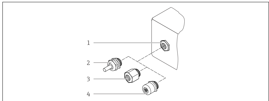
29 Entrées de câble/presse-étoupe possibles
