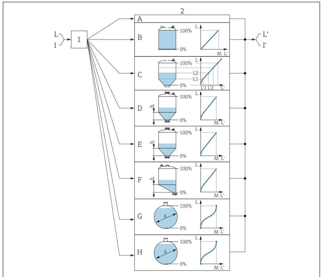
图 42 线性化：将物位和（相关）界面高度转换成体积或重量；转换取决于罐体形状
