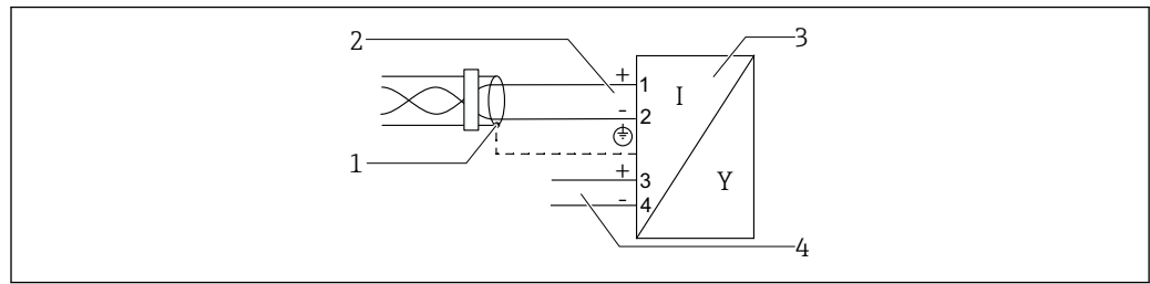
图 15 功能框图: PROFIBUS PA / FOUNDATION Fieldbus
