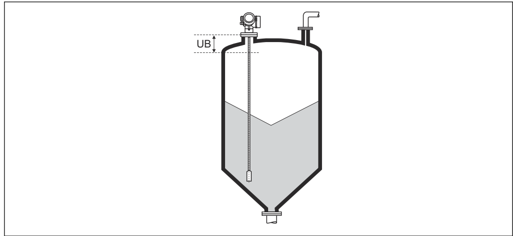
图 41 料位测量的盲区距离 (UB)
