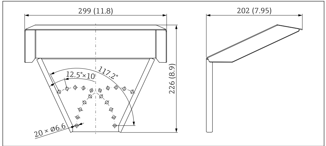
图 33 尺寸参数。测量单位 mm (in)
