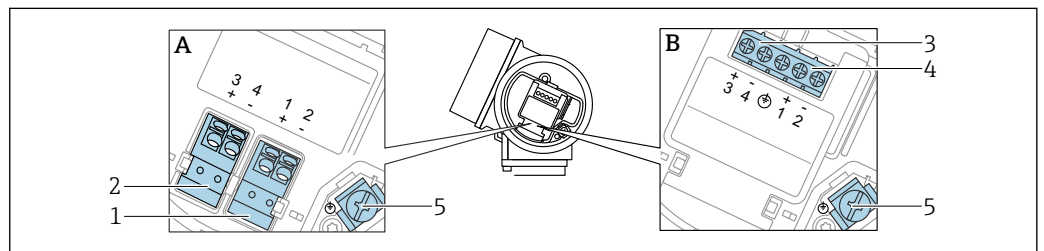
图 14 接线端子分配：PROFIBUS PA / FOUNDATION Fieldbus
