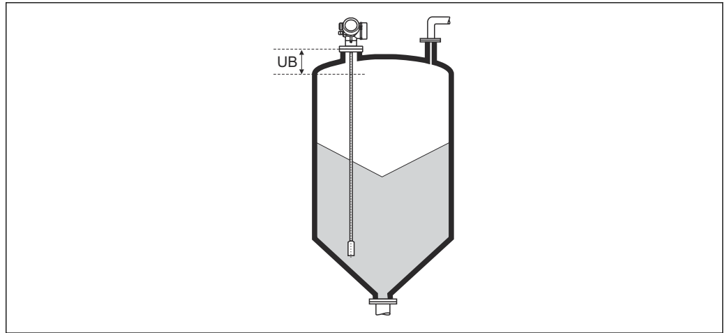
44 料位测量的盲区距离 (UB)
