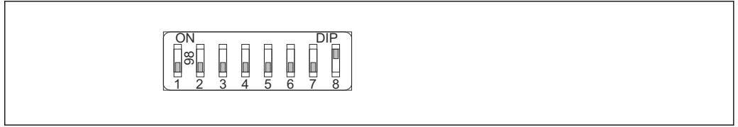
图 25 软件地址设定示意图；开关 8 拨至“ON”位置；进入操作菜单设置地址（Setup → Device address）。
