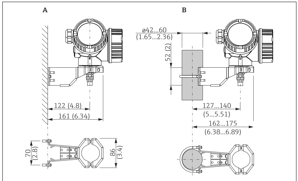
图 34 电子腔外壳安装架; 单位: mm (in)
