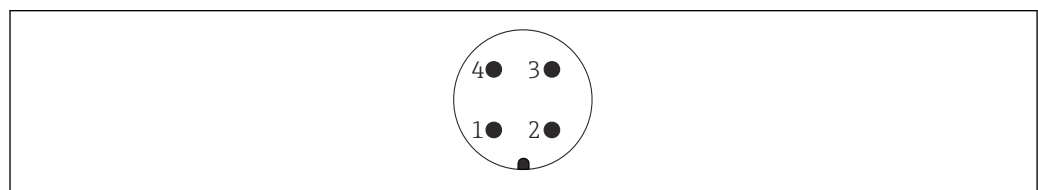
图 16 M12 插头的针脚分配
