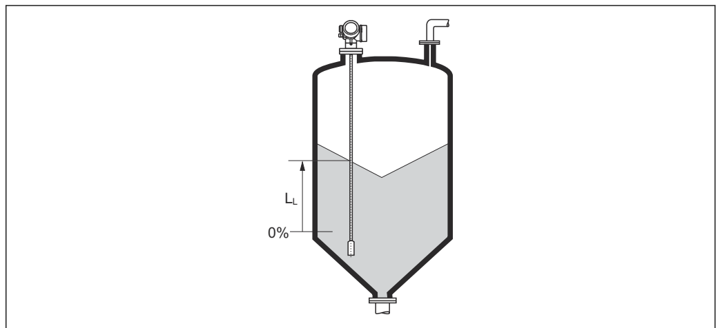
39 料位测量时的料位
