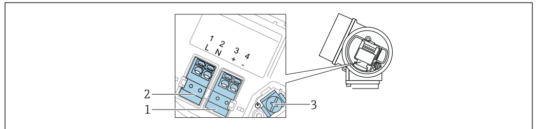
图 13 接线端子分配，四线制：4 ... 20 mA HART (90 ... 253 V AC )
