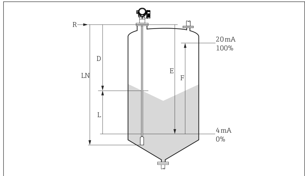
图 27 固体散料料位测量的设置参数
