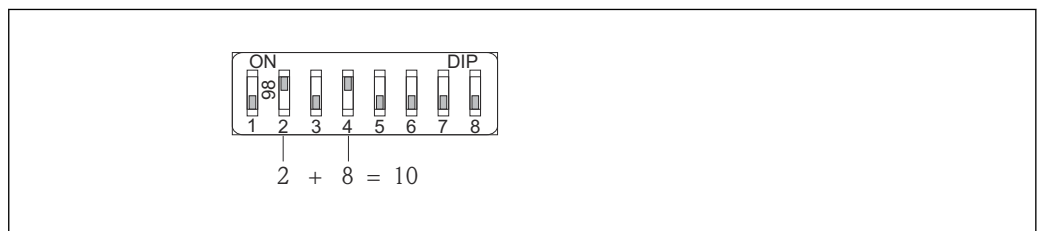
24 Esempio di indirizzamento hardware: il microinterruttore 8 è in posizione "OFF"; i microinterruttori 1...7 definiscono l'indirizzo.
