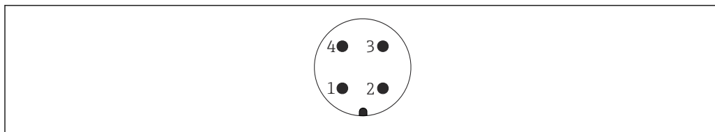
16 Assegnazione dei pin del connettore M12
