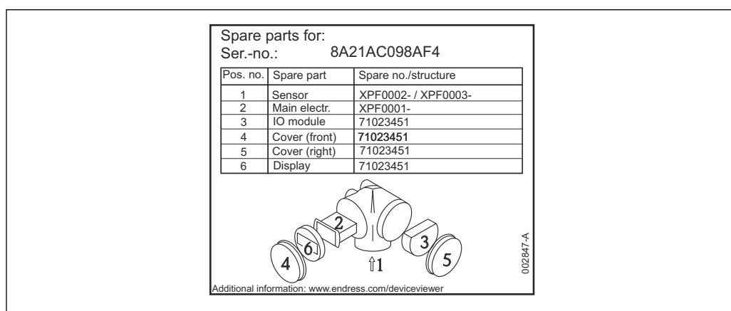
▣ 30 Пример заводской таблички с перечнем запасных частей, размещаемой на крышке присоединительного отсека
