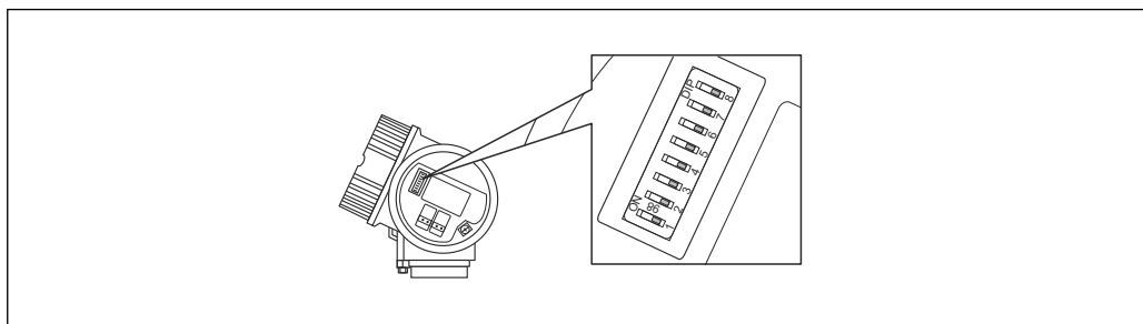
23 Переключатель адресов в клеммном отсеке
