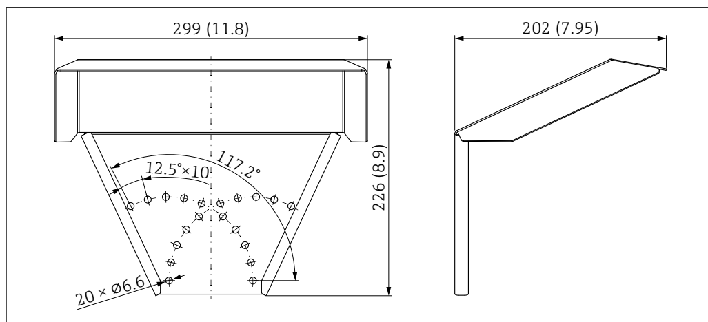
■ 33 Размеры. Единица измерения мм (дюйм)
