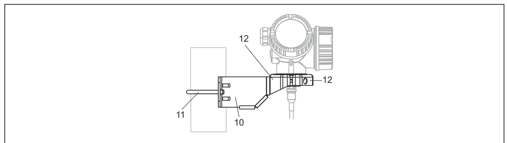
35 Материал; монтажный кронштейн
