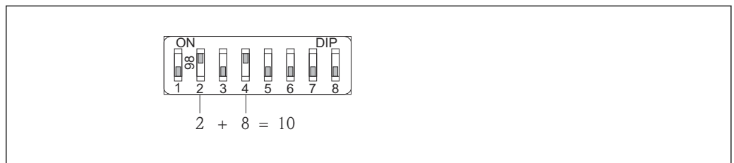
☞ 17 Exemple pour l'adressage hardware ; le commutateur 8 est en position "OFF" ; les commutateurs 1 à 7 définissent l'adresse.
