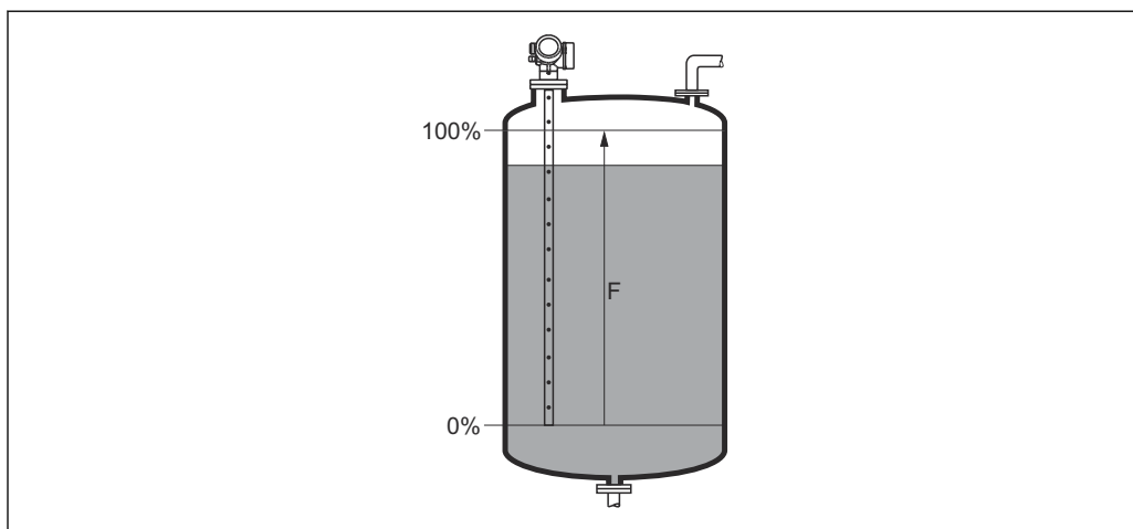
31 Plage de mesure (F) pour la mesure sur liquides
