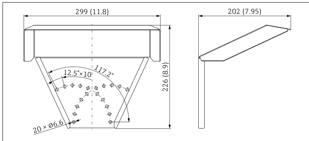
■ 26 Dimensions. Unité de mesure mm (in)
