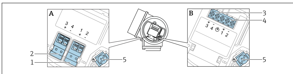
7 Назначение клемм; PROFIBUS PA/FOUNDATION Fieldbus
