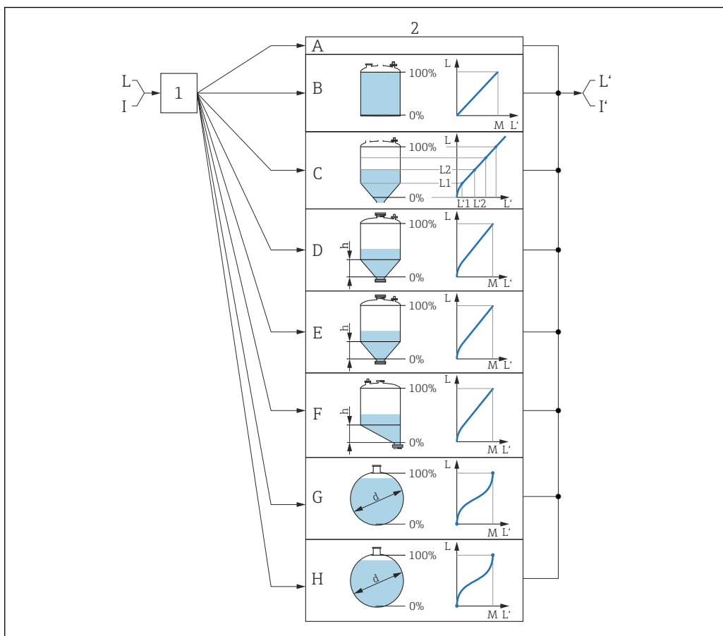
35 Линеаризация: преобразование уровня и, если применимо, границы раздела фаз в объем или массу; преобразование зависит от формы резервуара
