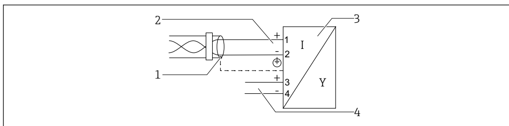
8 Блок-схема: PROFIBUS PA/FOUNDATION Fieldbus
