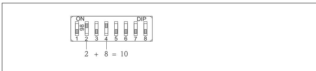
17 Пример аппаратной адресации: переключатель 8 переведен в положение OFF; переключатели 1–7 определяют адрес.
