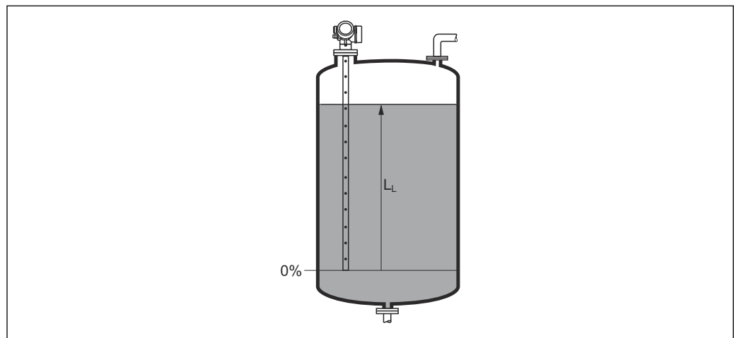
32 Nivel en caso de mediciones de líquido
