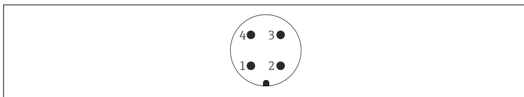
9 Asignación de pins del conector M12
