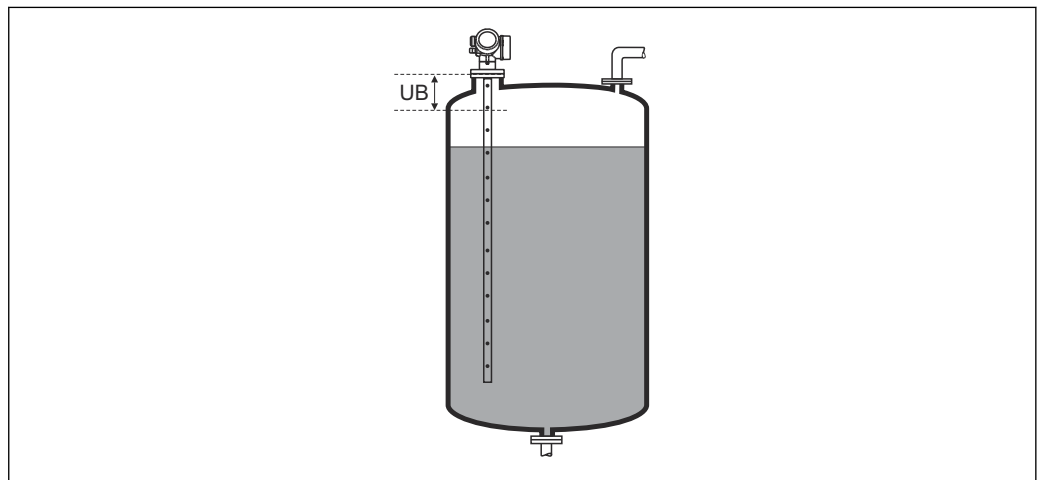
37 Distancia de bloqueo (UB) para mediciones de líquidos
