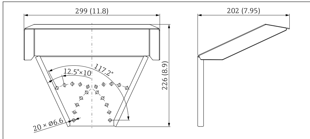
图 26 尺寸参数。测量单位 mm (in)
