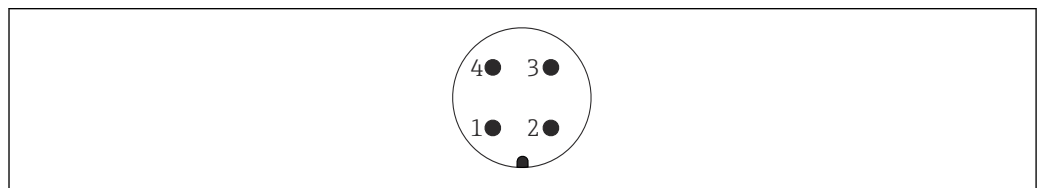
图 9 M12 插头的针脚分配
