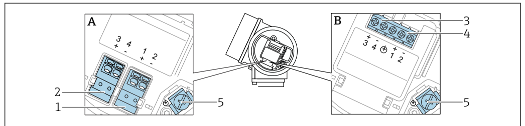
图 7 接线端子分配：PROFIBUS PA / FOUNDATION Fieldbus
