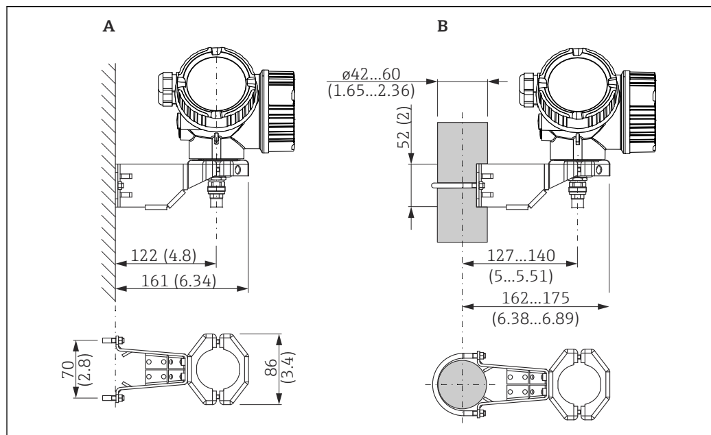
图 27 电子腔外壳安装架; 单位: mm (in)
