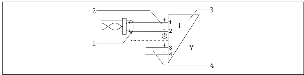
图 8 功能框图: PROFIBUS PA / FOUNDATION Fieldbus
