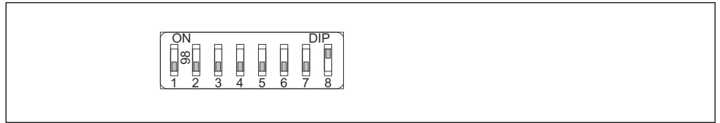
图 18 软件地址设定示意图；开关 8 拨至“ON”位置；进入操作菜单设置地址（Setup → Device address）。
