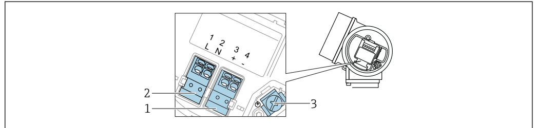
图 6 接线端子分配，四线制：4 ... 20 mA HART (90 ... 253 V AC )
