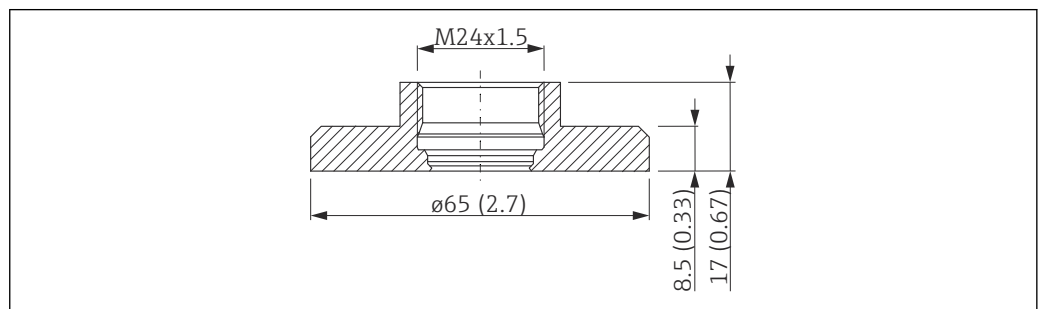
33 Размеры; приварной переходник
