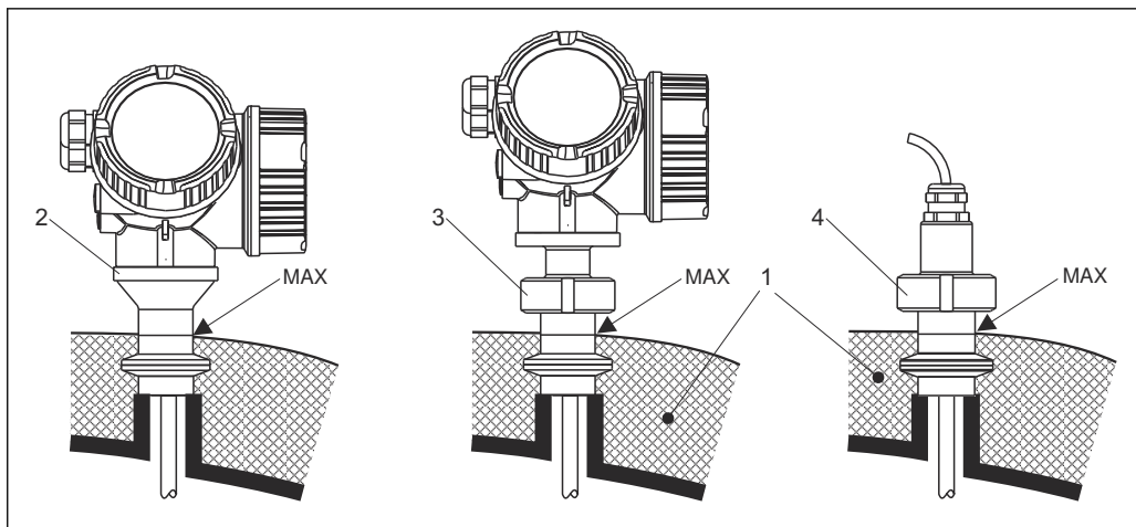
4 Гигиенические технологические соединения
