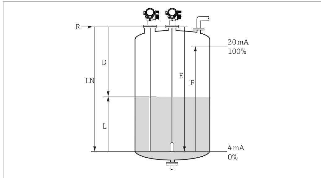
20 Параметры конфигурации для измерения уровня жидкости
