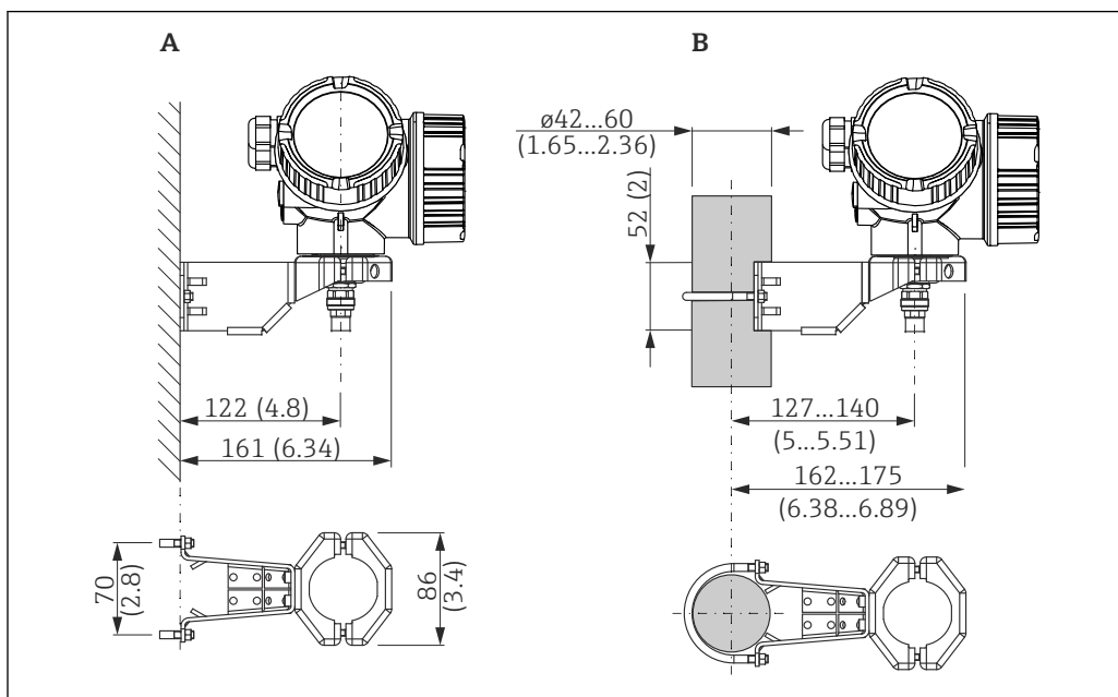
5 Монтаж корпуса блока электроники на монтажном кронштейне. Единица измерения мм (дюйм)
