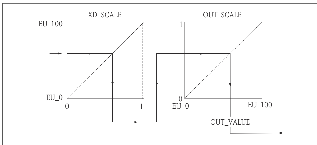
22 Масштабирование измеренного значения в блоке аналоговых входов
