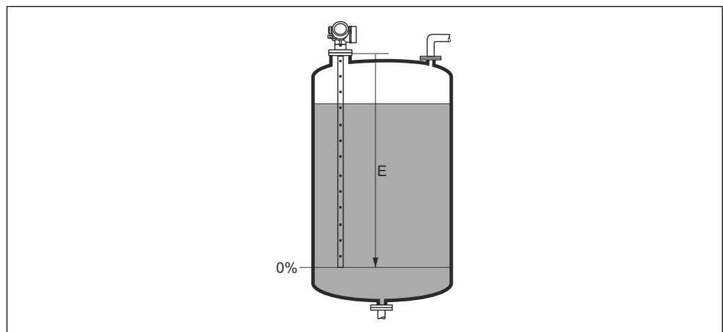
🔗 34 液位测量时的空标 (E)
