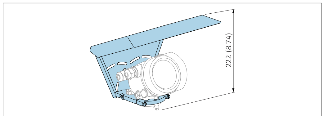
图 29 高度。测量单位 mm (in)
