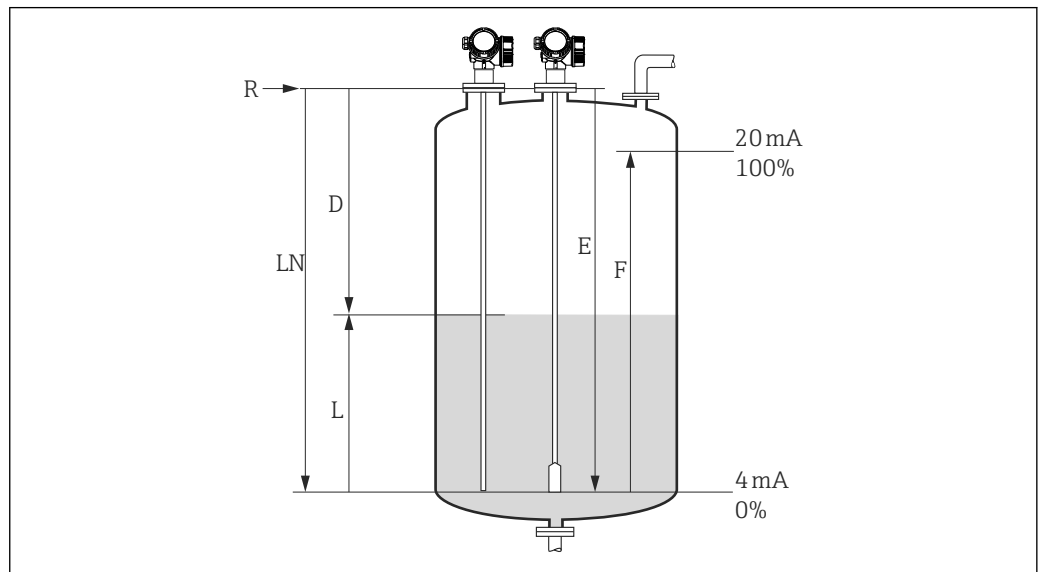
图 23 液位测量的设置参数
