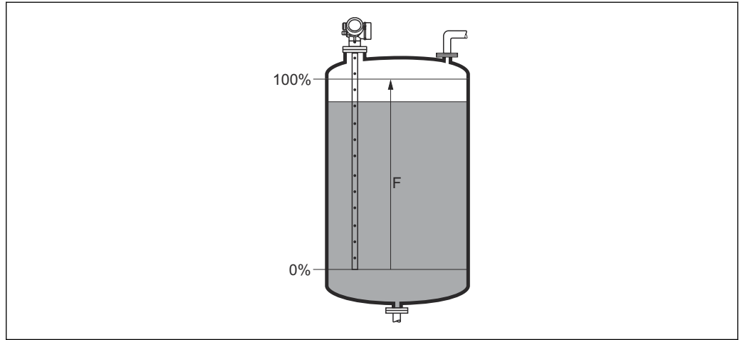
35 液位测量时的满标 (F)
