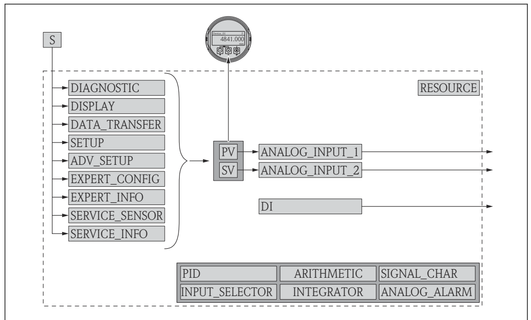
图 18 设备块的出厂设置
