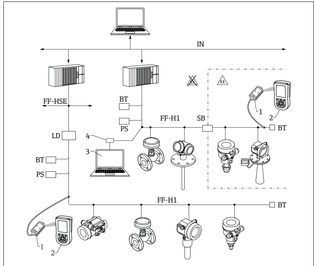
图 13 FOUNDATION Fieldbus 系统架构及组件
