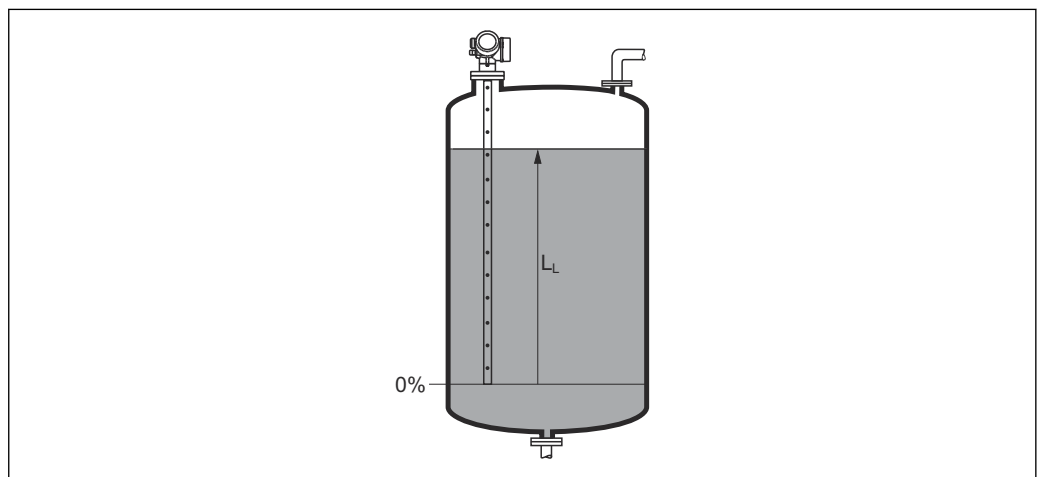
36 液位测量时的液位
