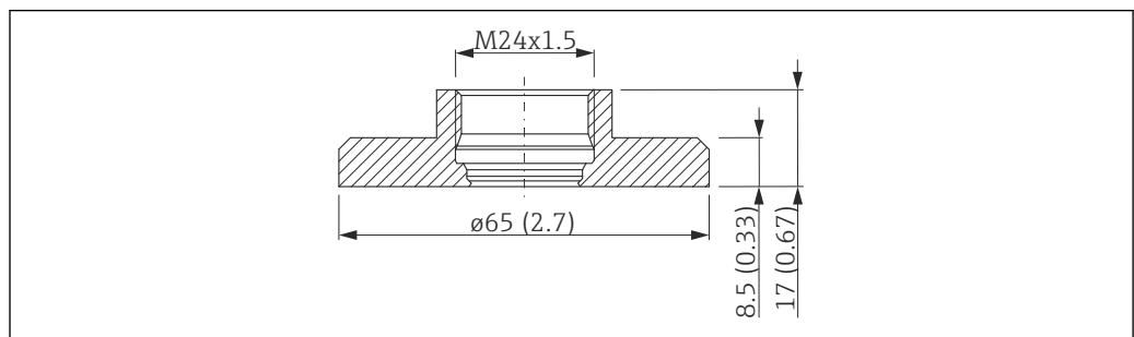
33 Dimensioni, adattatore a saldare
