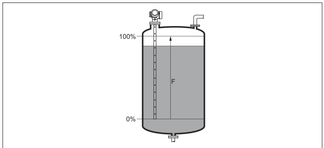
35 Calibrazione di pieno (F) per misure di livello nei liquidi
