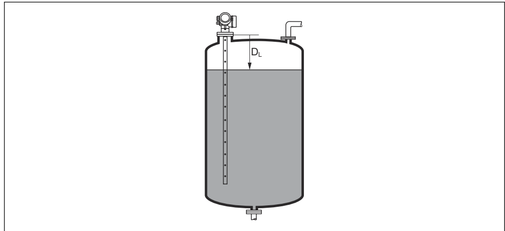
37 Distanza per misure di liquidi
