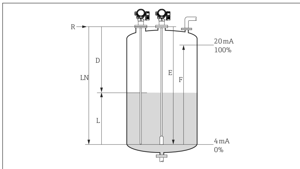
23 Parametri di configurazione per la misura di livello nei liquidi
