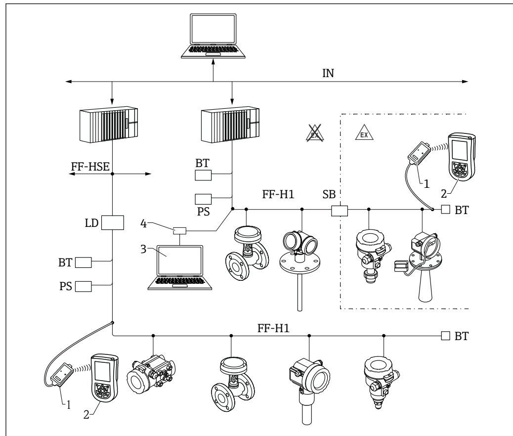
Fig. 13 Architettura del sistema FOUNDATION Fieldbus con componenti associati
