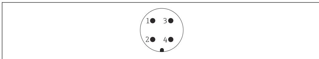
11 Affectation des broches du connecteur 7/8"
