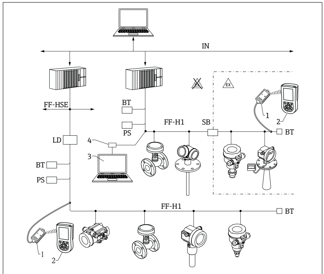
15 Architecture du système FOUNDATION Fieldbus avec composants associés
