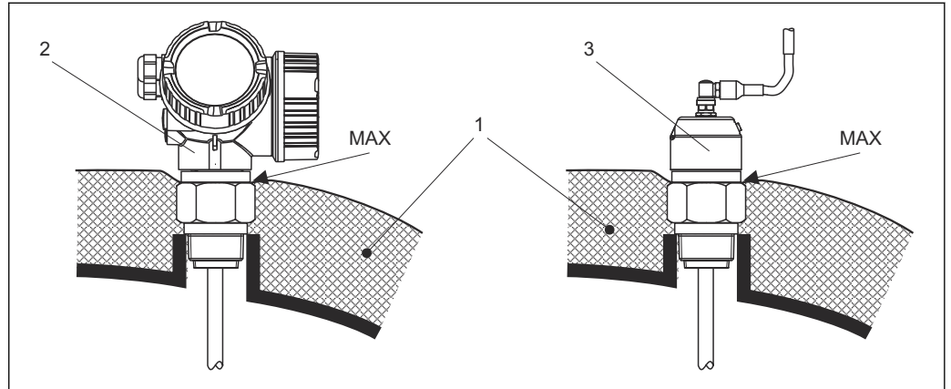
図 5 プロセス接続 (ネジ)
