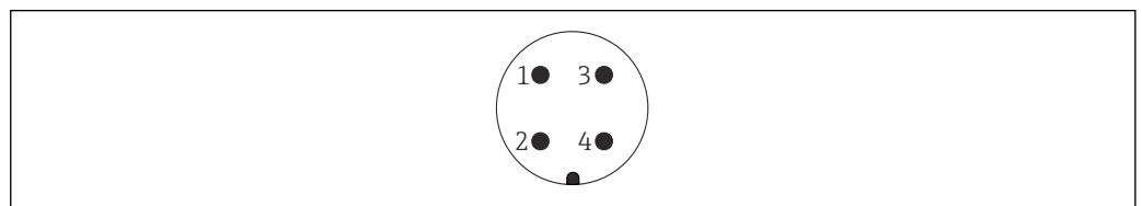
図 11 7/8" プラグのピン割当て
